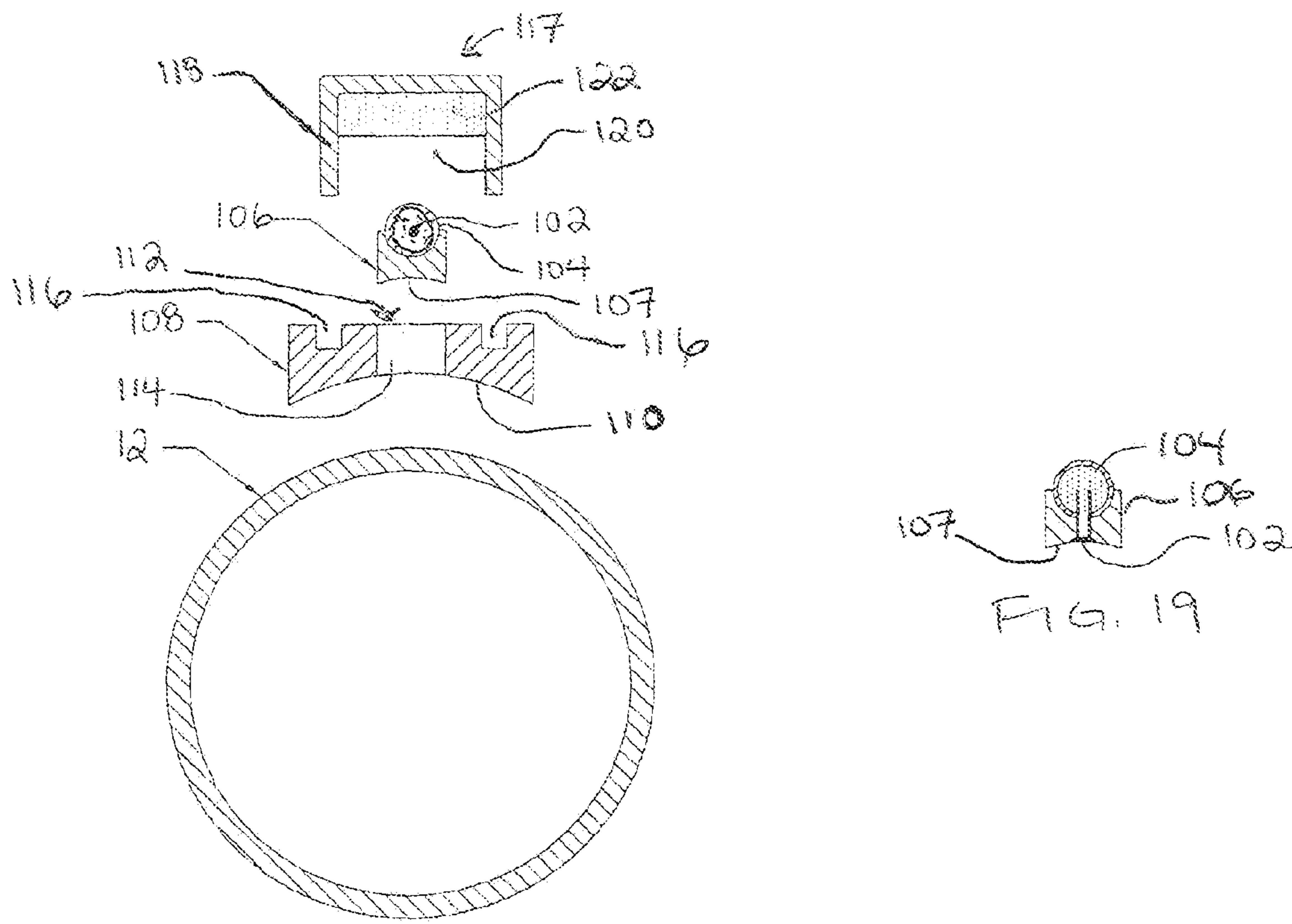
FIG. 18
