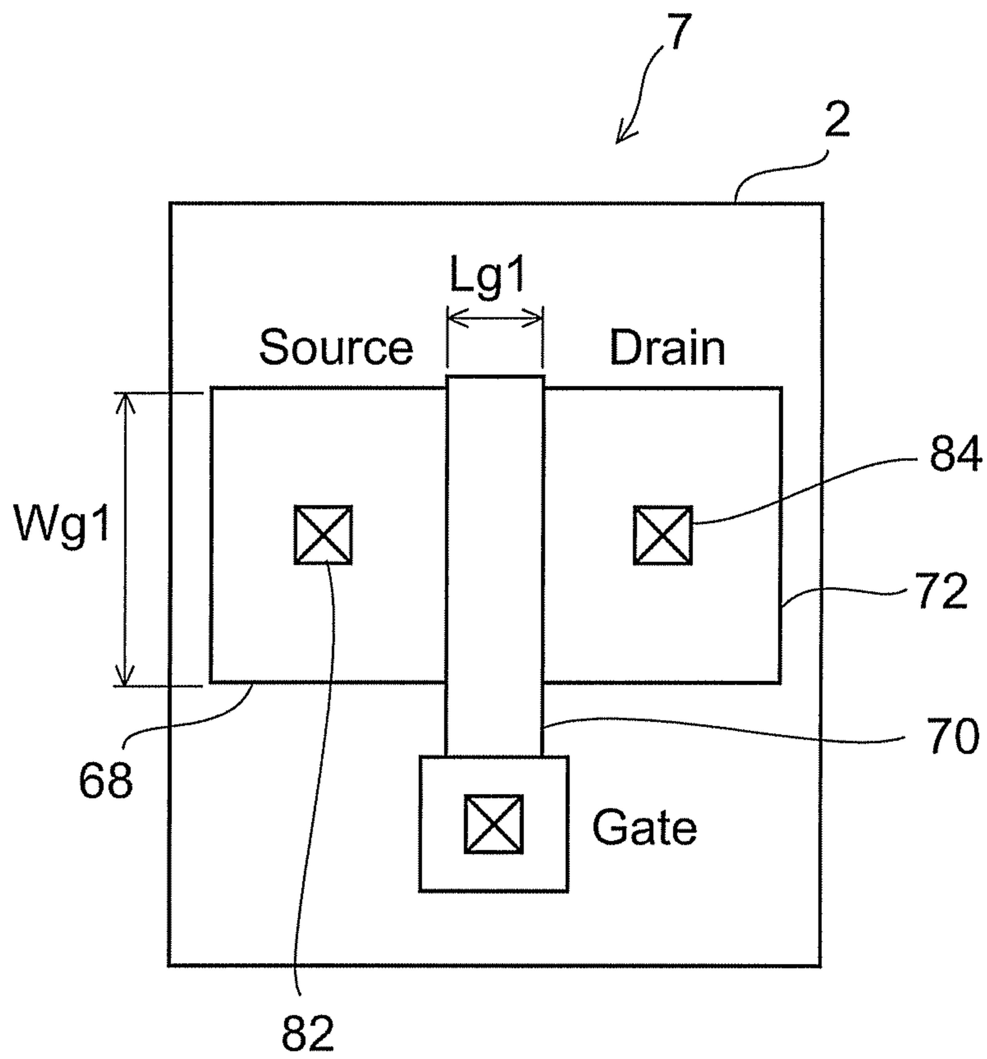
FIG. 5
