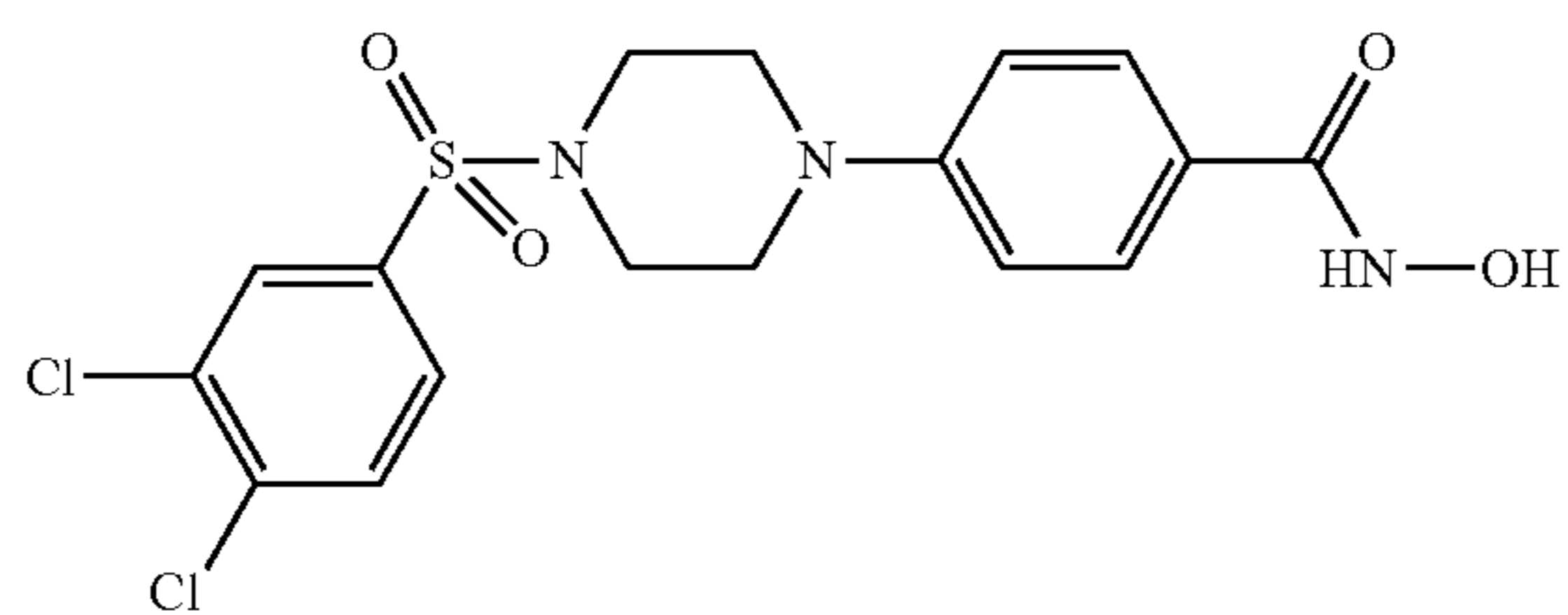
Co. No. 80; Ex. [B1]
