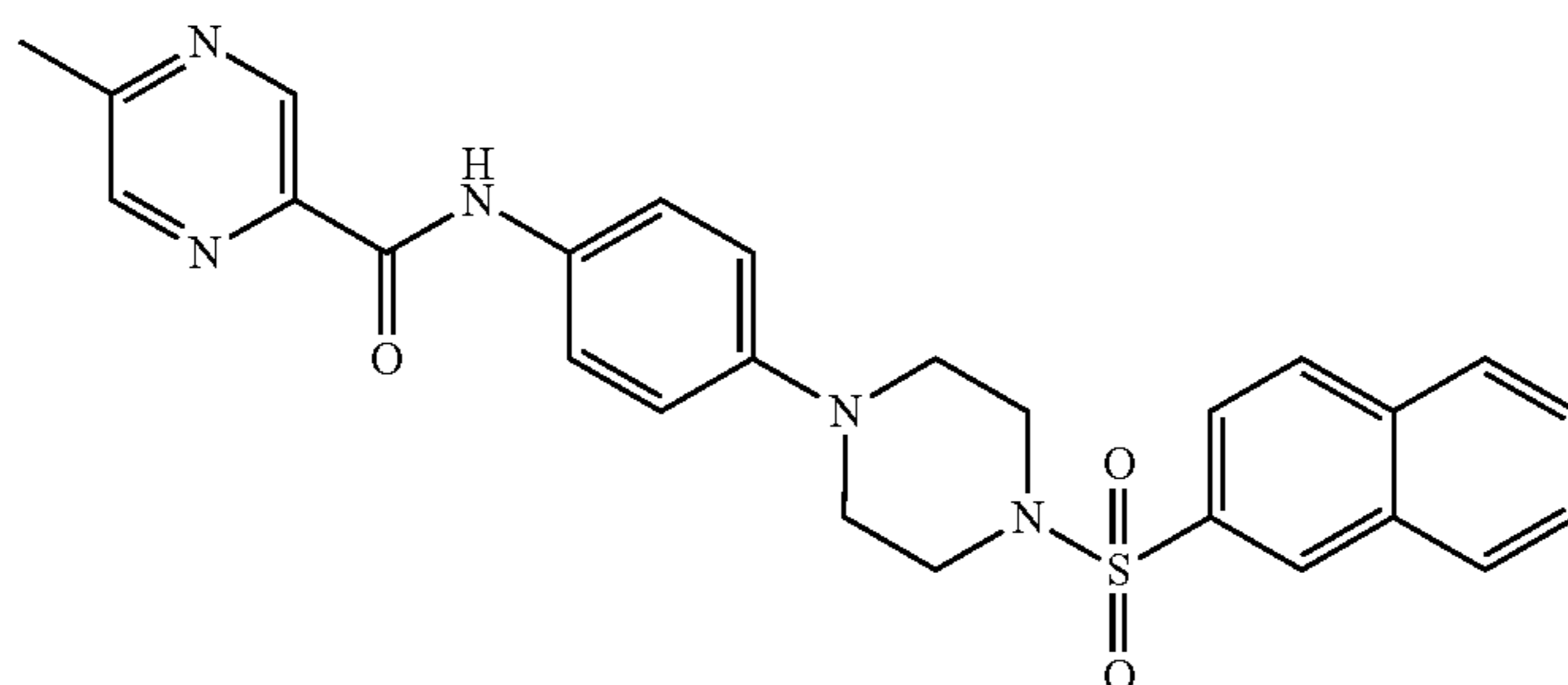
Co. No. 85; Ex. [B6]; mp. 250° C.
