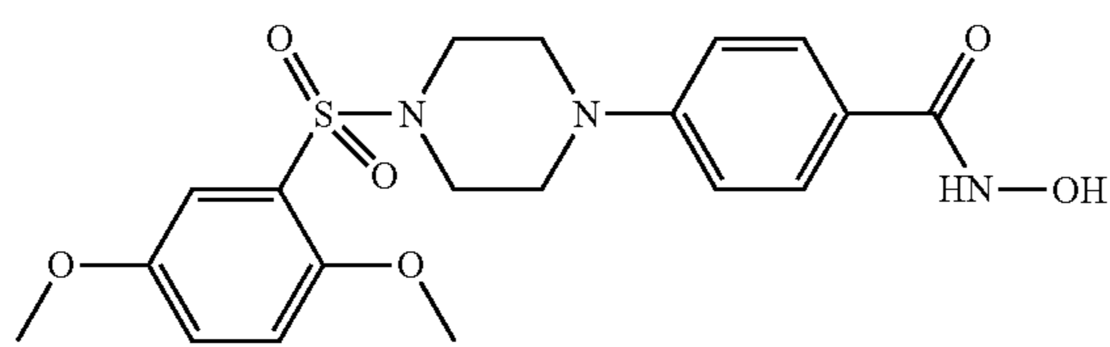
Co. No. 77; Ex. [B1]
