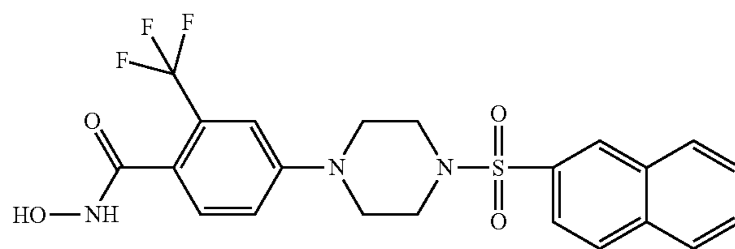
Co. No. 11; Ex. [B12]; mp. 196° C.
