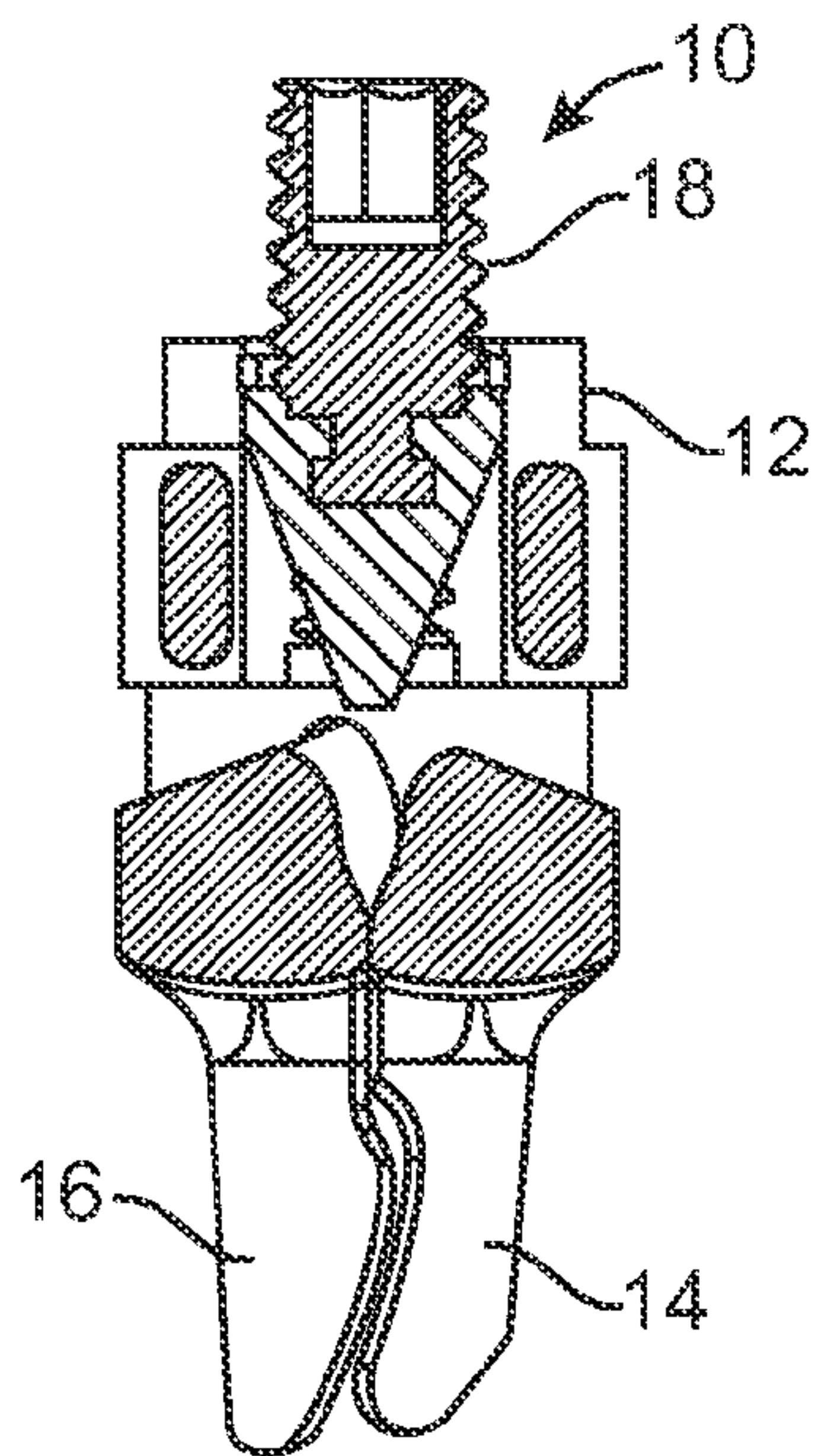
SECTION A-A
