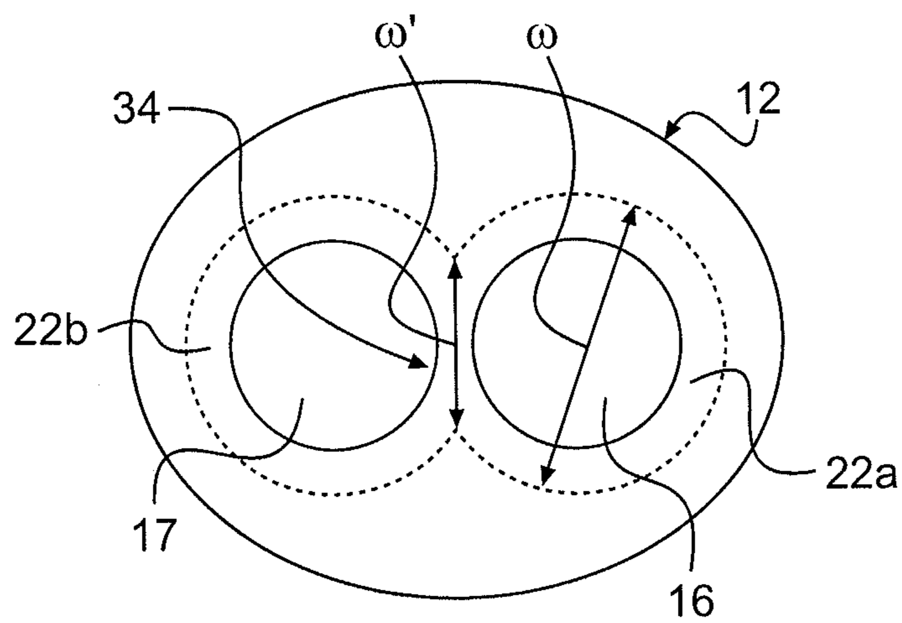
FIG. 6A
