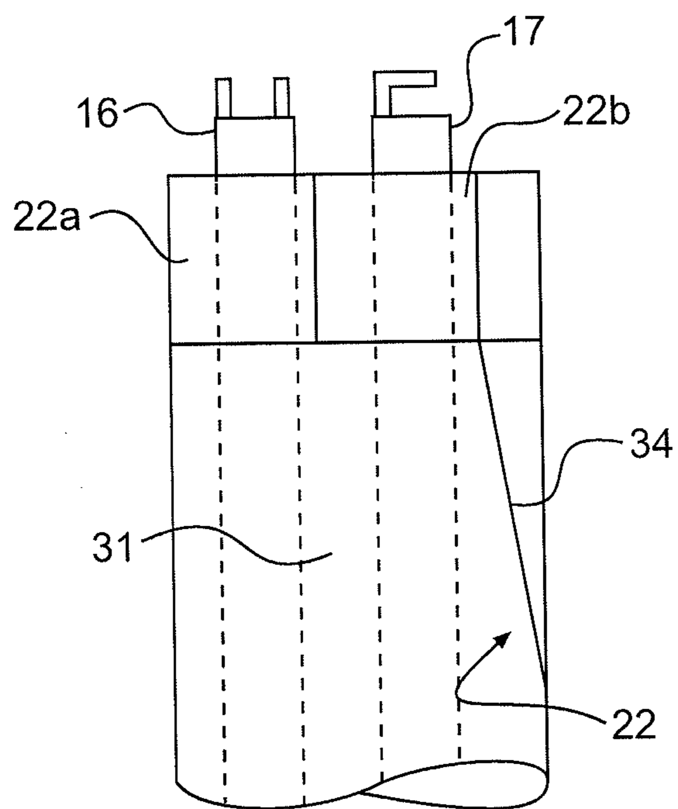
FIG. 7B
