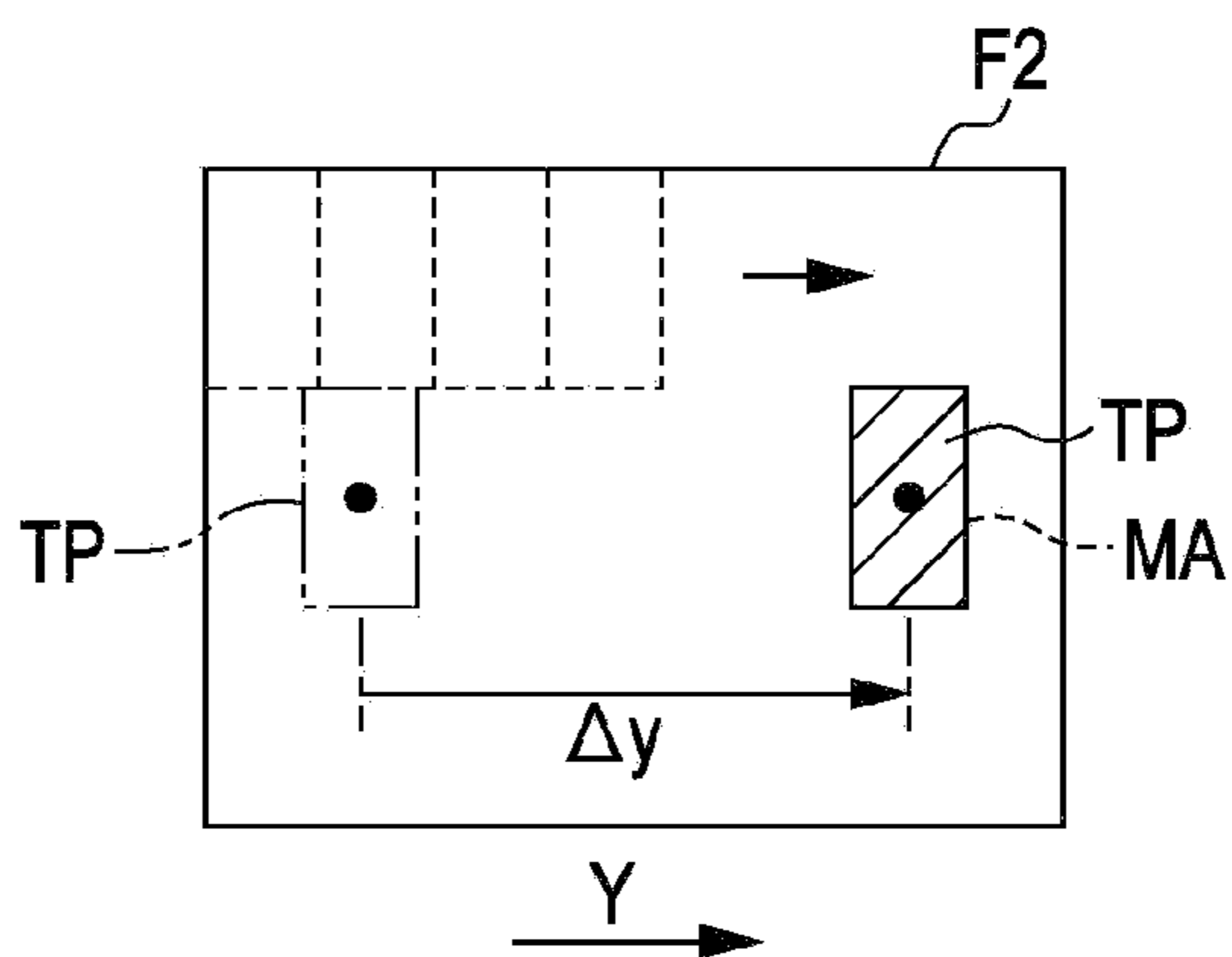
FIG. 5B TEMPLATE MATCHING
