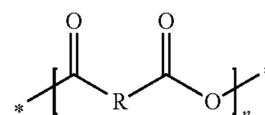
Polyanhydride
