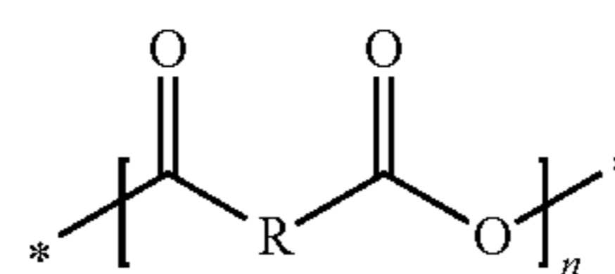
Polyanhydride
