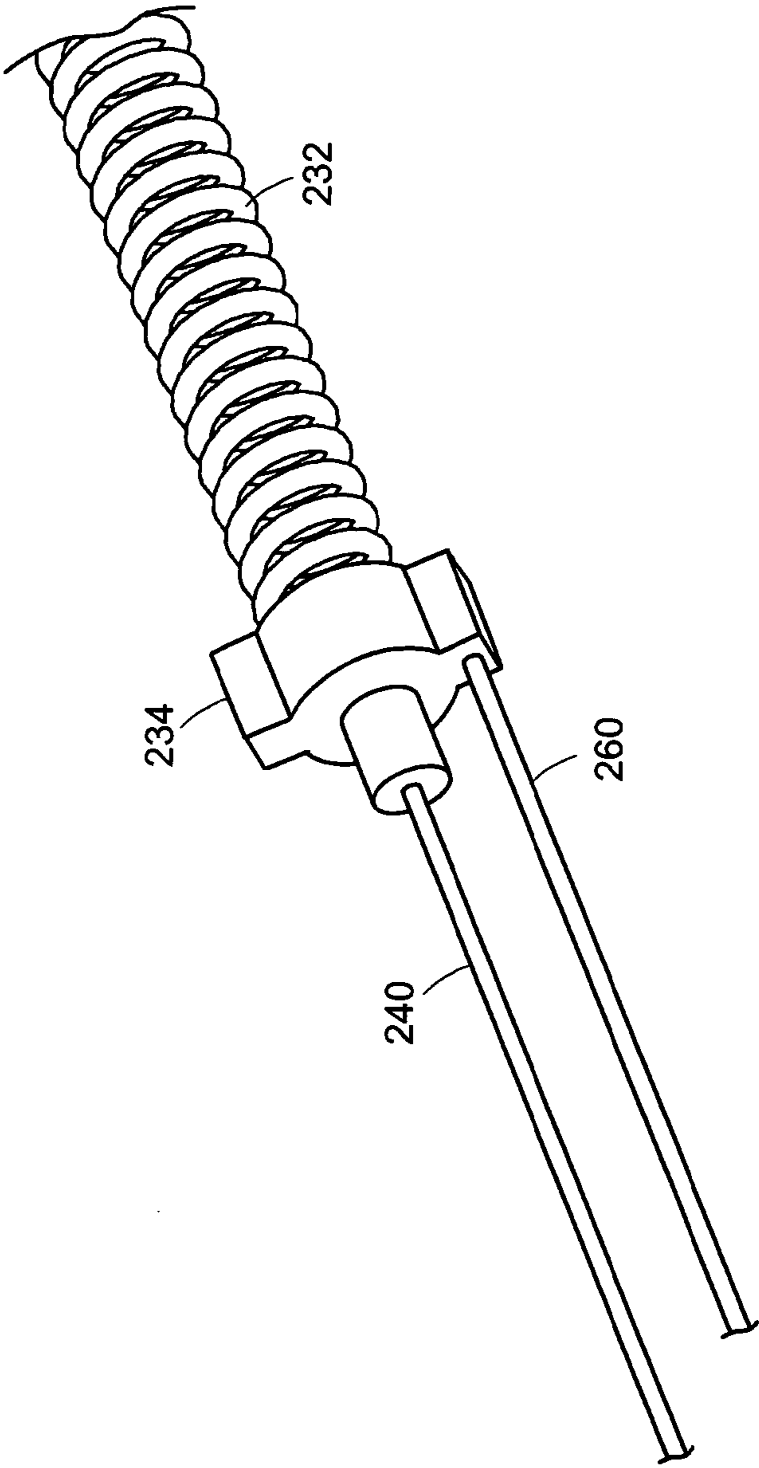
FIG. 2E
