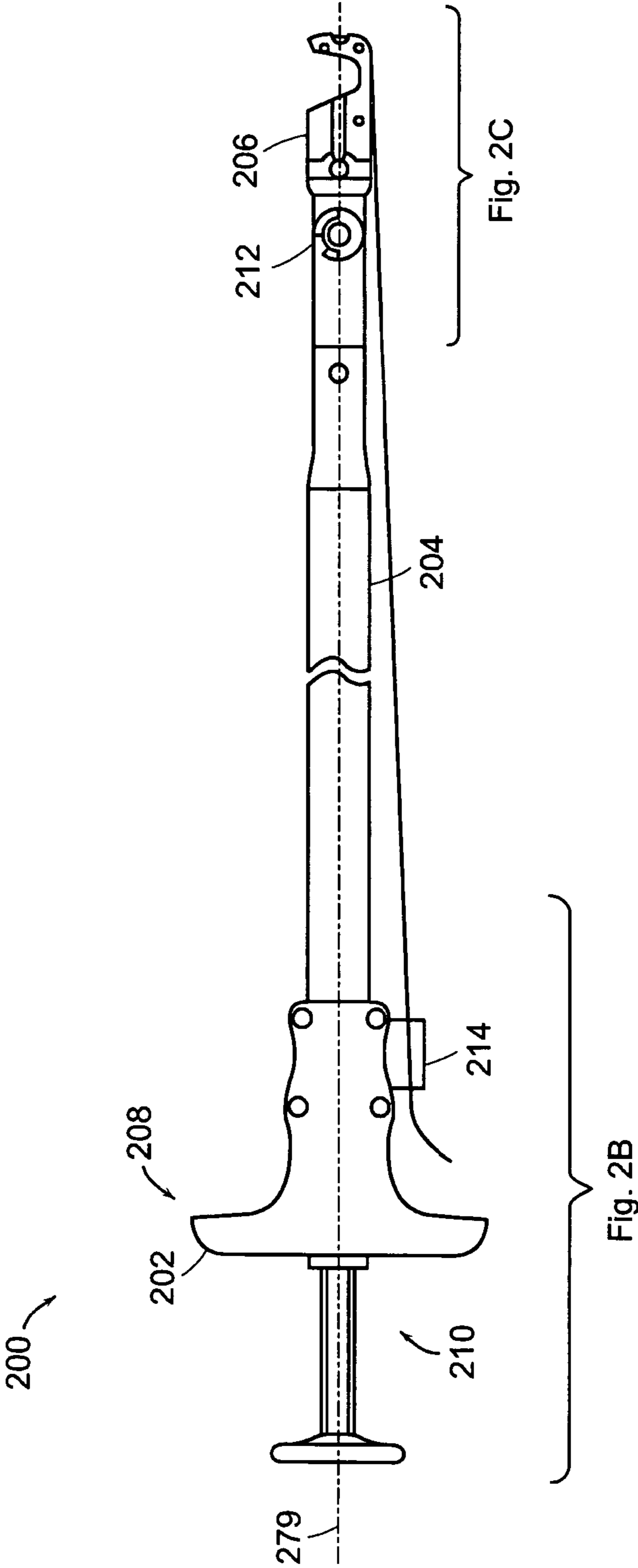
FIG. 2A
