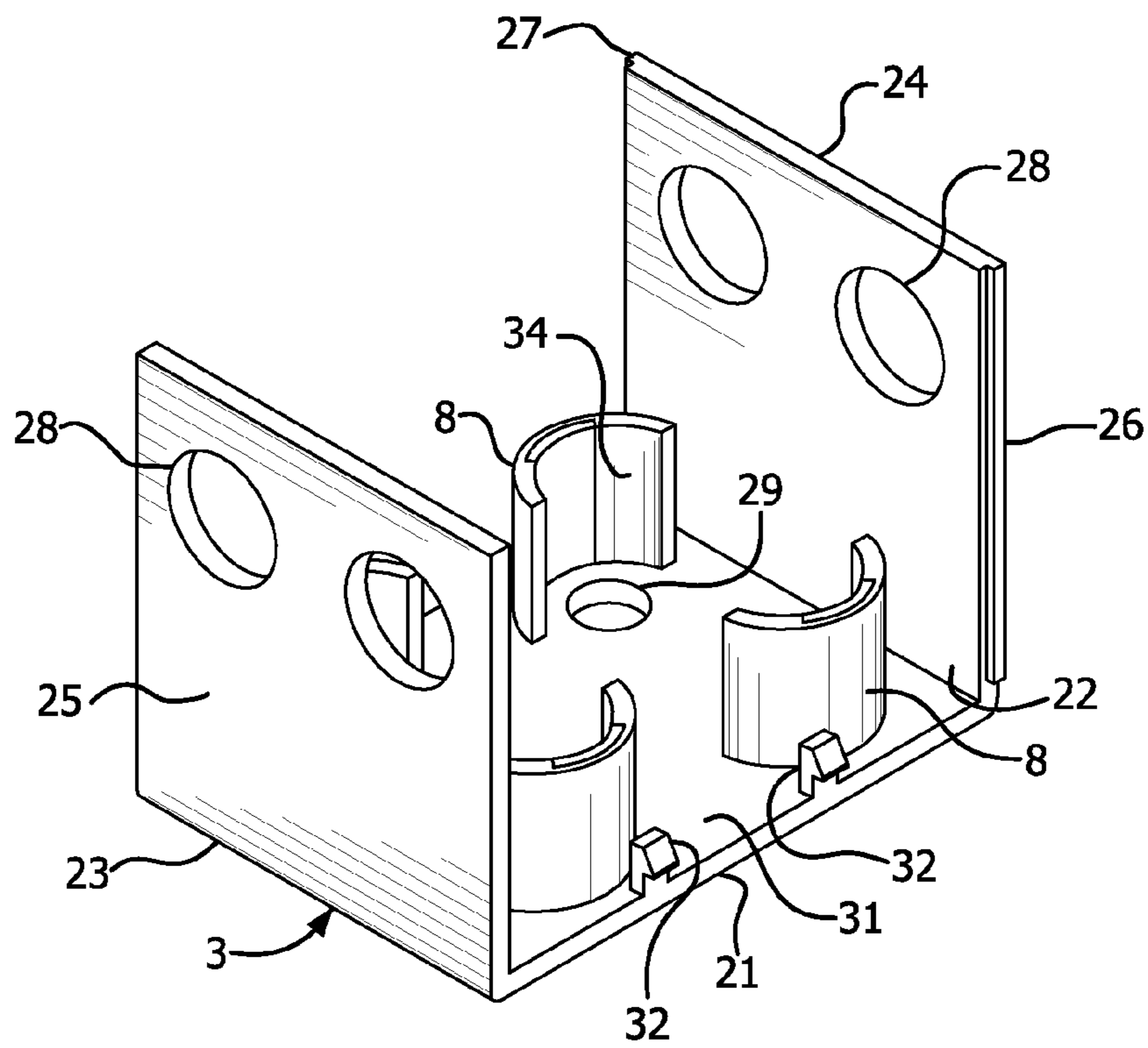
FIG. 10
