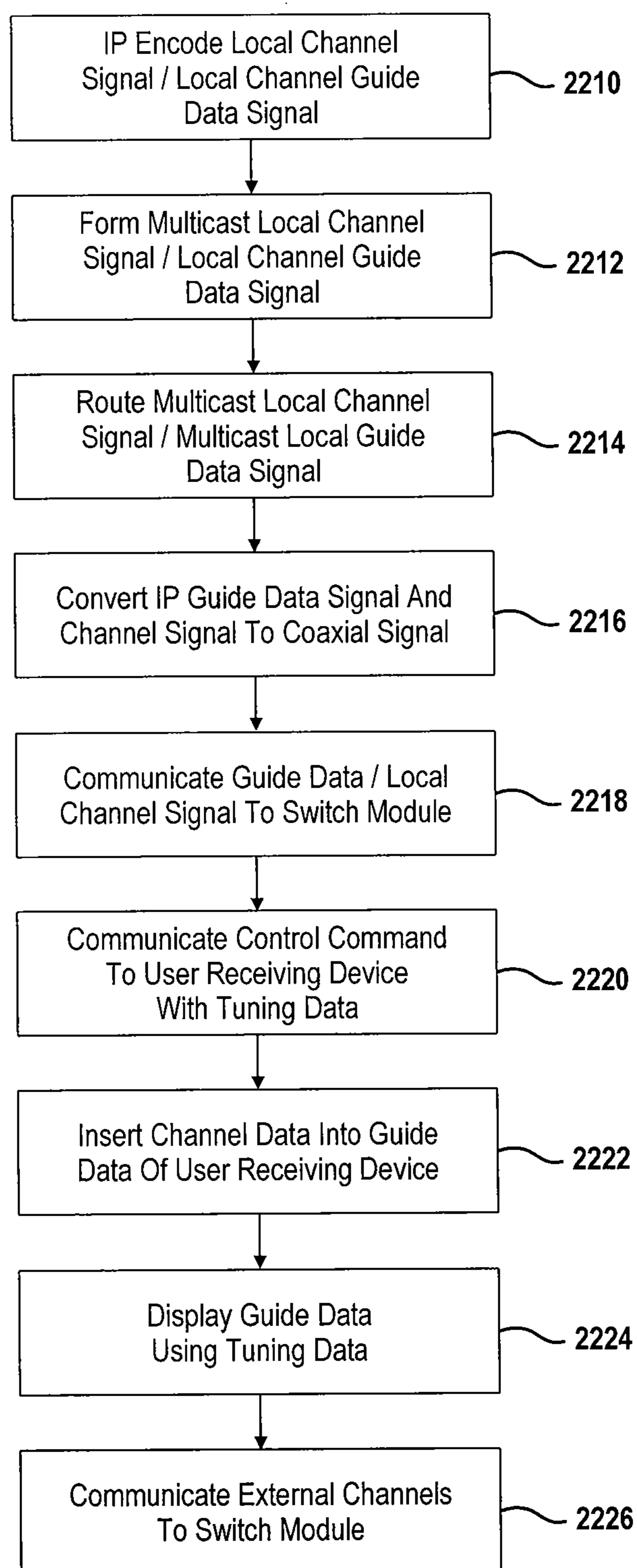
FIG. 22
