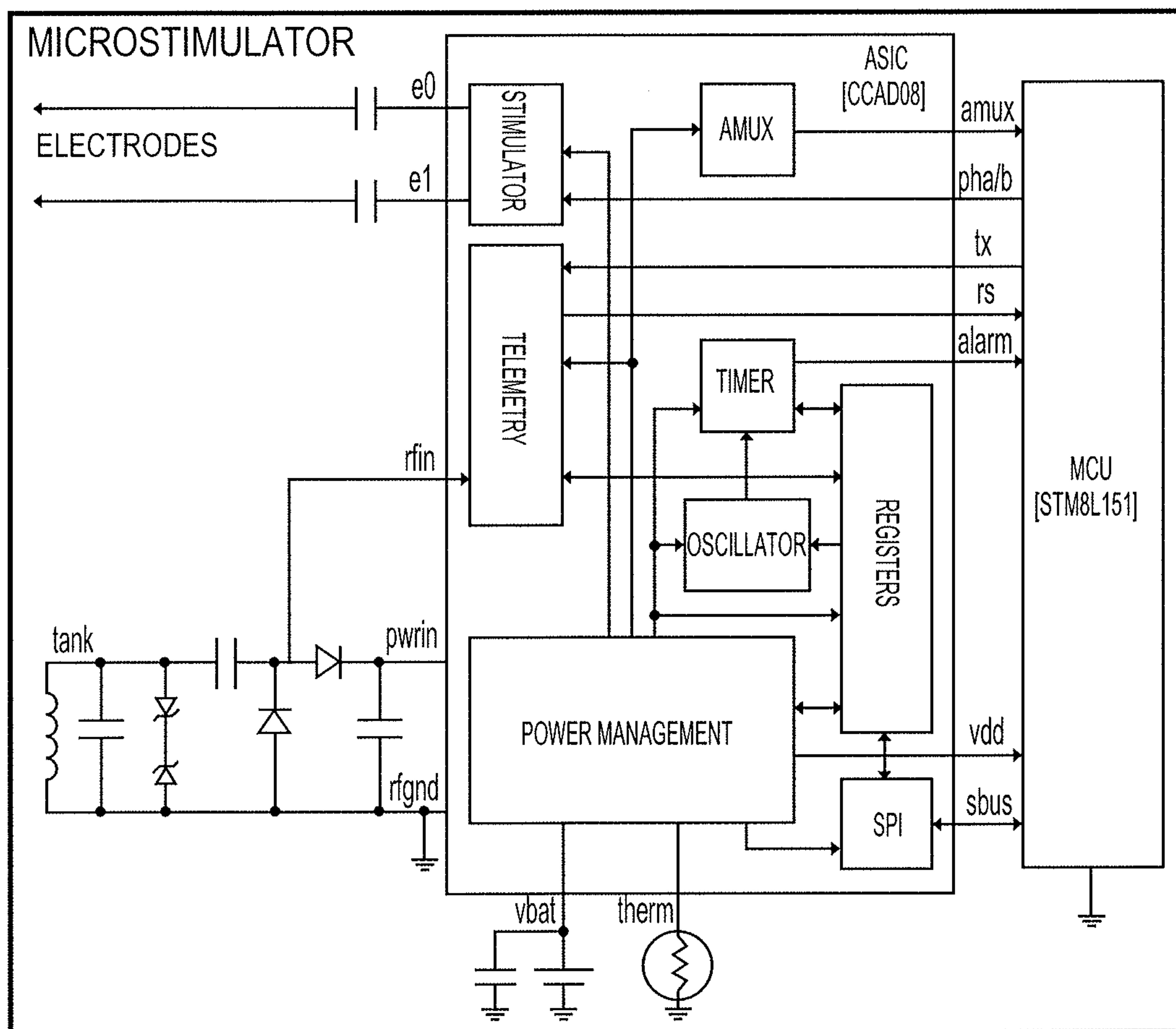
FIG. 24A
