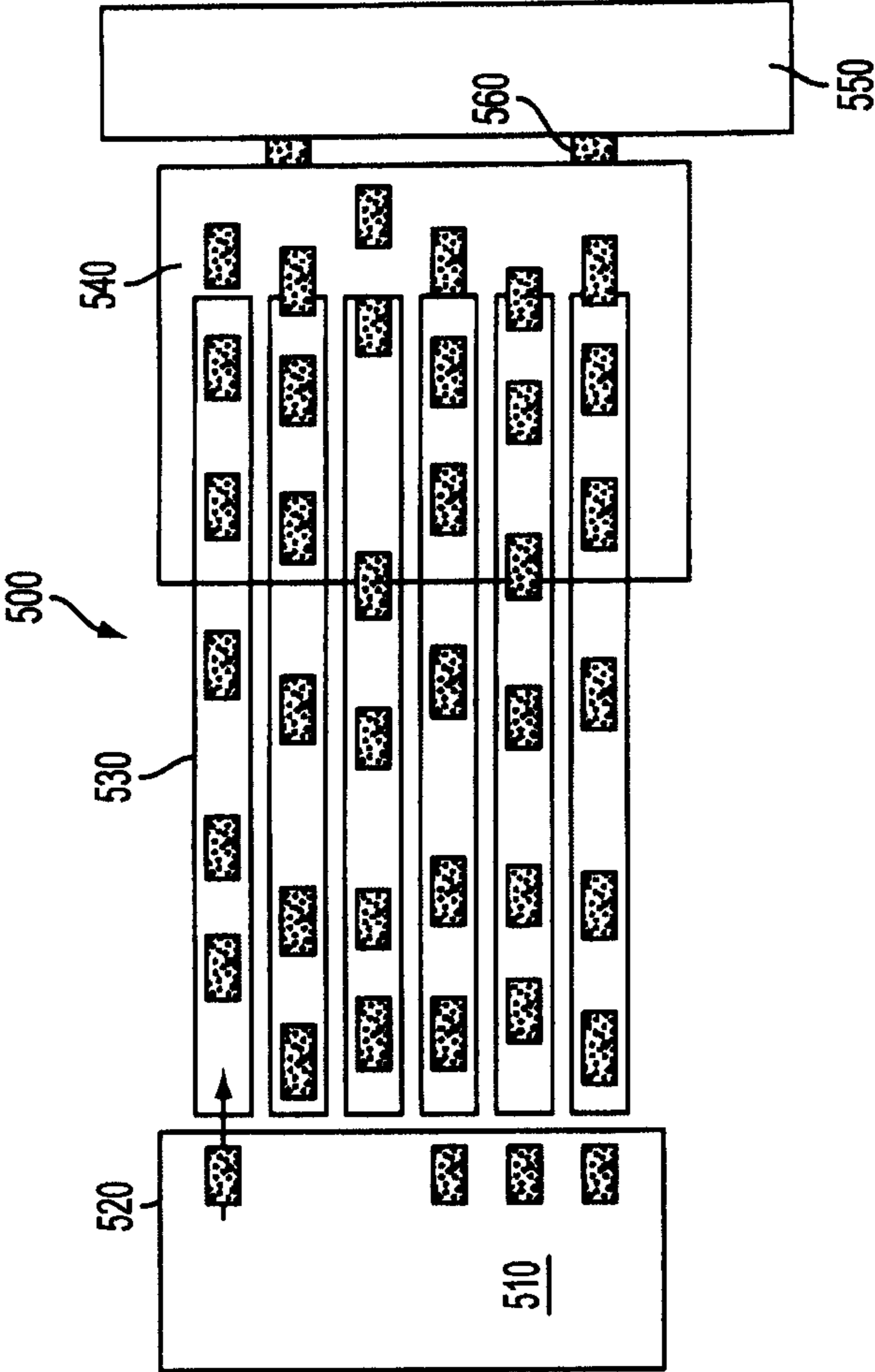
FIG. 7A
