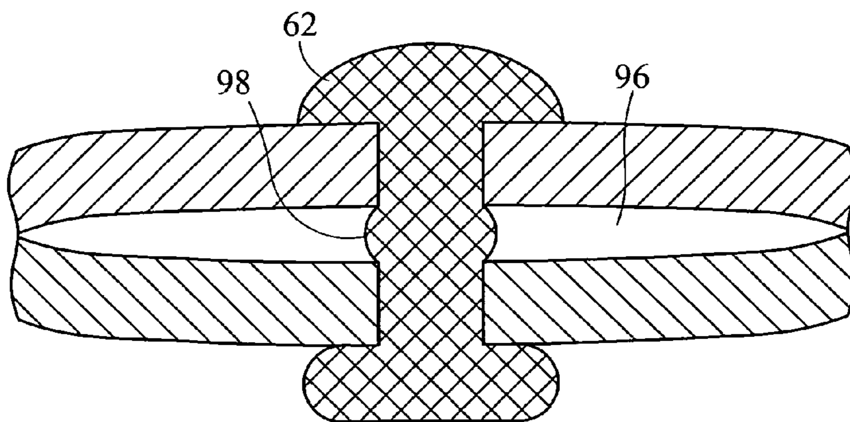
FIG. 4E PRIOR ART
