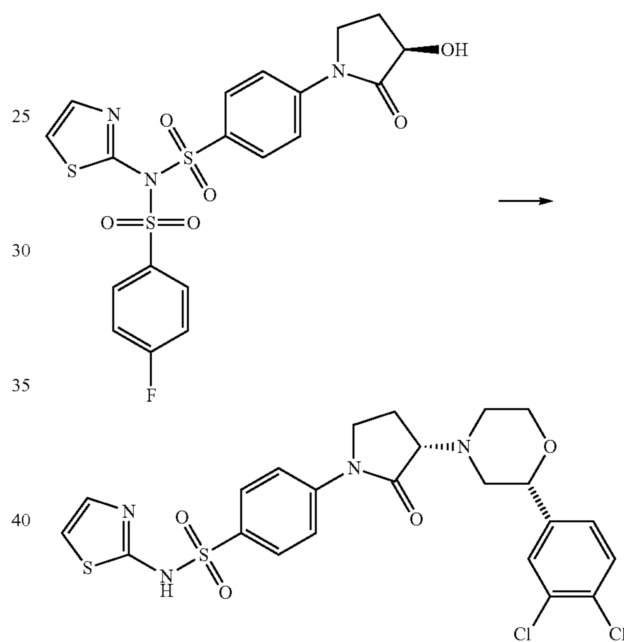
4-((S)-3-((R)-2-(3,5-dichlorophenyl)morpholino)-2-oxopyrrolidin-1-yl)-N-(thiazol-2-yl)benzenesulfonamide
