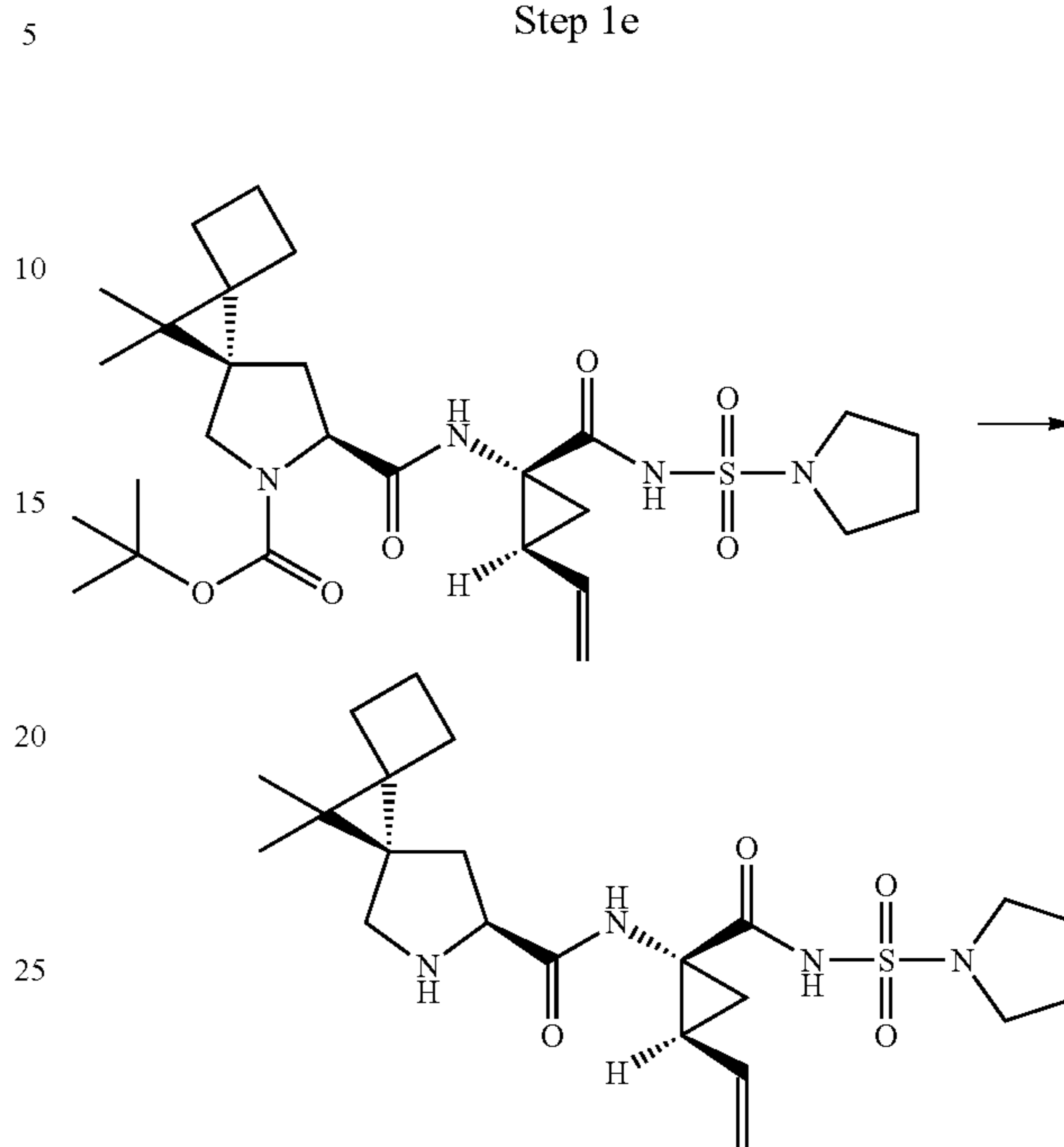
Compound 1e
