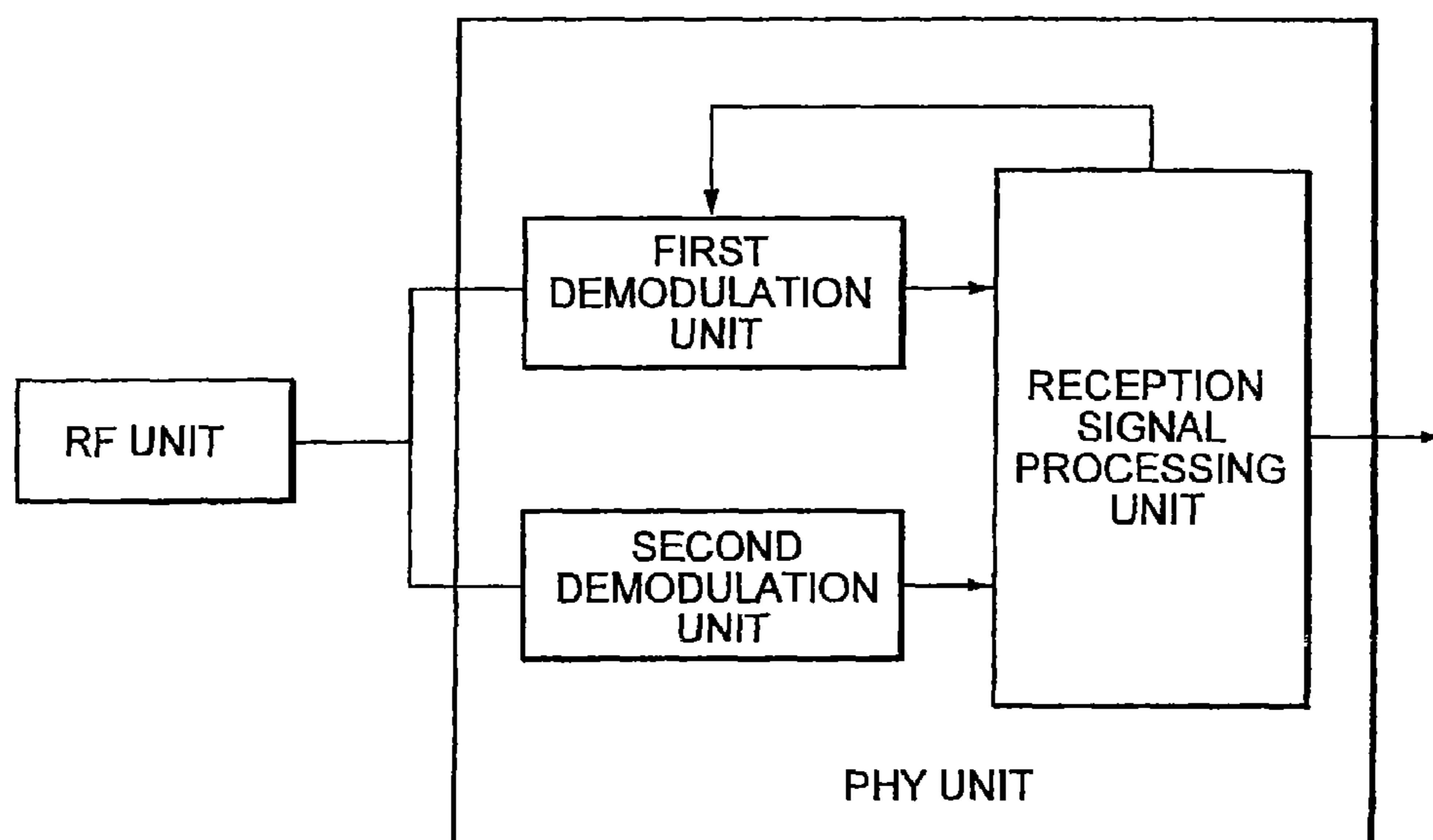
FIG. 15
