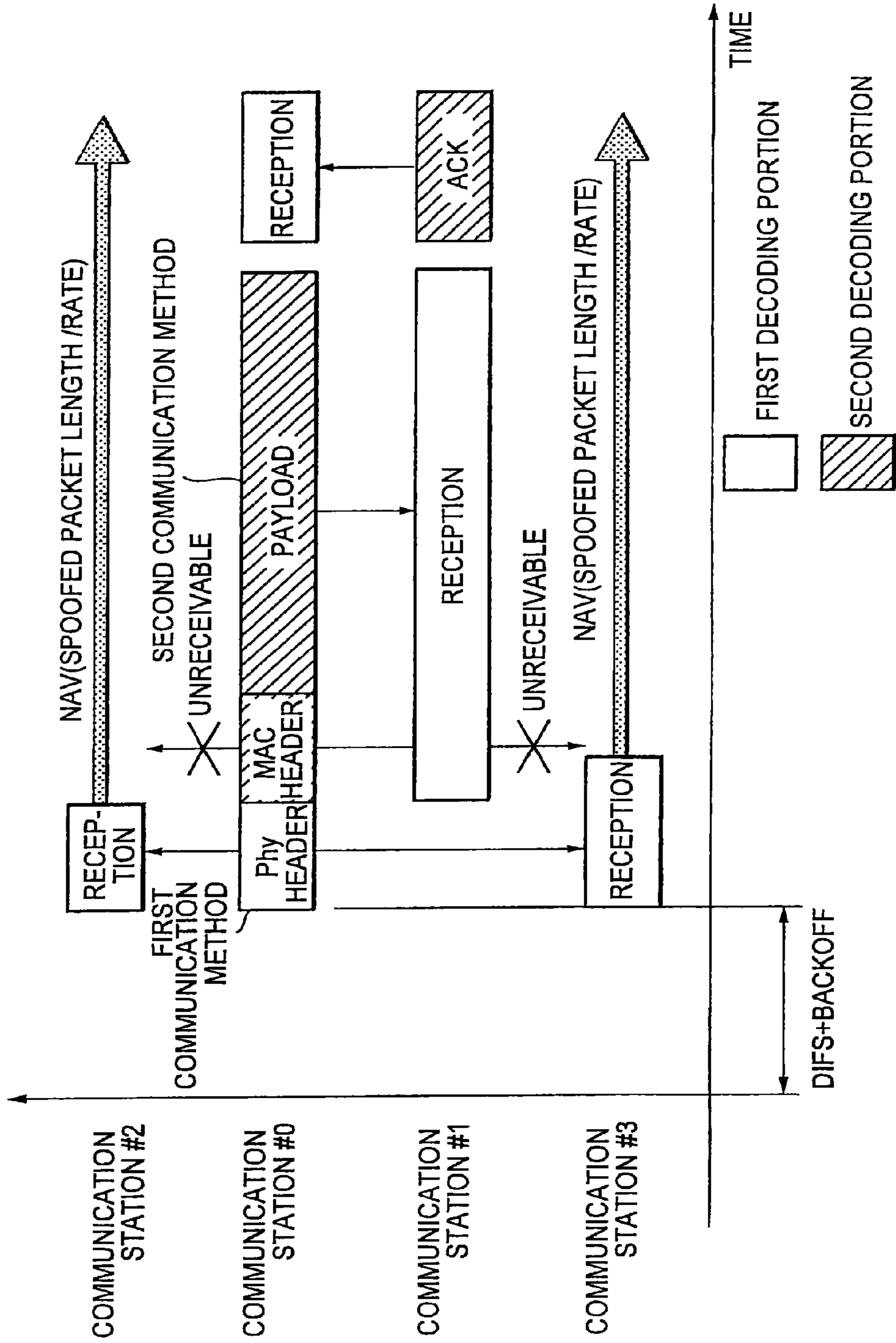
FIG. 8
