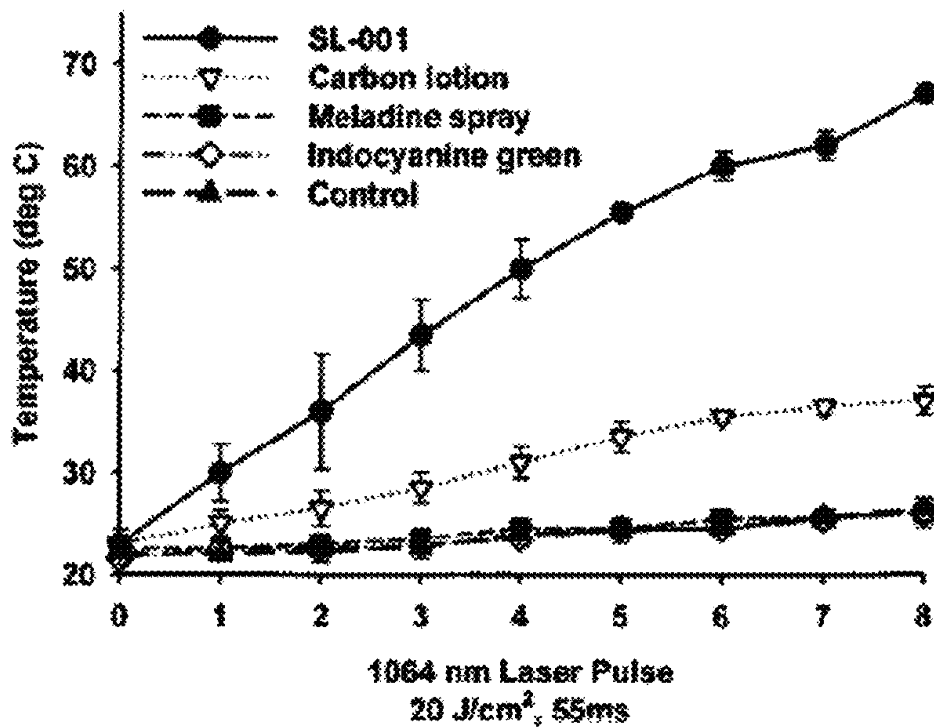
FIG. 11A
