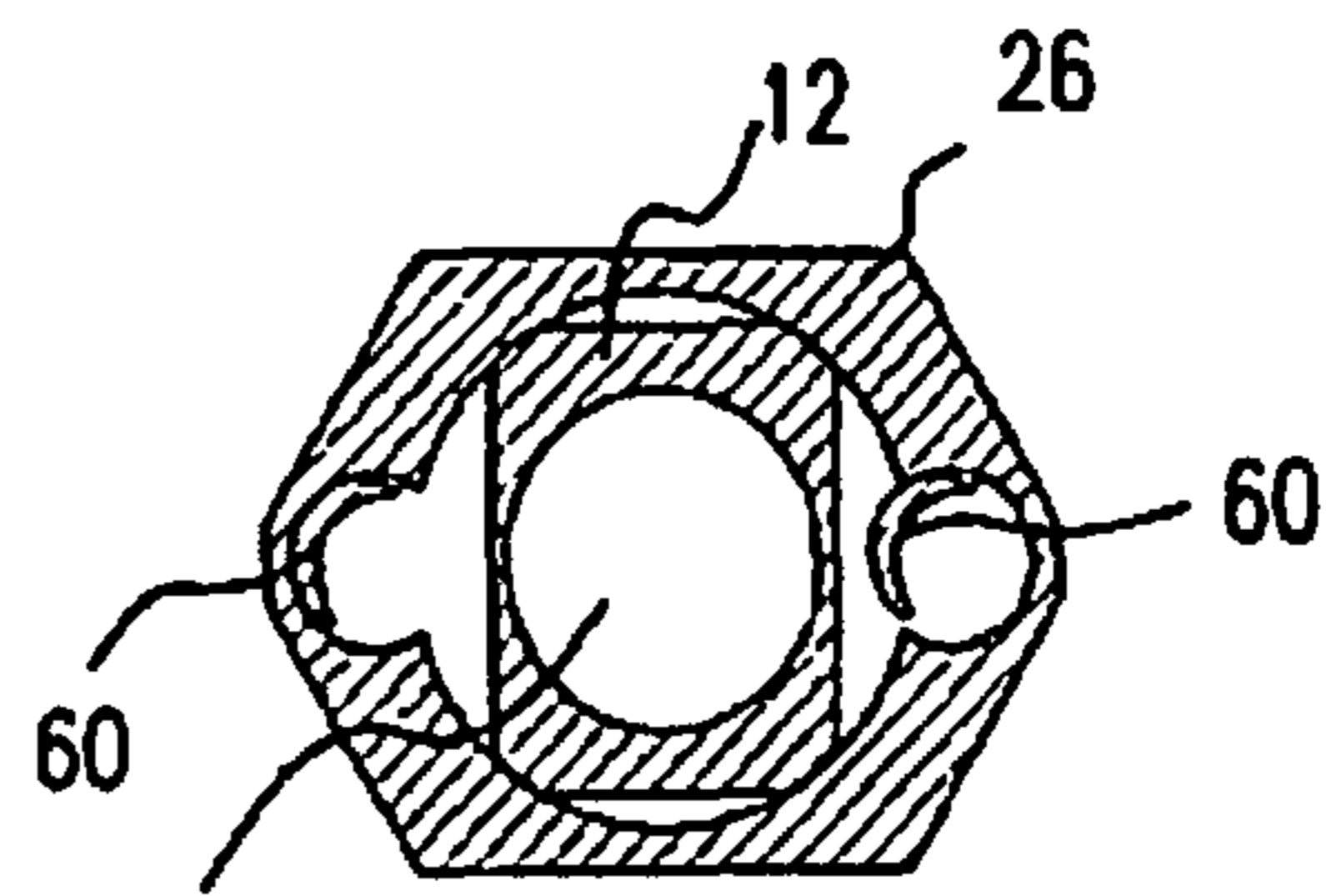
SECTION B-B SCALE 2:1
