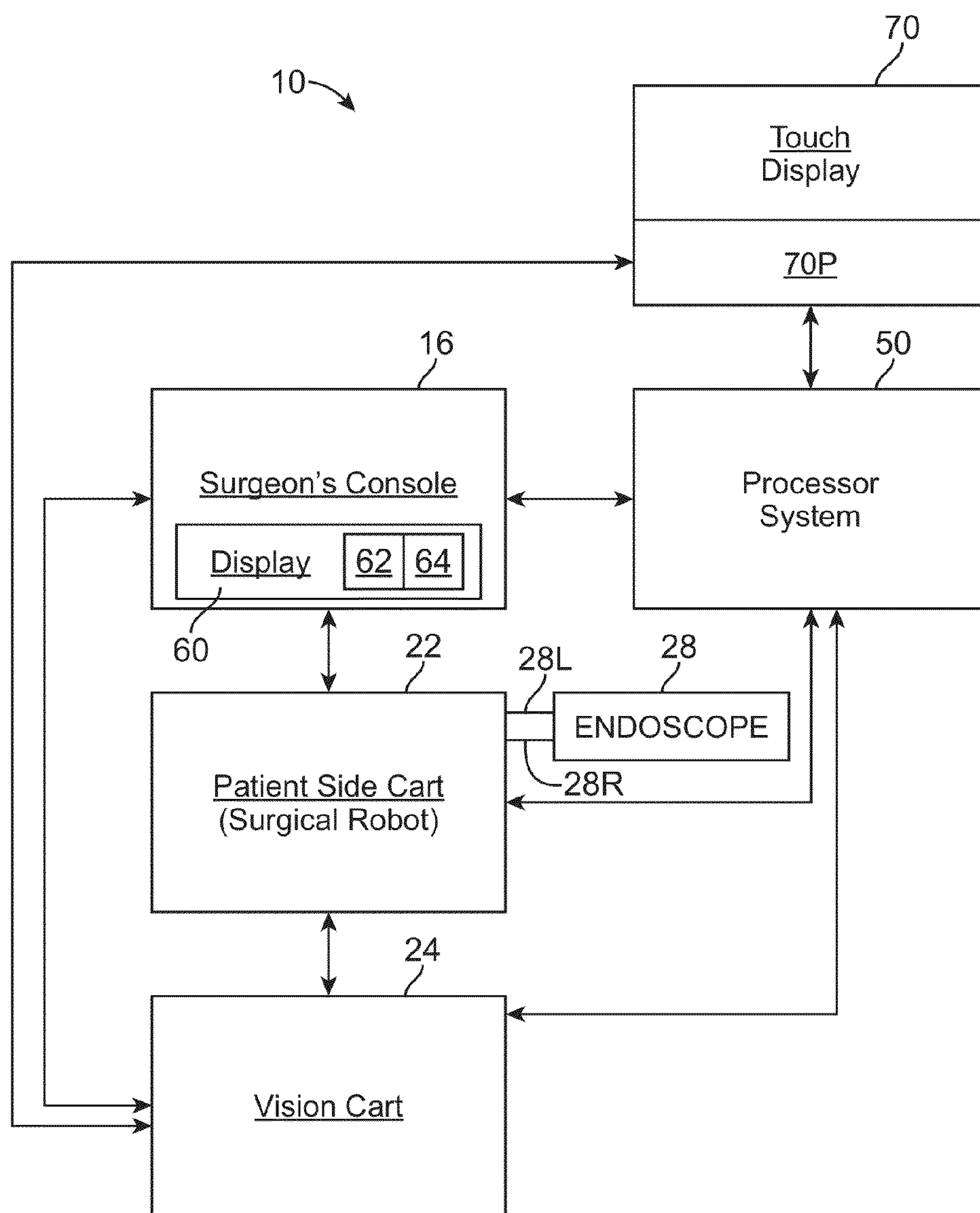
FIG. 1E
