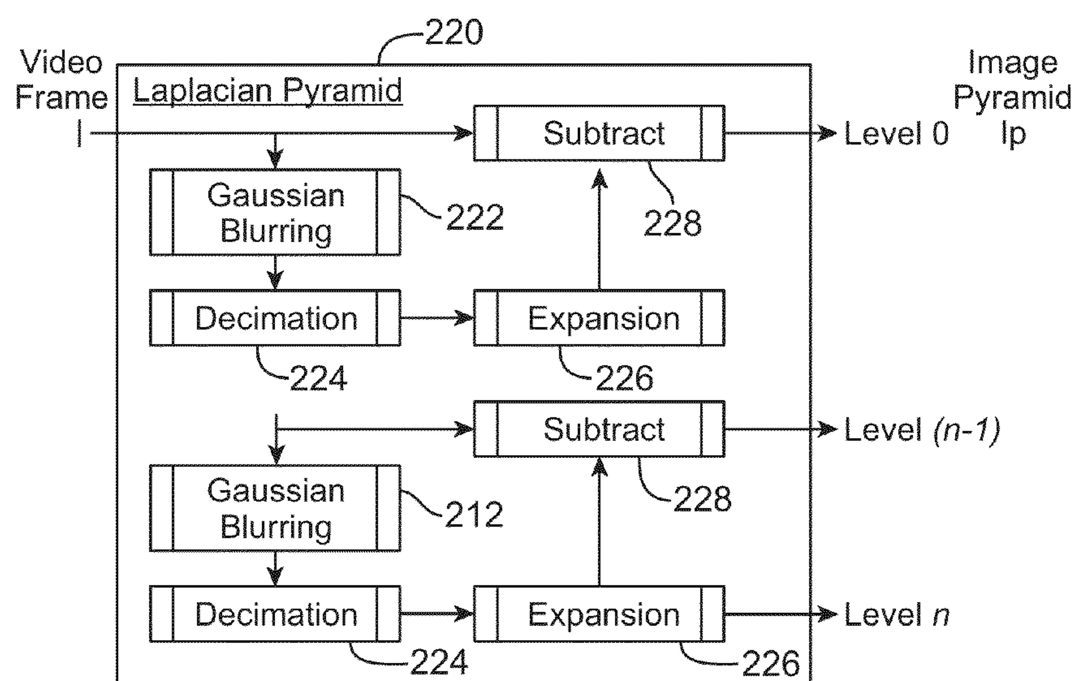
FIG. 2B
