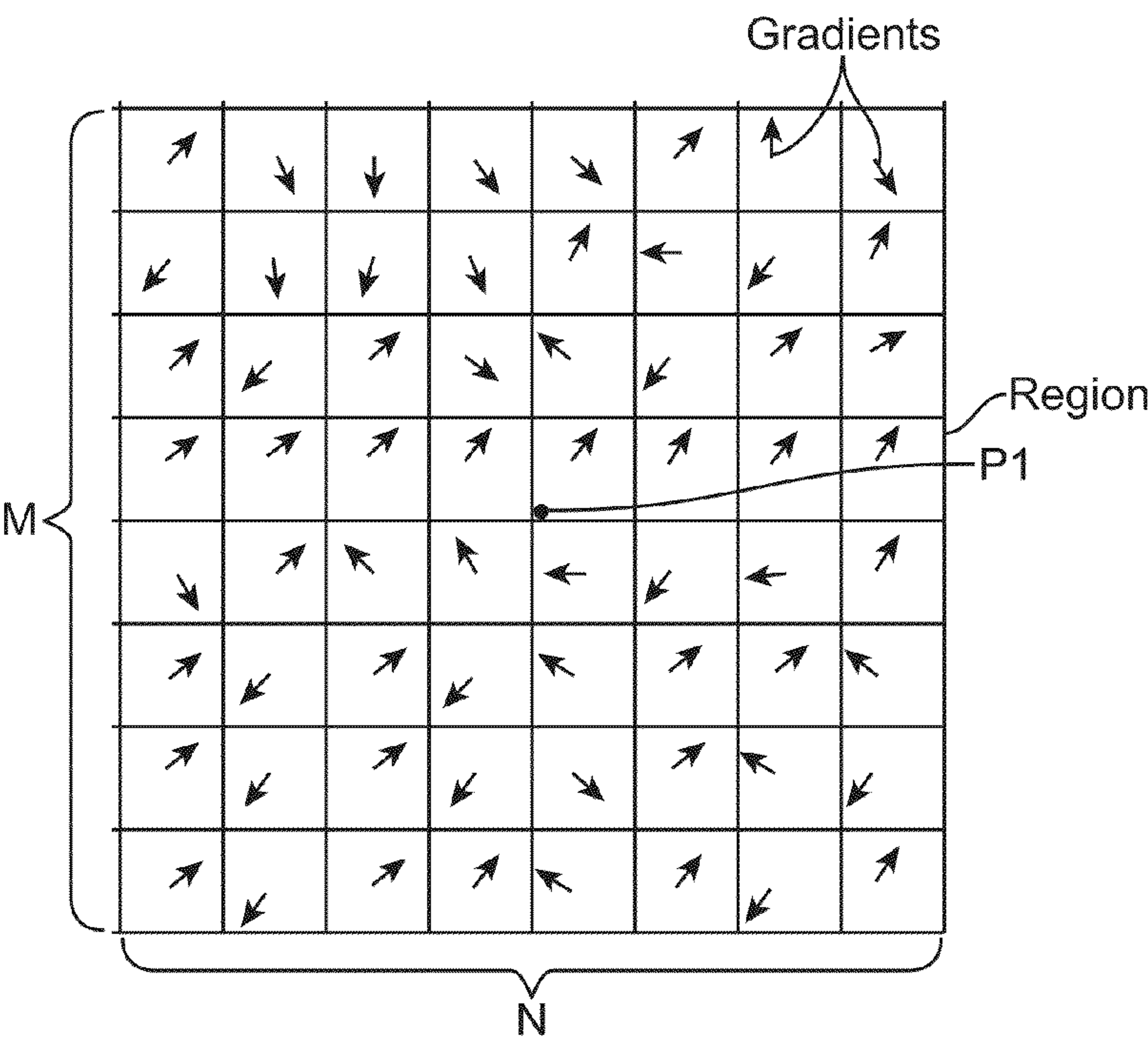
FIG. 2E1
