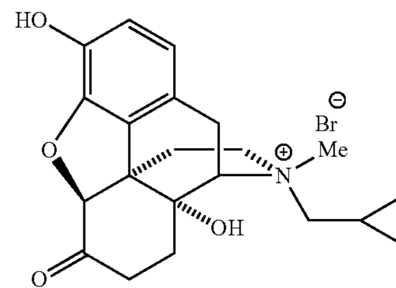
(+)S-Naltrexone methobromide
