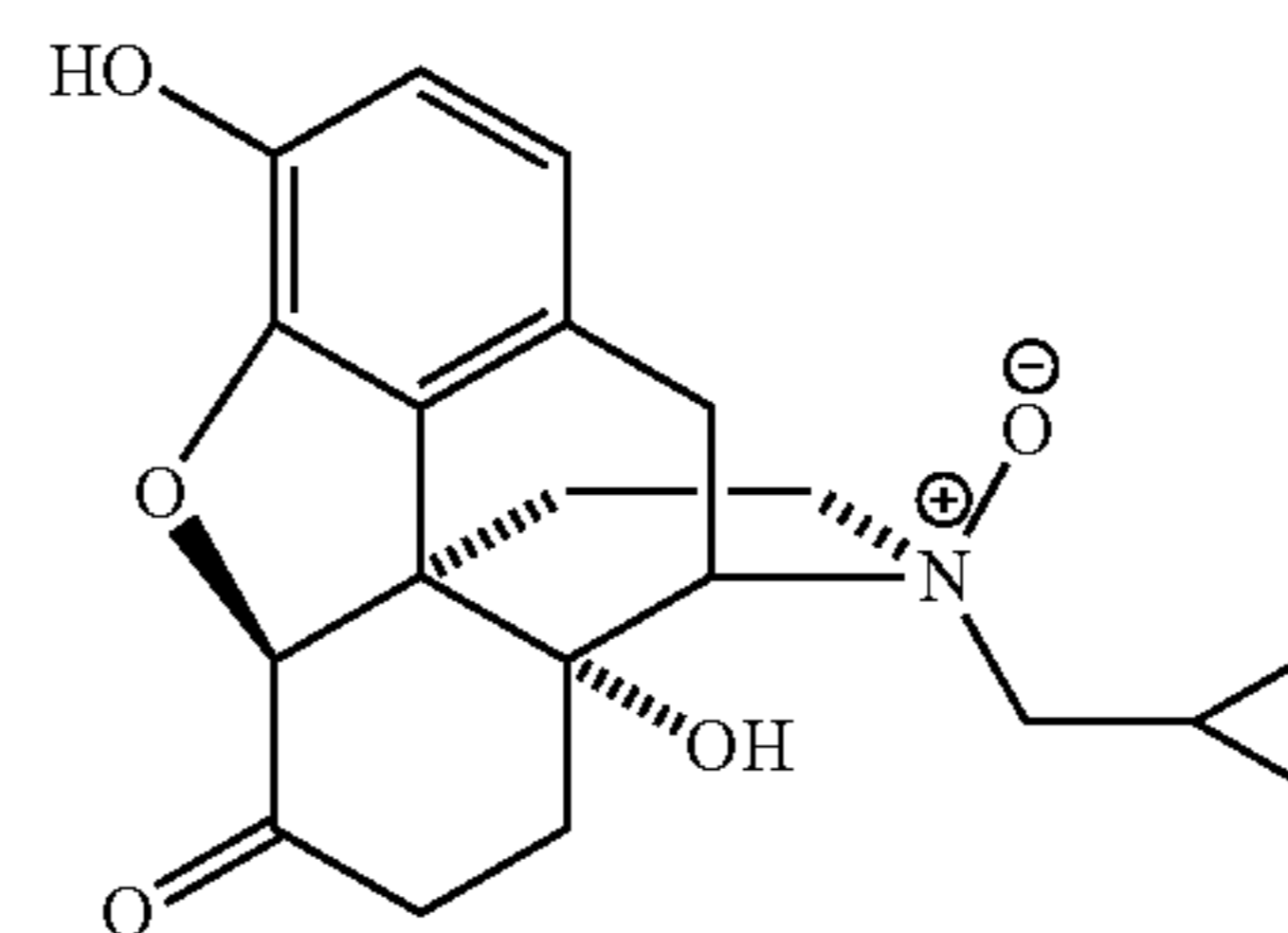
(+)Naltrexone N-Oxide
