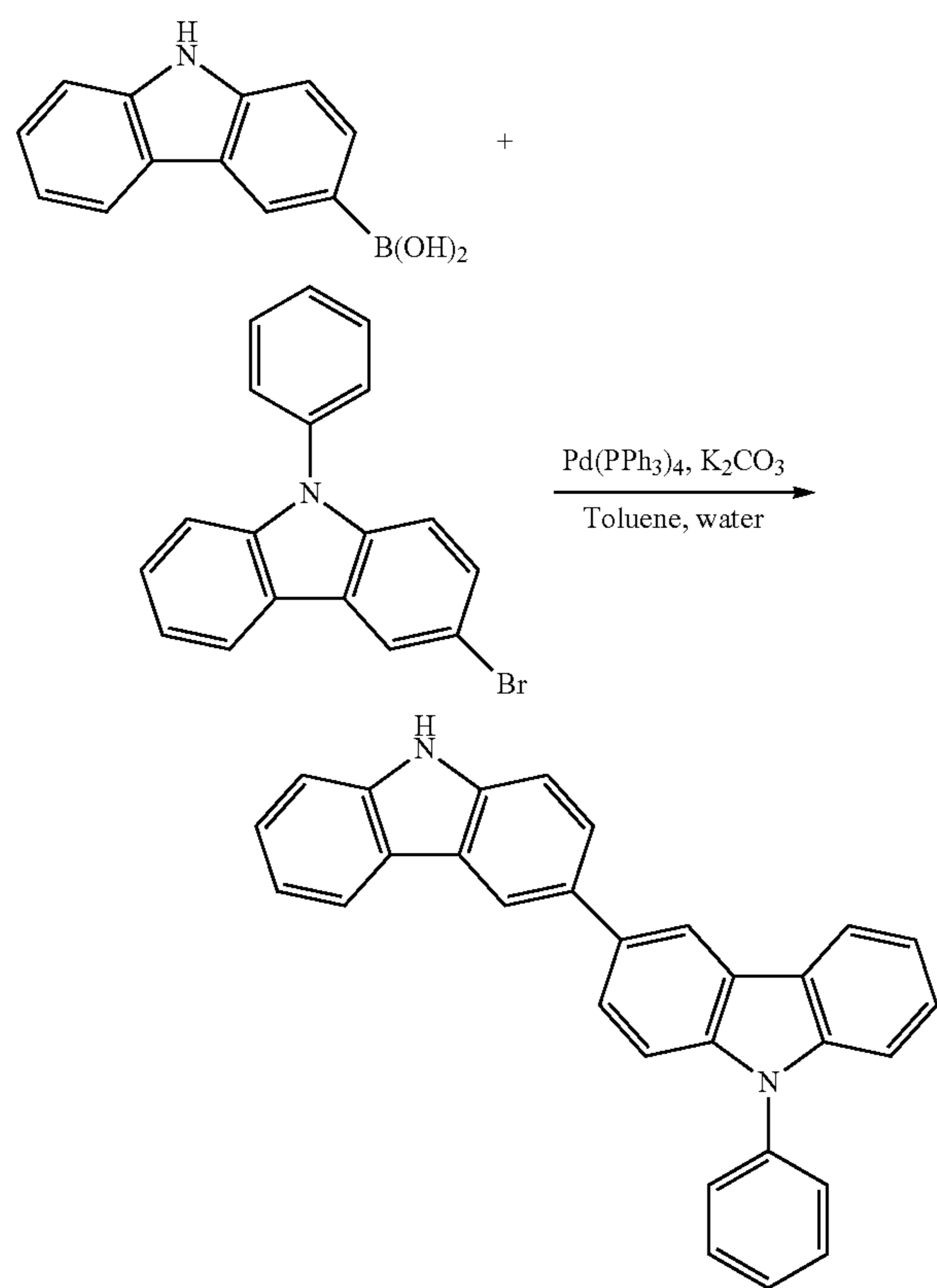
[13-a]
