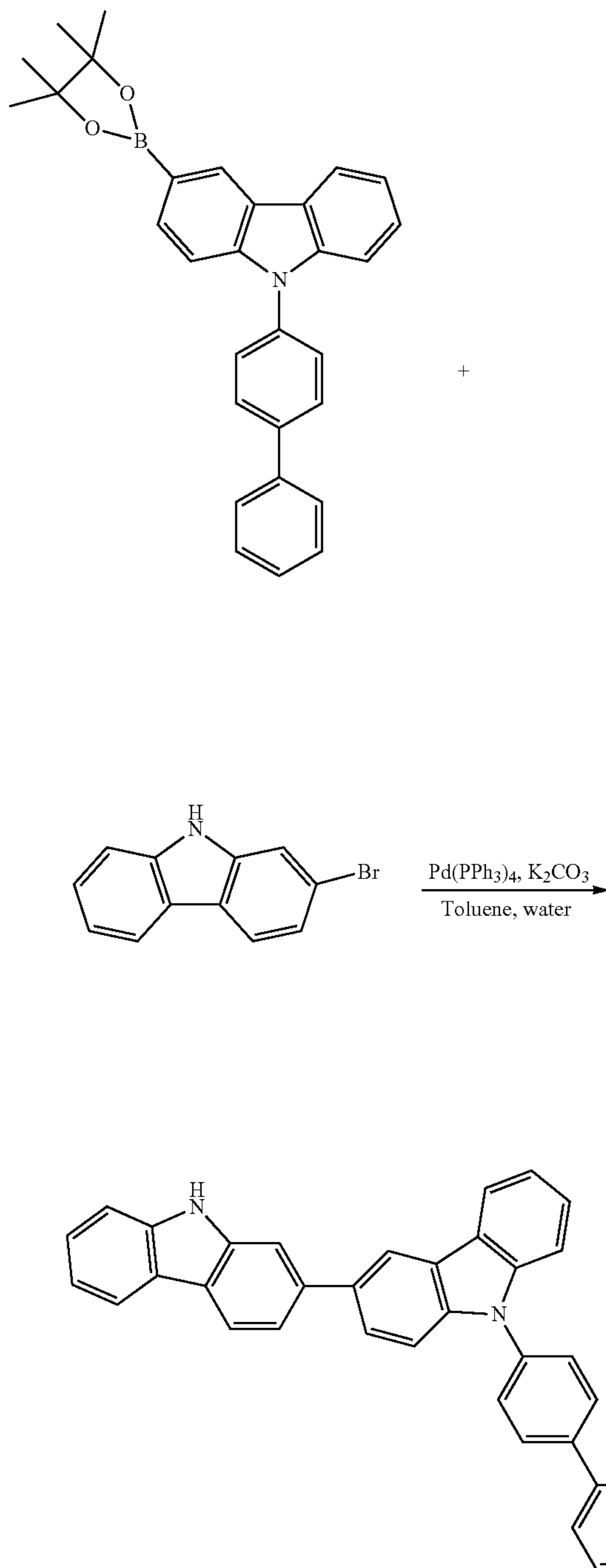
[29-a]
