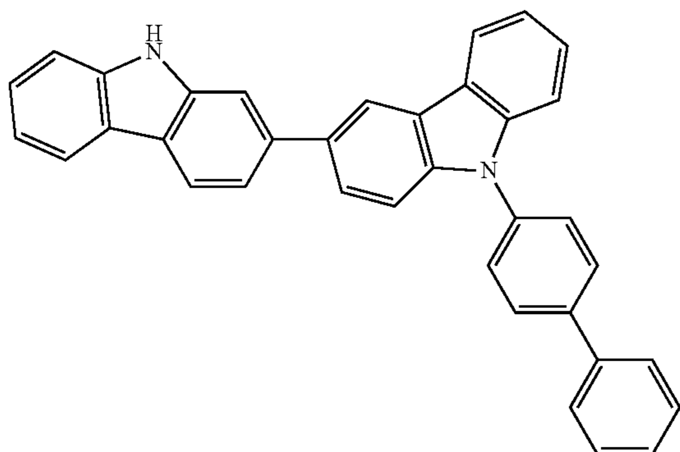
[27-a]
