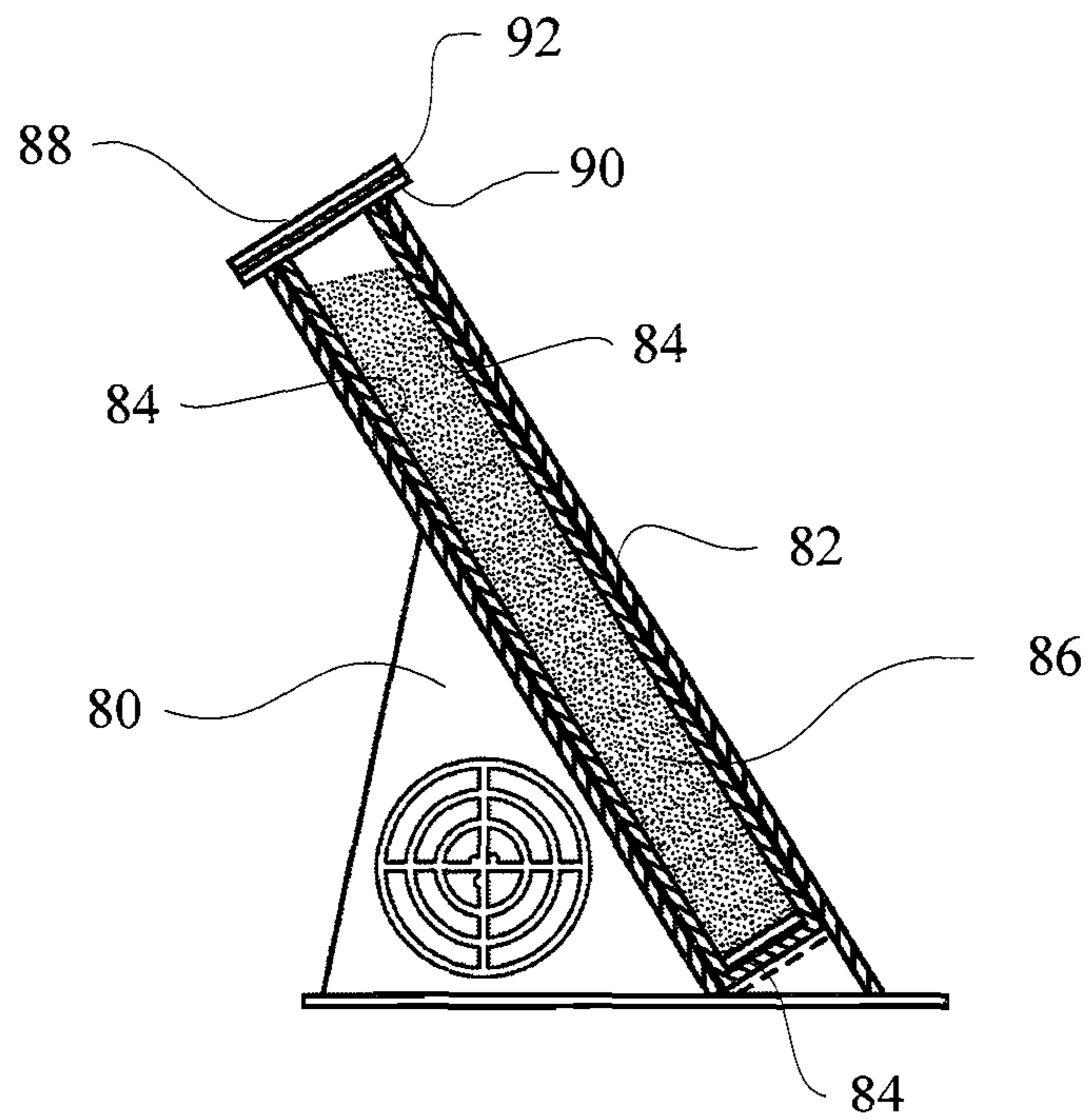
FIG. 1E (Prior Art)
