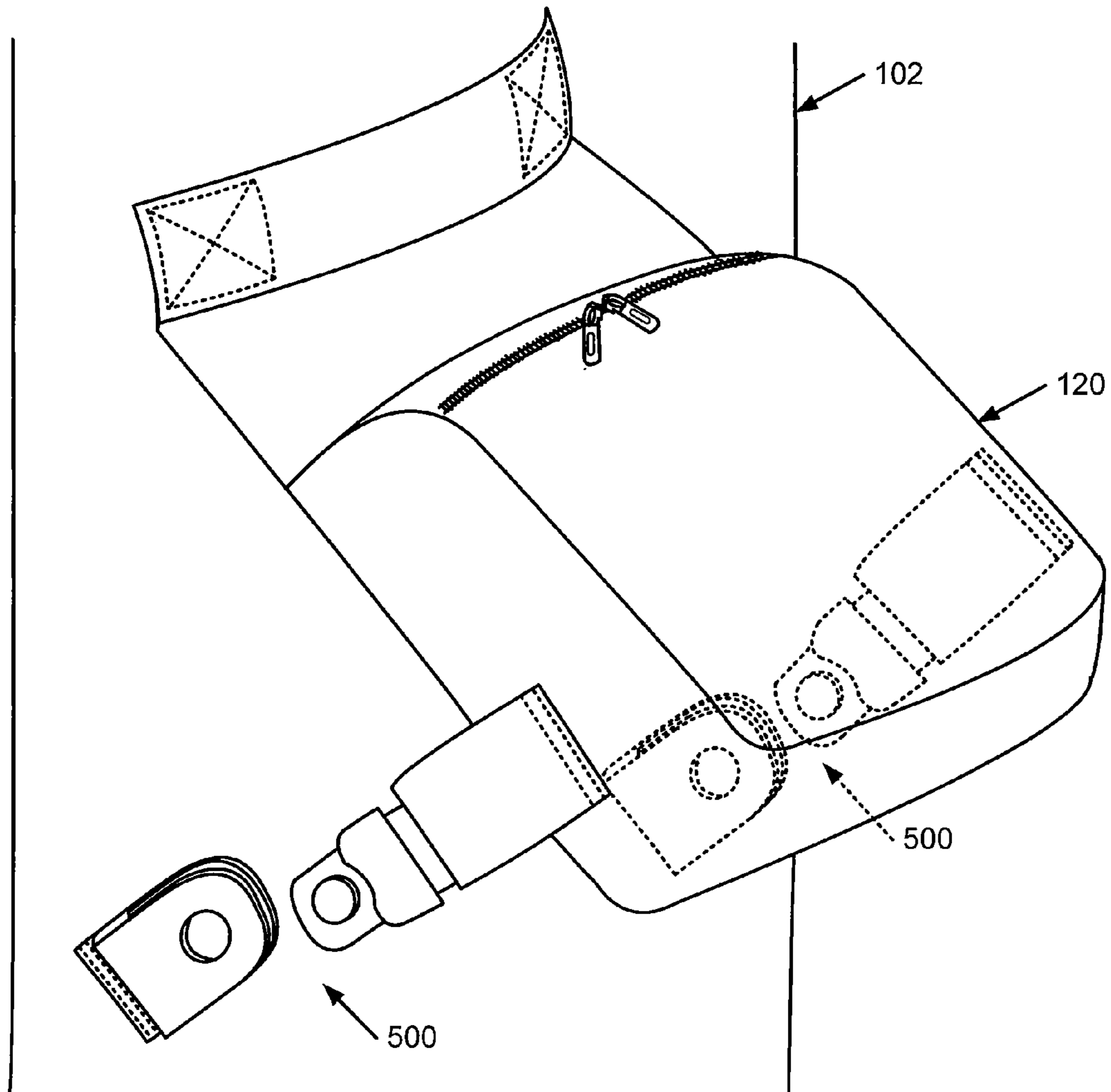
FIG. 5
