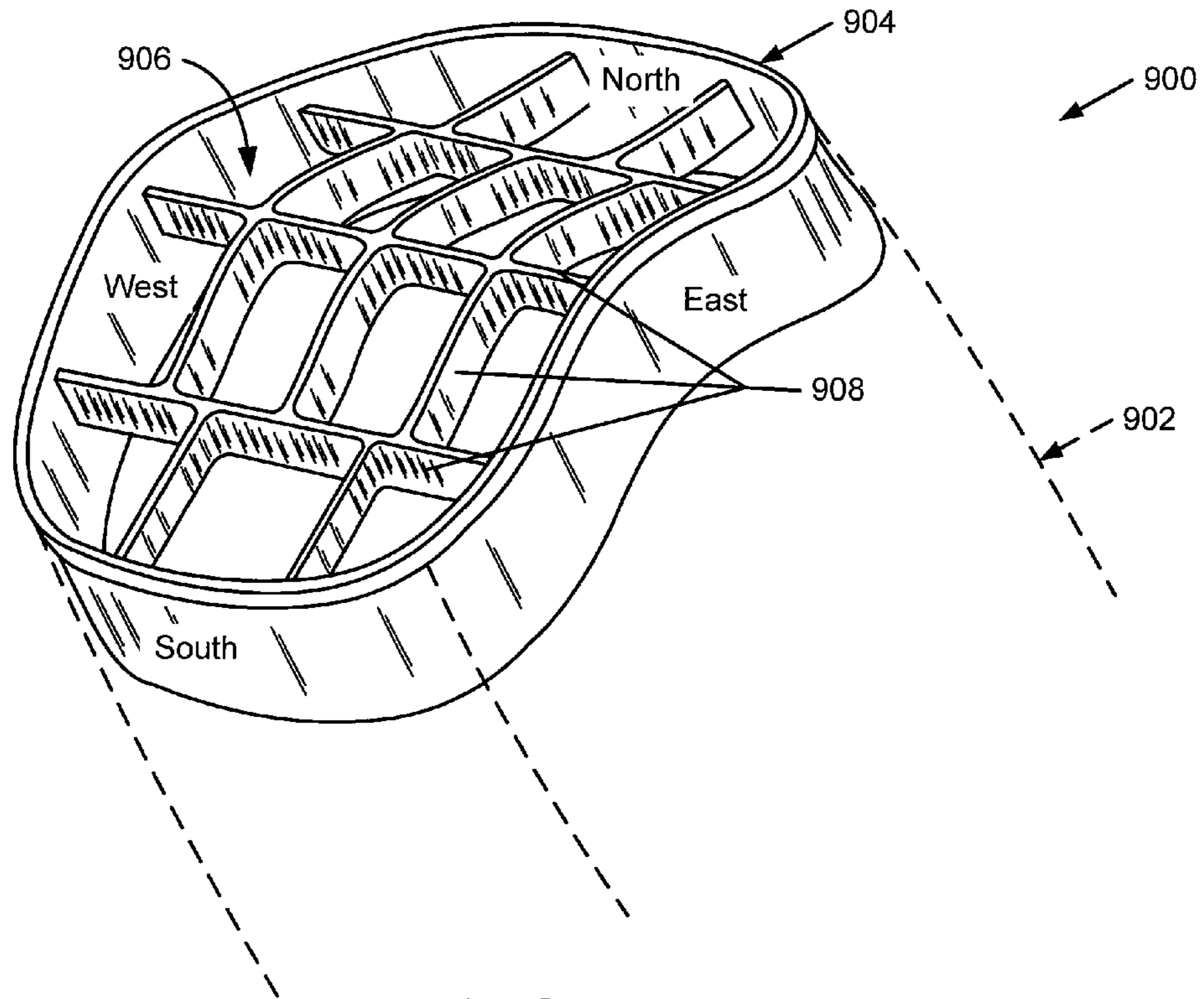
FIG. 9A
