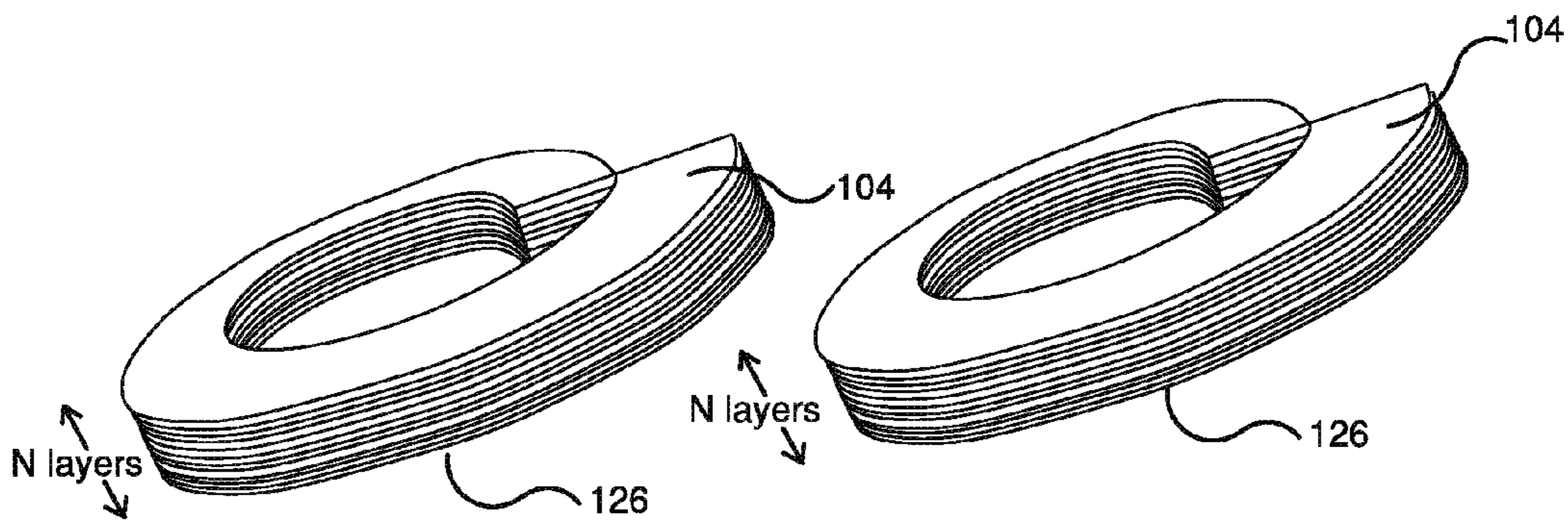
FIG. 7D
