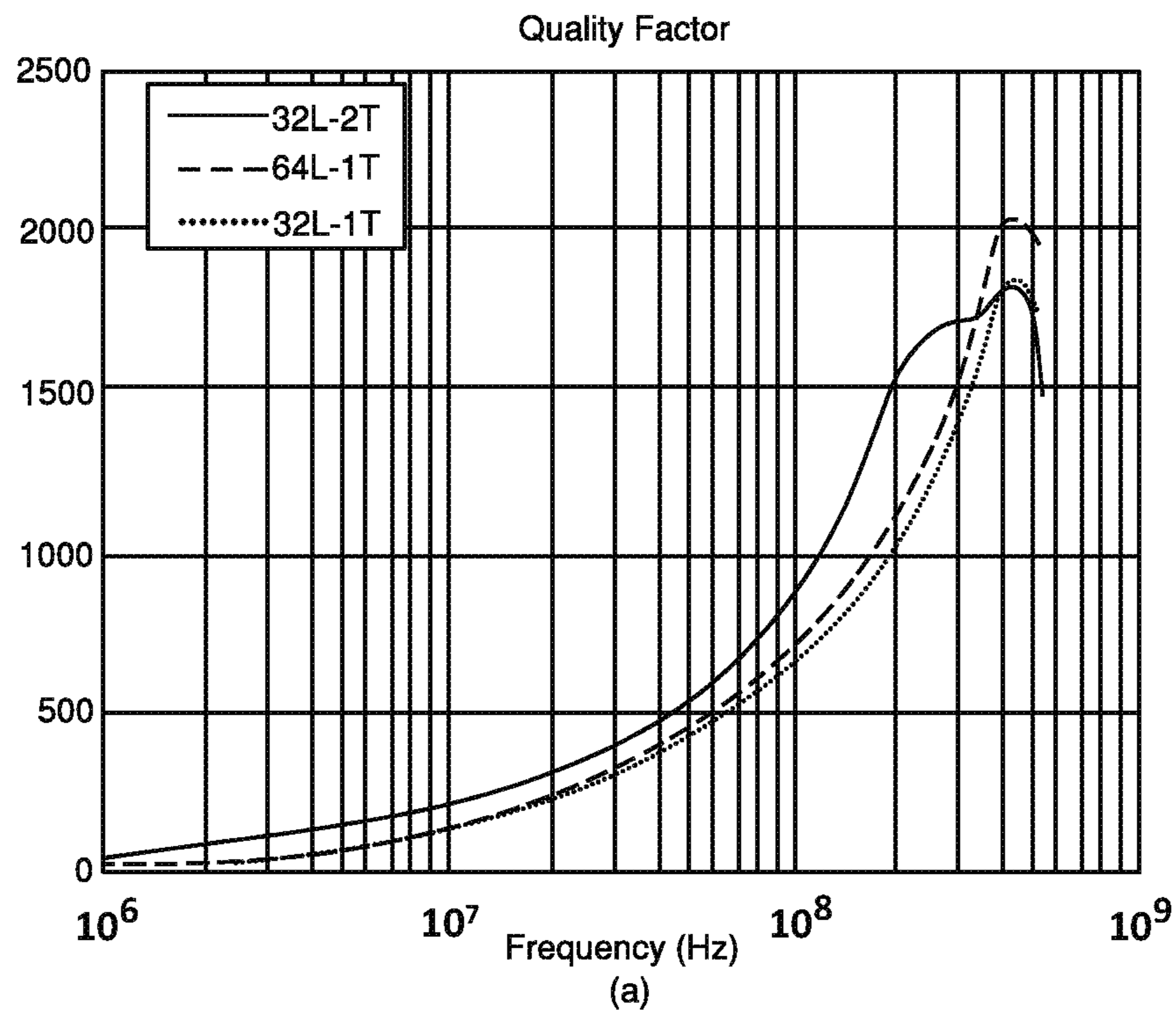
FIG. 11A
