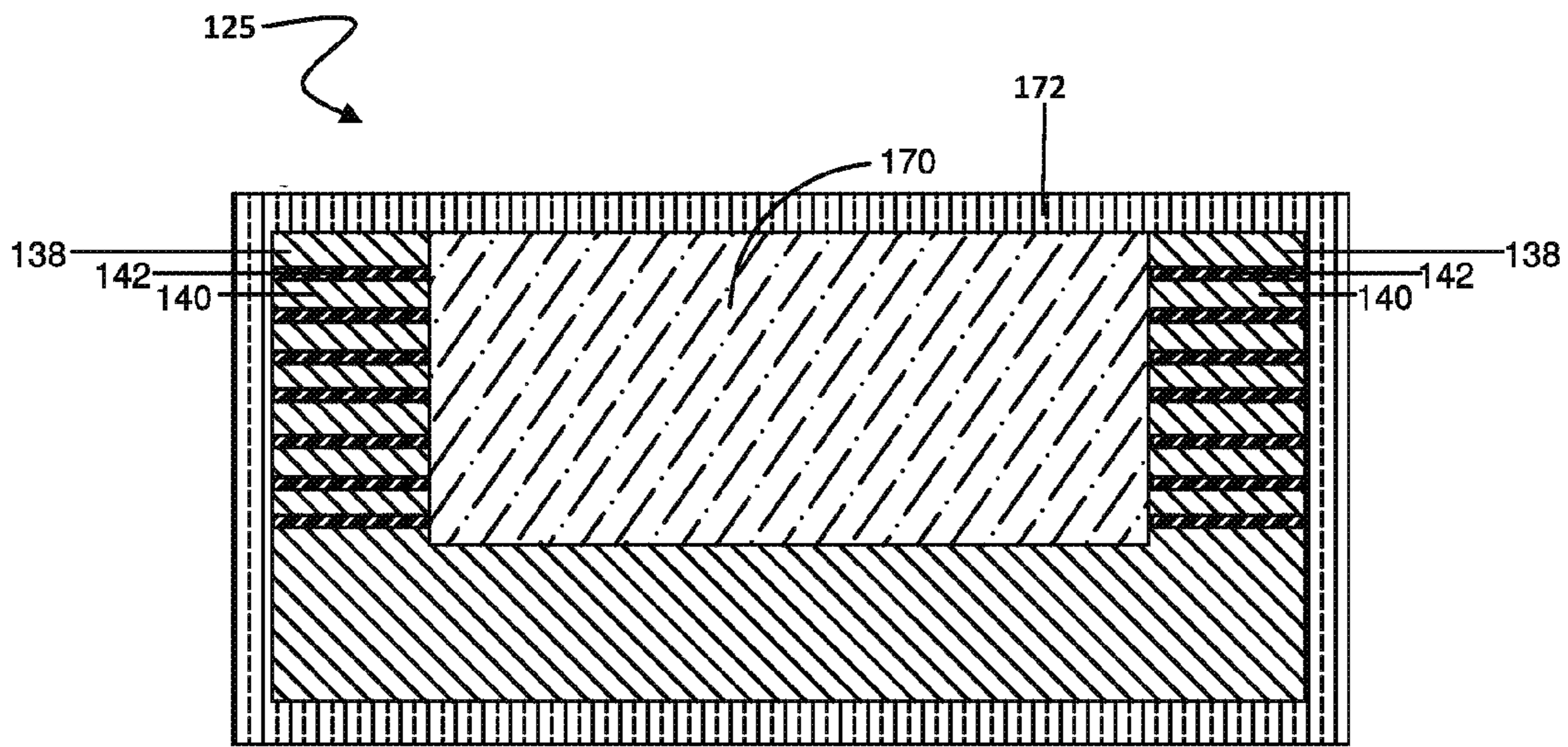
FIG. 13B
