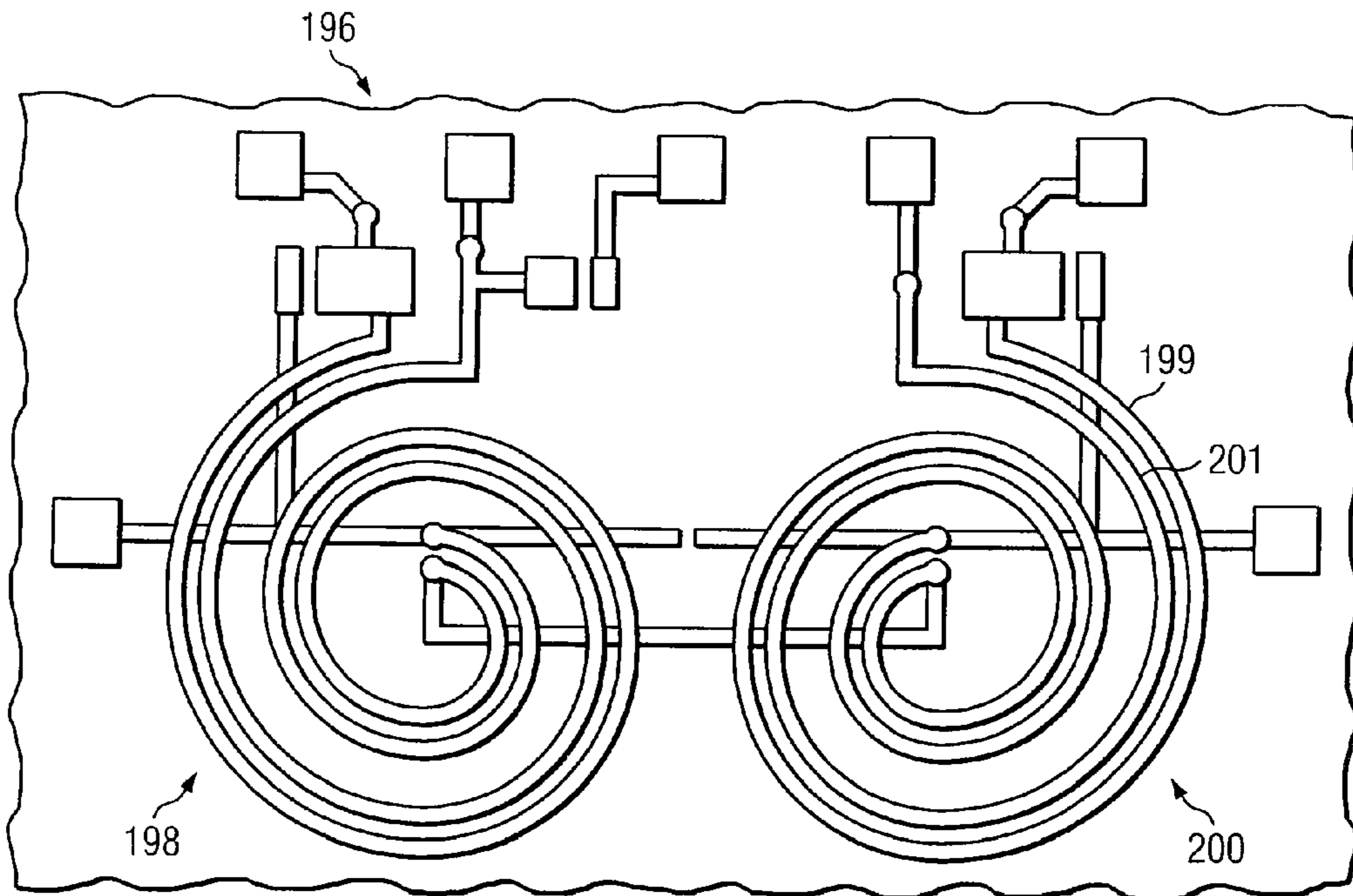
FIG. 7A
