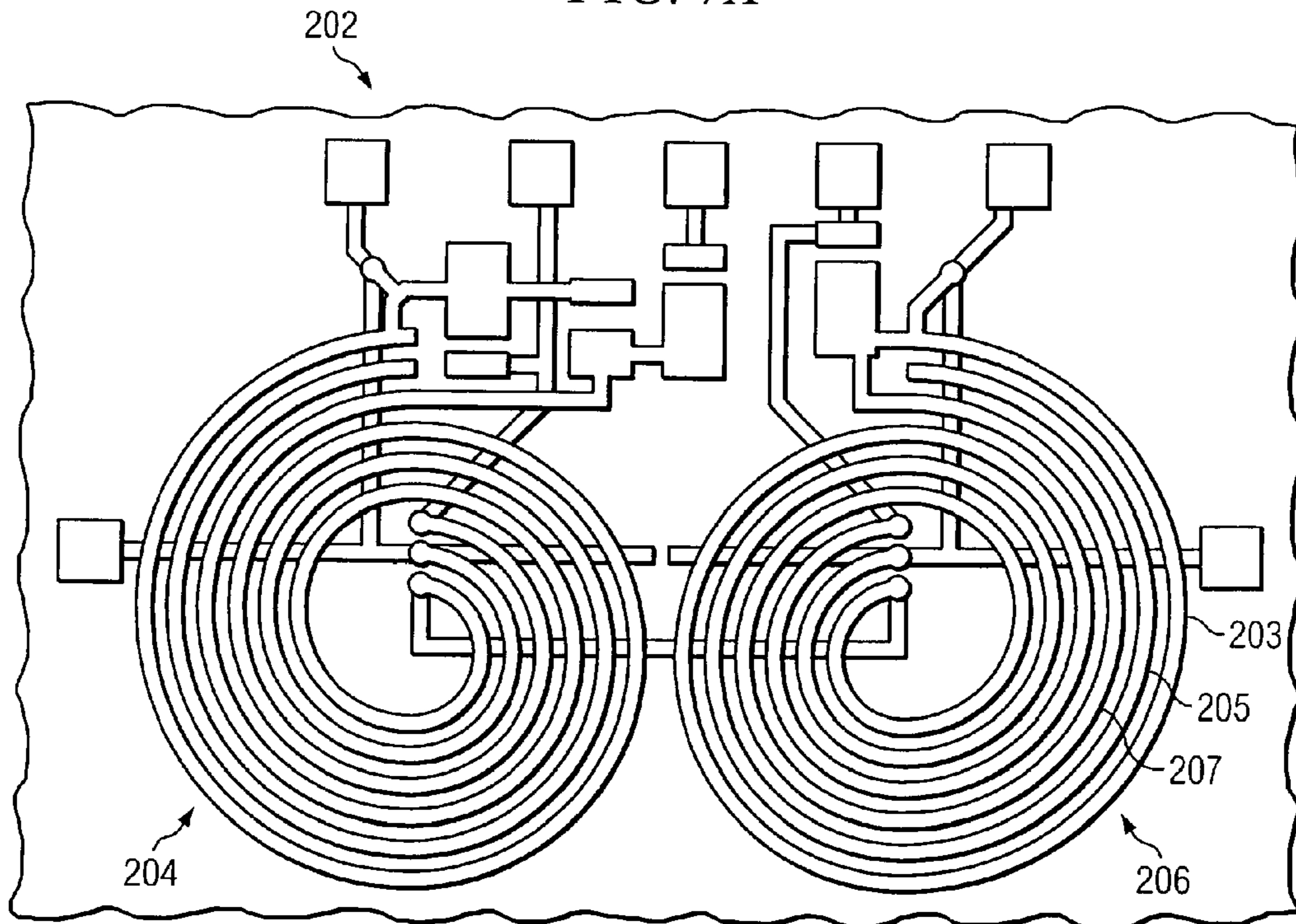
FIG. 7B
