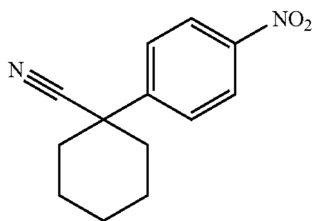
a) 1-(4-Nitro-phenyl)-cyclohexanecarbonitrile
