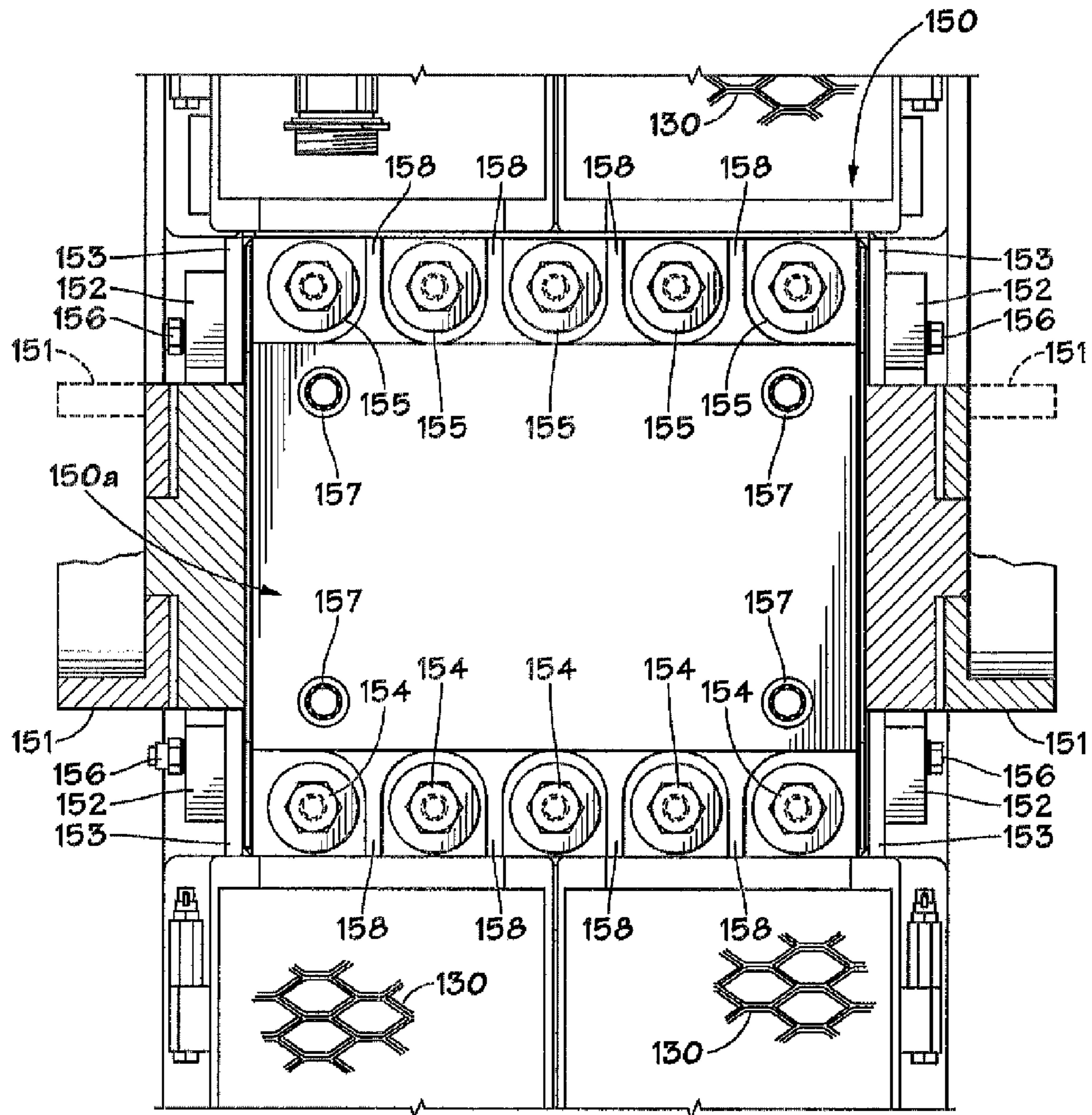
FIG. 2e
