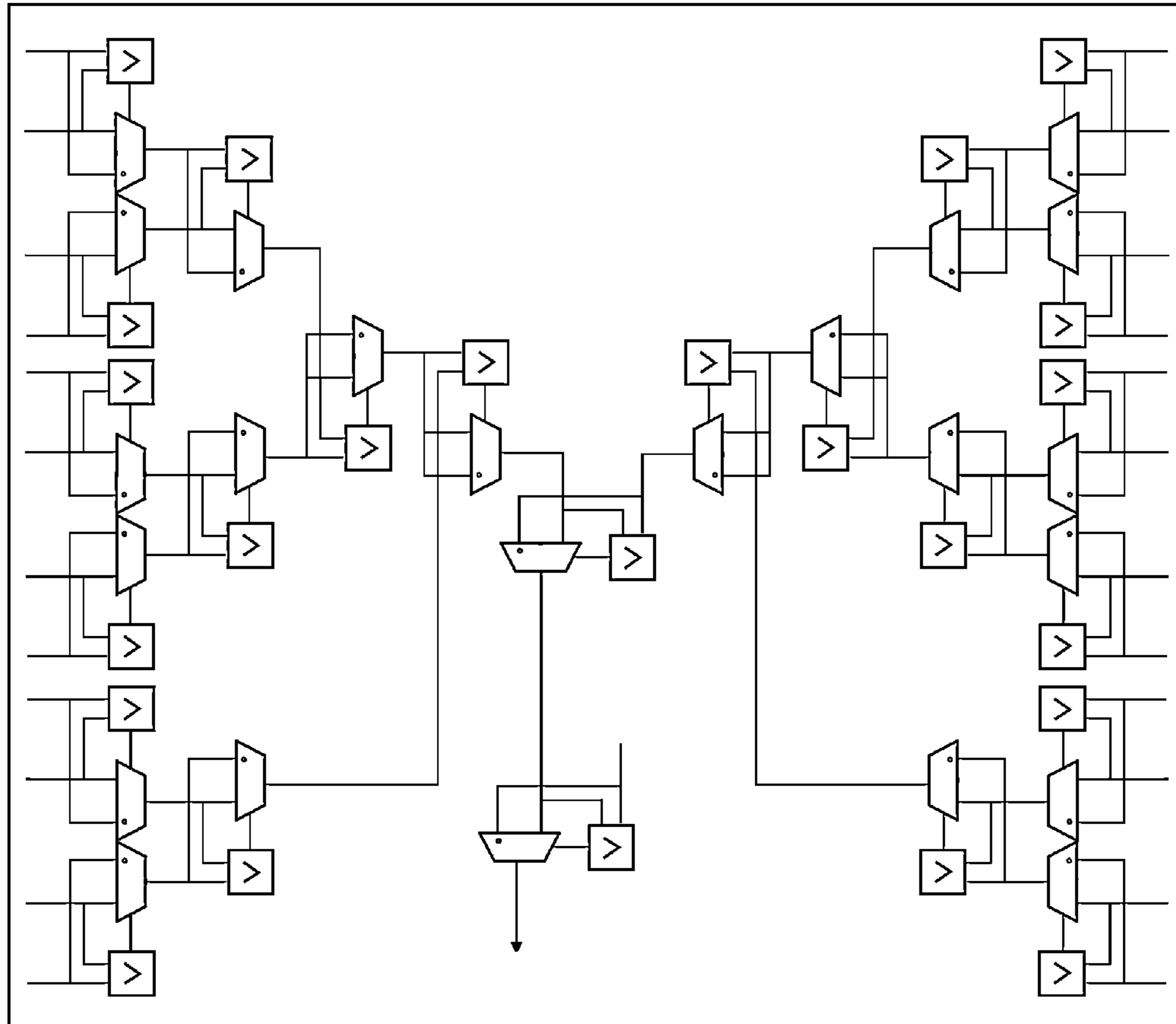
Minimize 25 Values
