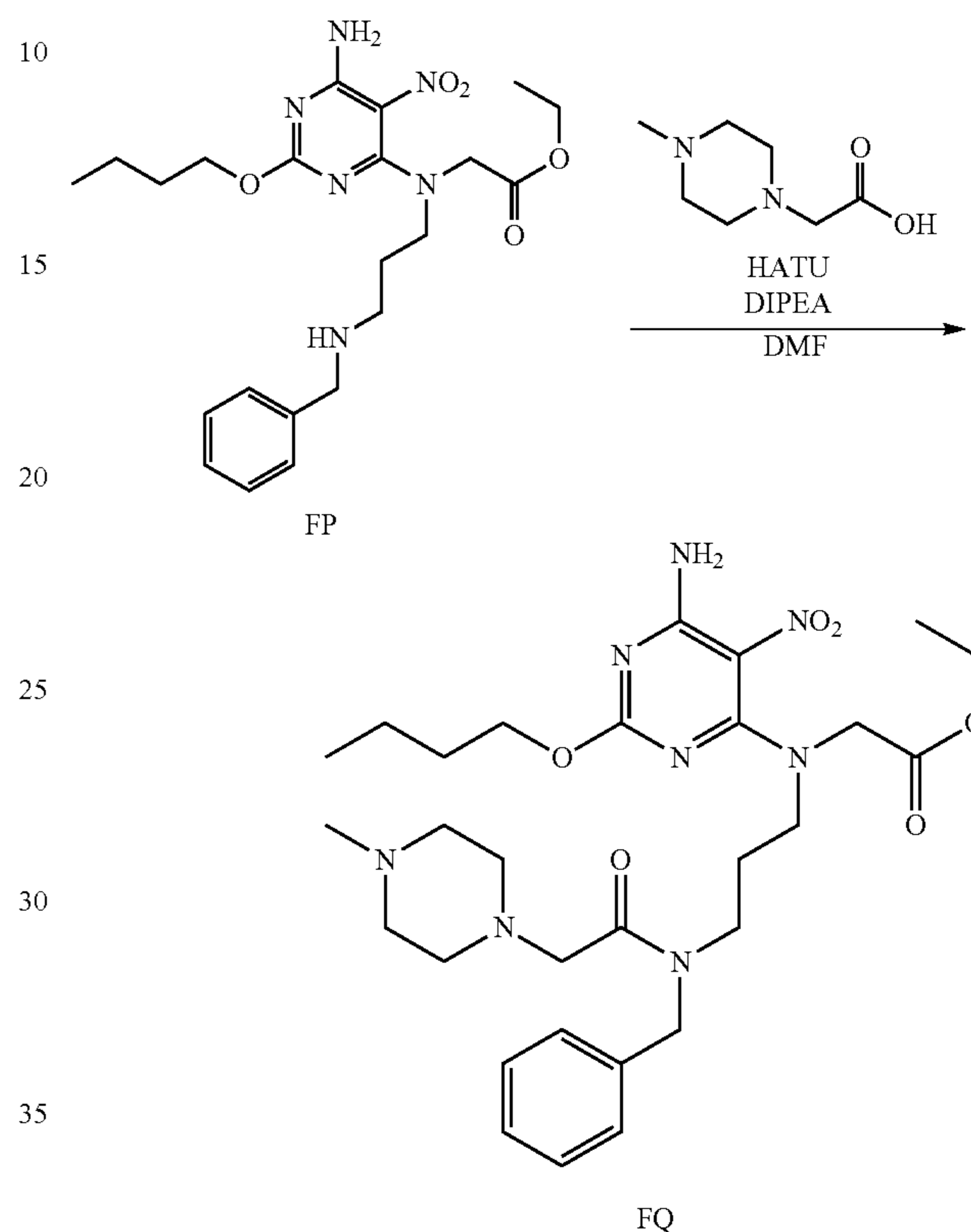
Scheme 107:
