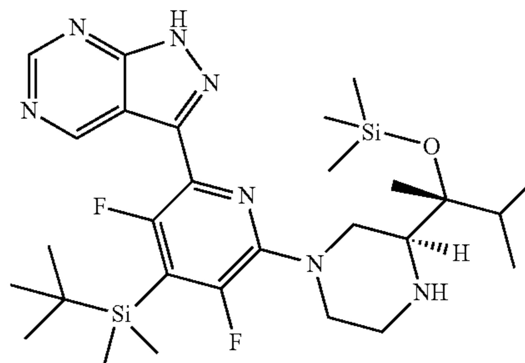
3-(4-(tert-butyl dimethylsilyl)-3,5-difluoro-6-((S)-3-((R)-3-methyl-2-((trimethylsilyl)oxy)butan-2-yl)piperazin-1-yl)pyridin-2-yl)-1H-pyrazolo[3,4-d]pyrimidine
