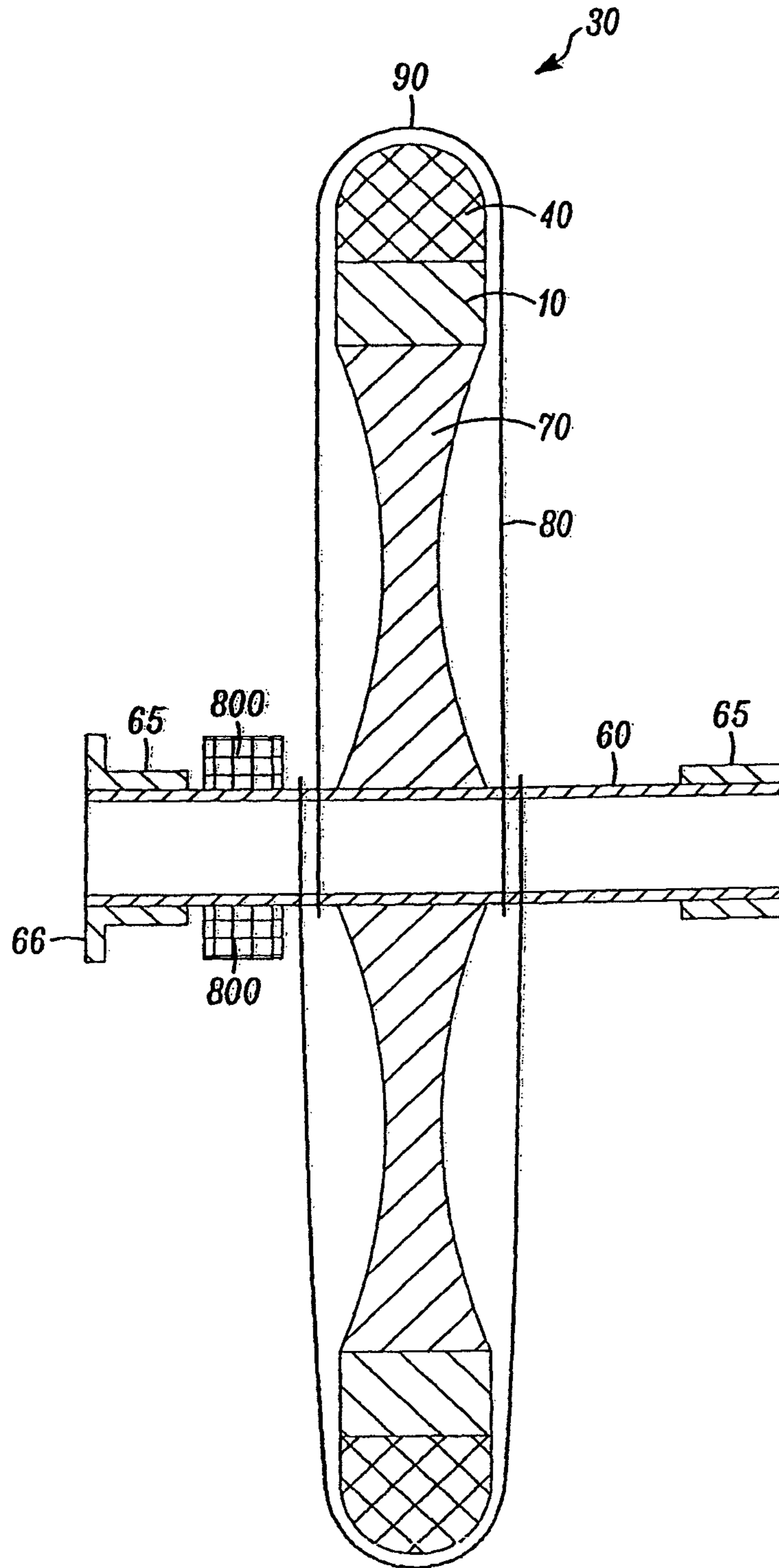
FIG. 14
