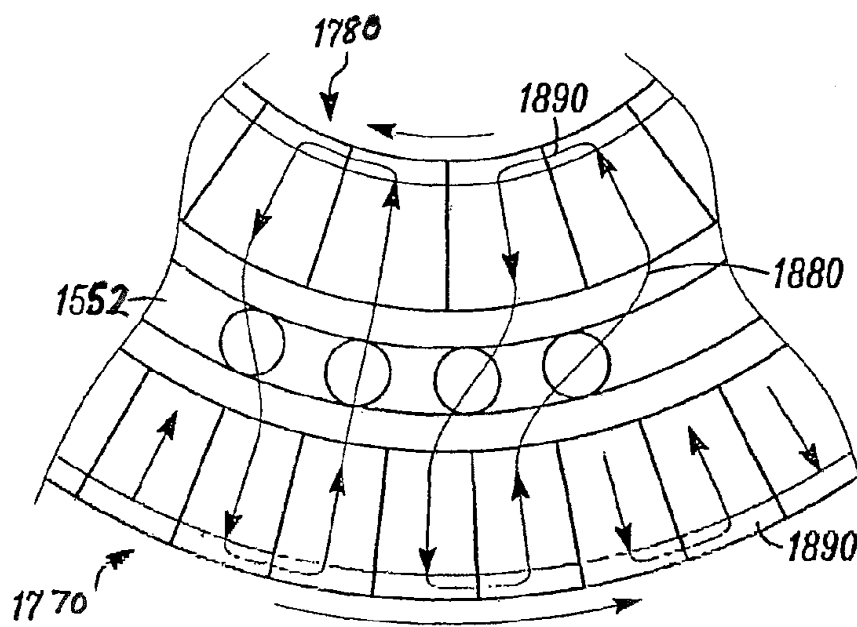
FIG. 18B
