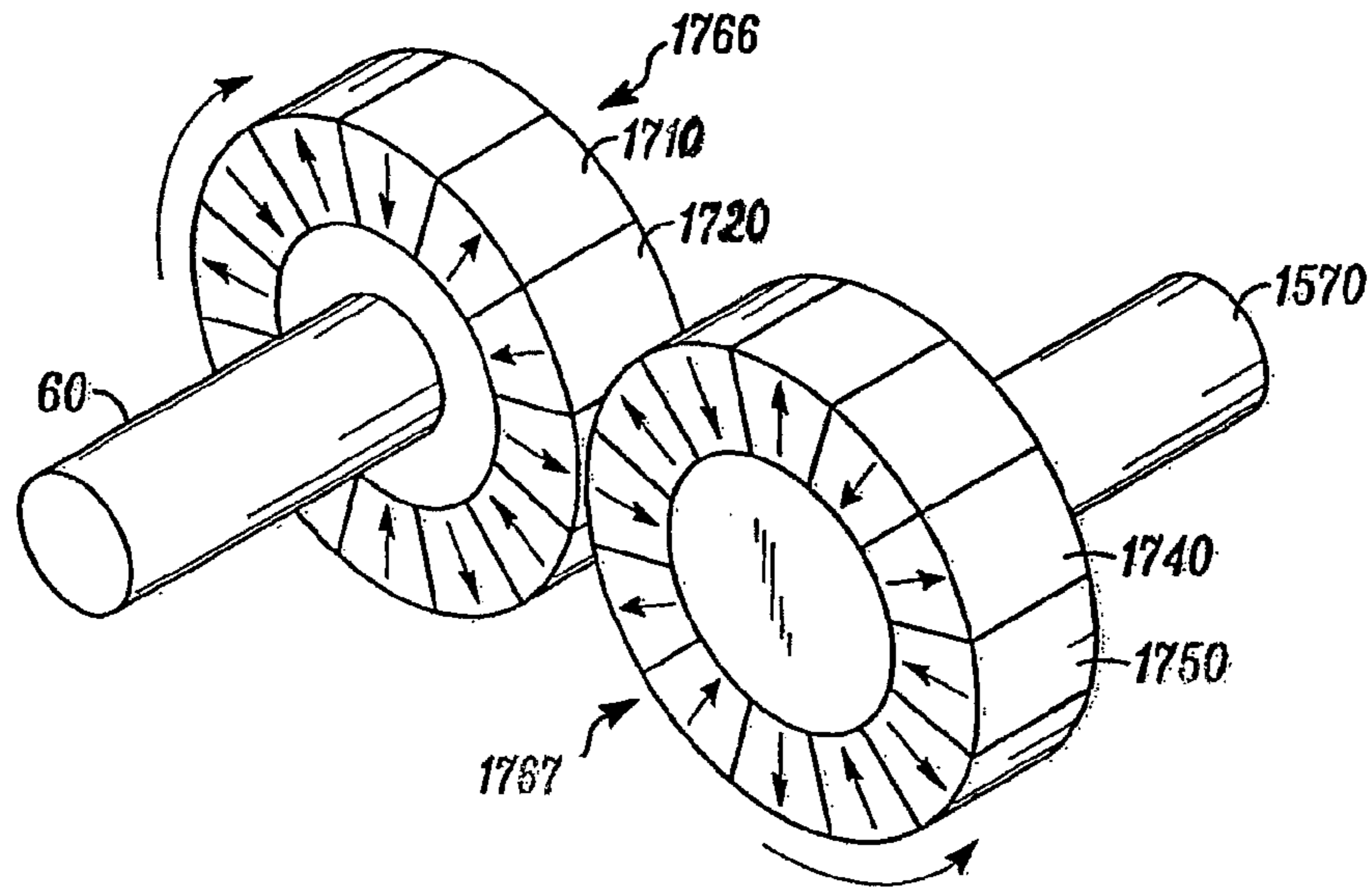
FIG. 17A
