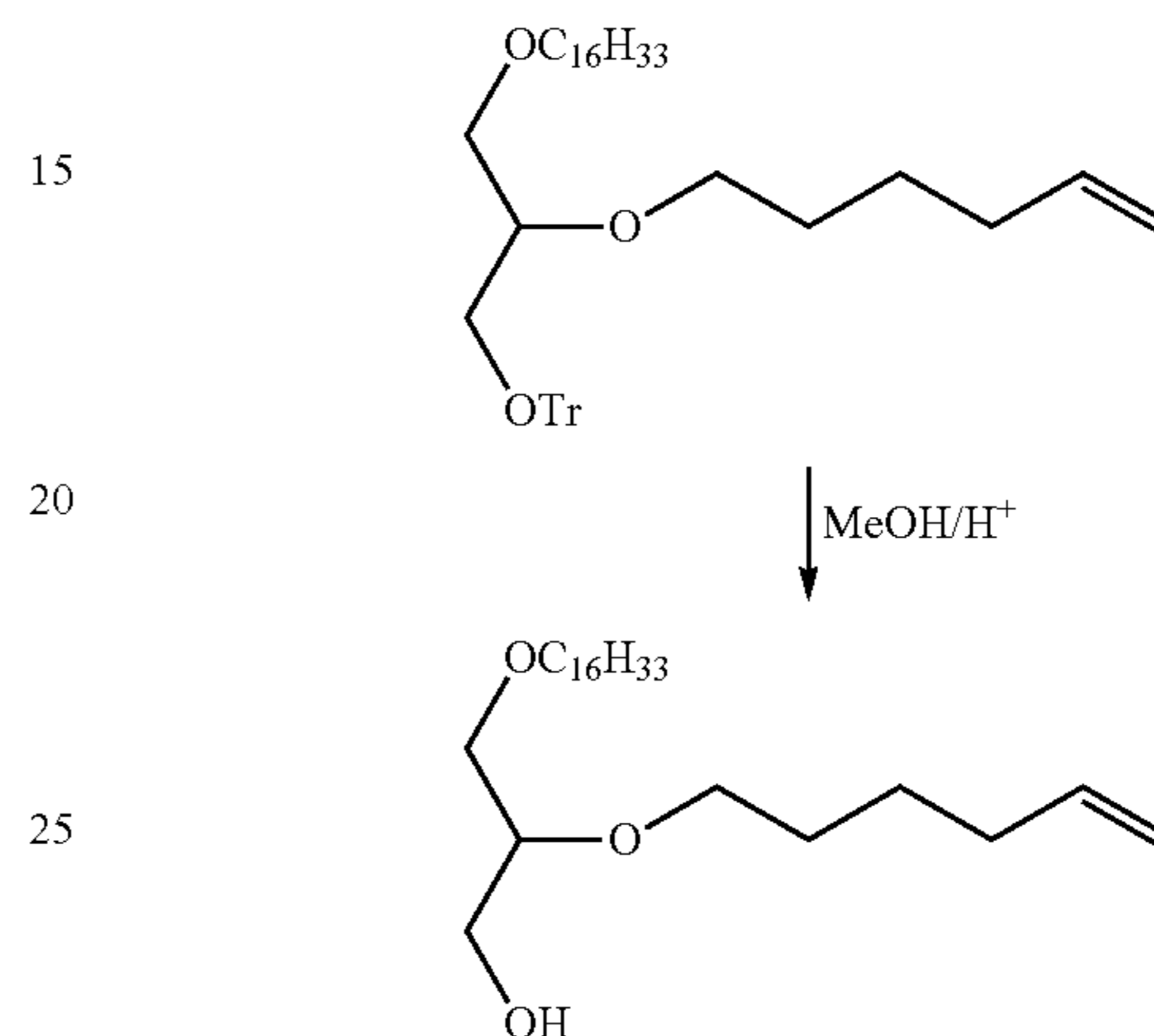
Scheme VI
