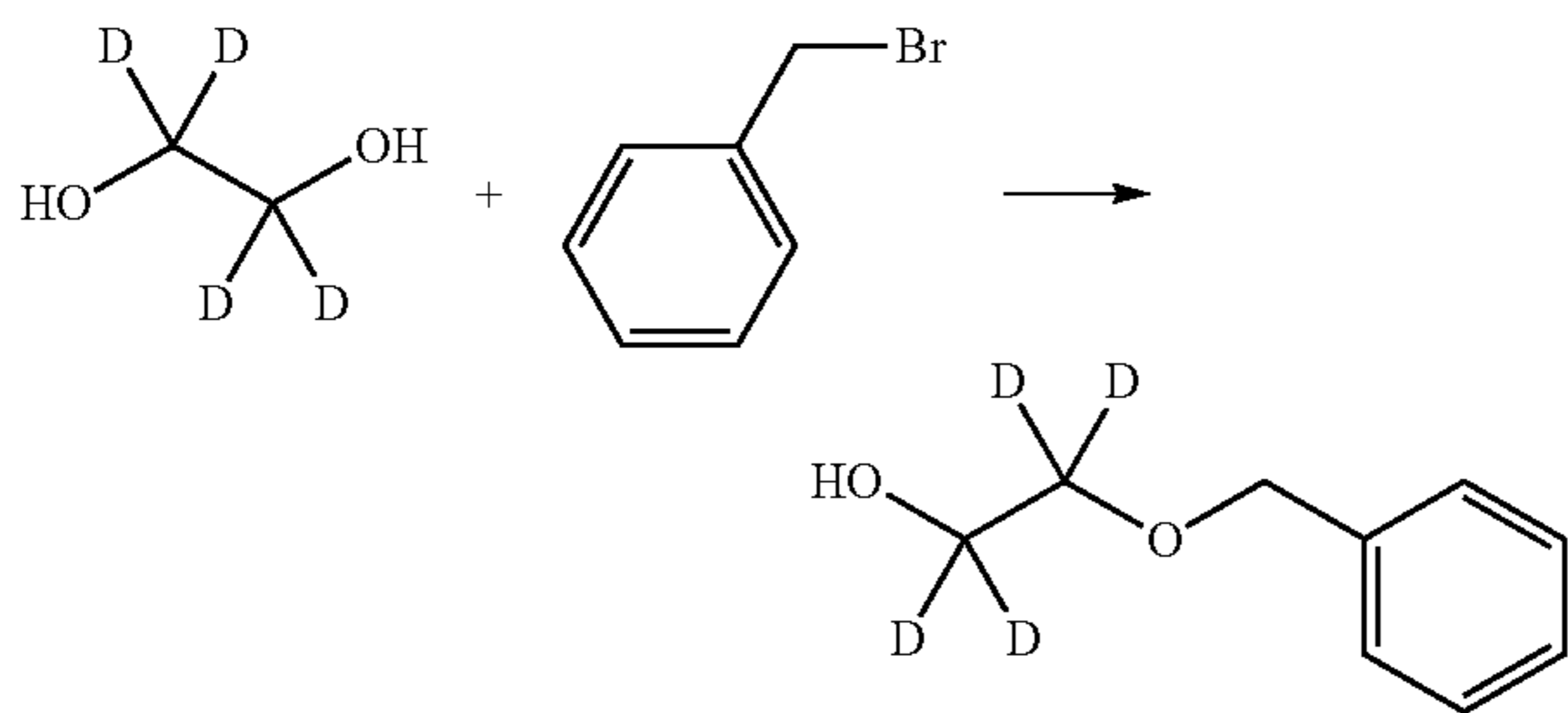
2-(Benzyloxy)-d 4 -ethanol
