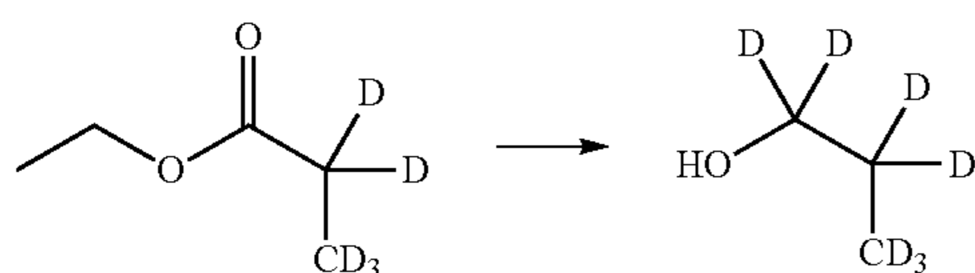
d 5 -Propan-1-ol
