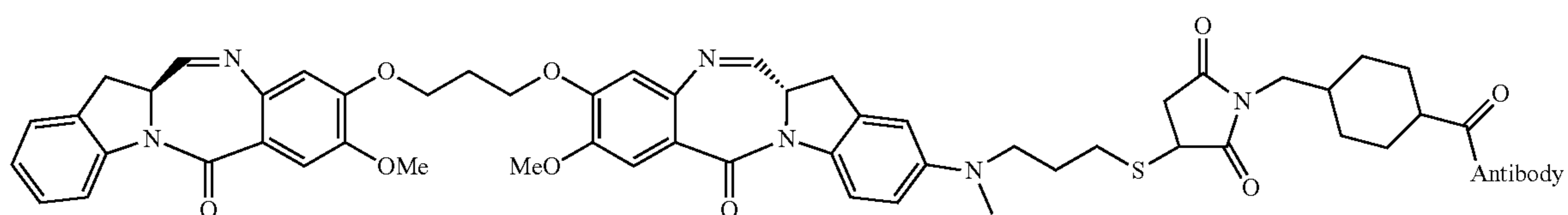
Dimer 7
