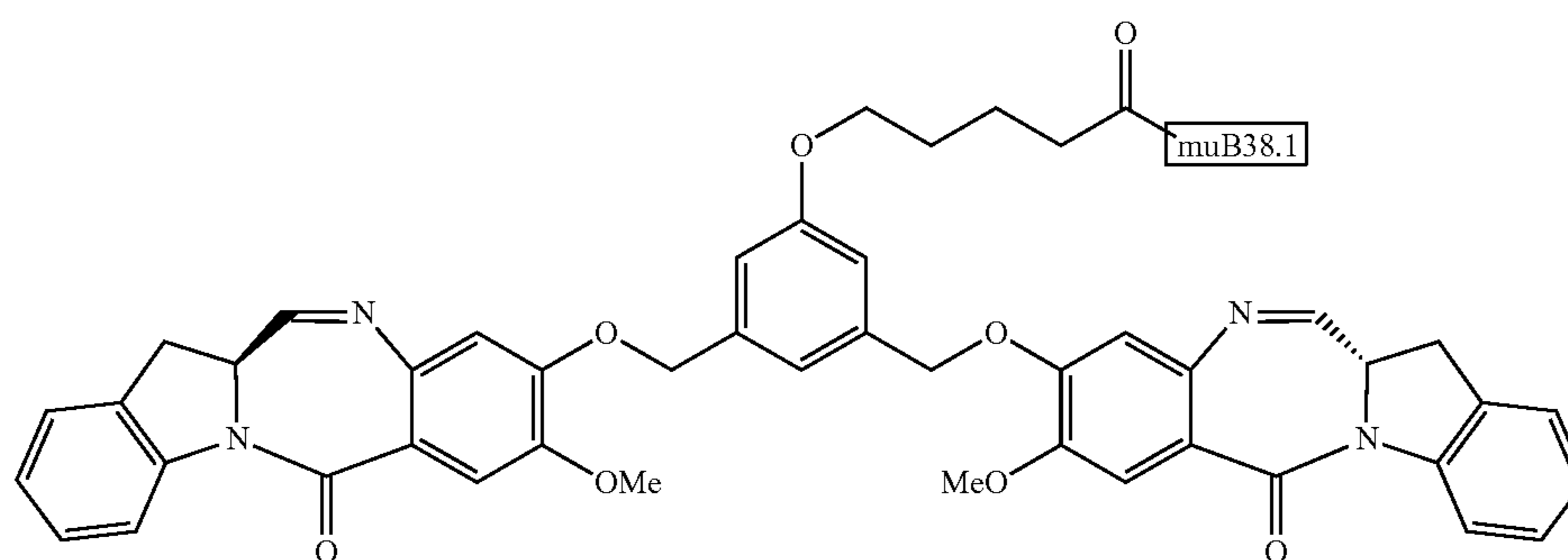
B38.1-IGN-03
