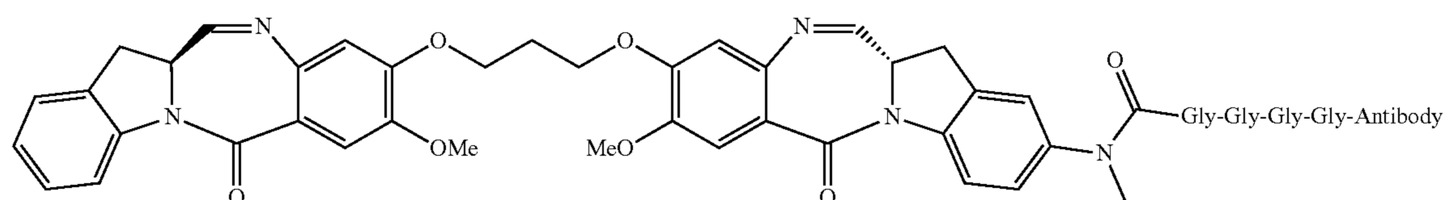
Dimer 5
