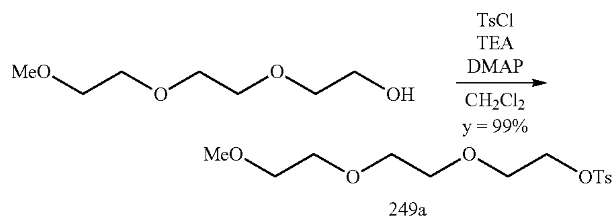
2-(2-(2-methoxyethoxy)ethoxy)ethyl 4-methylbenzenesulfonate
