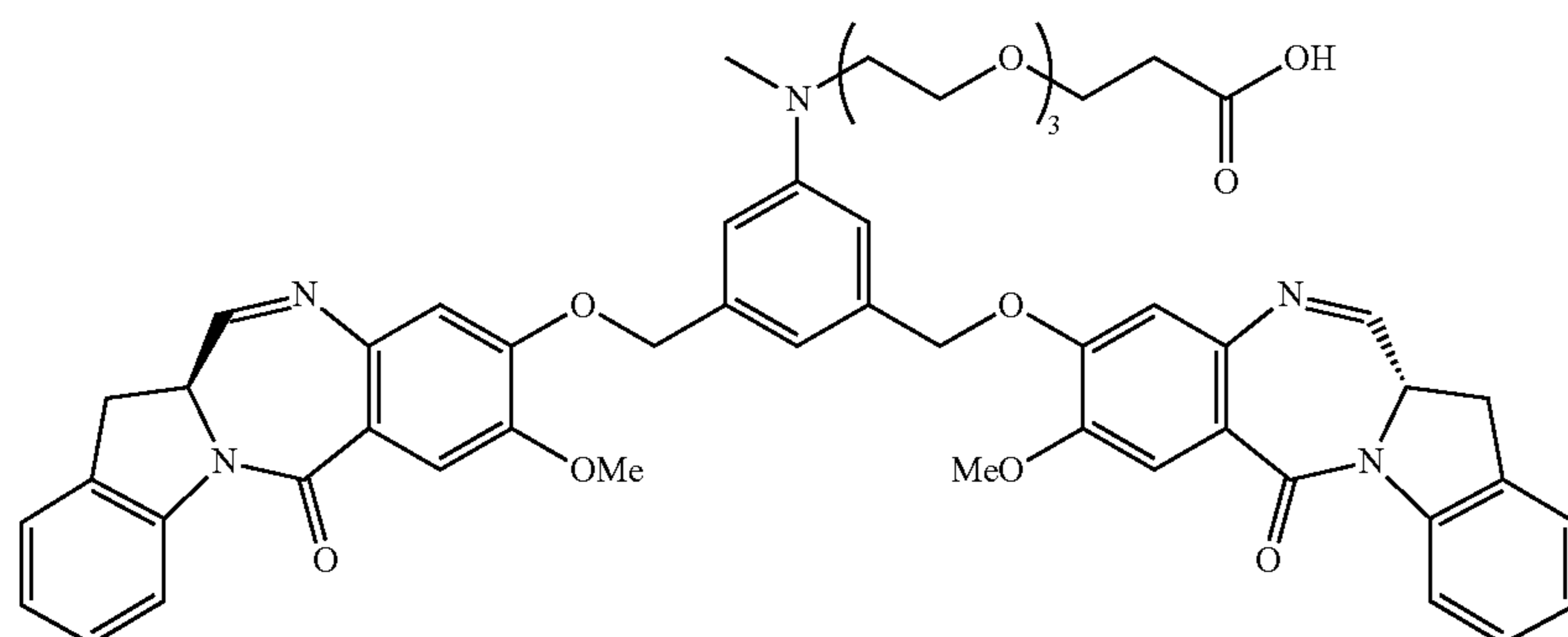
264d
