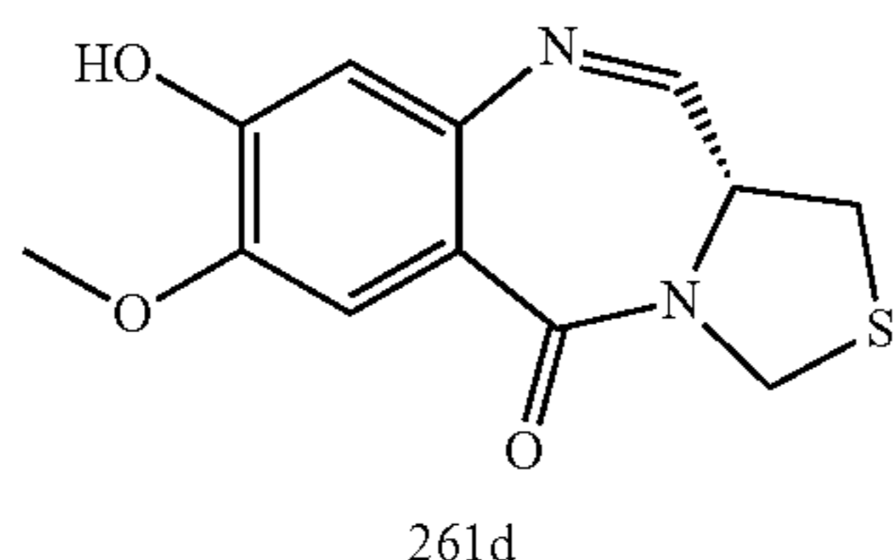
261d
