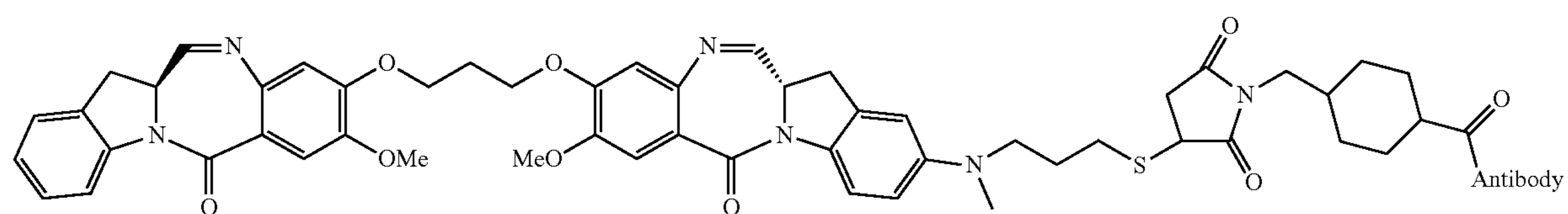
Dimer 7
