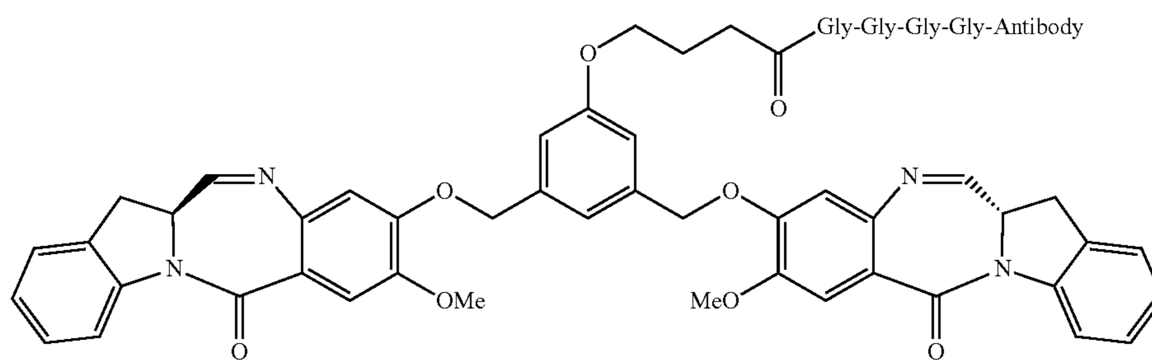
Dimer 1
