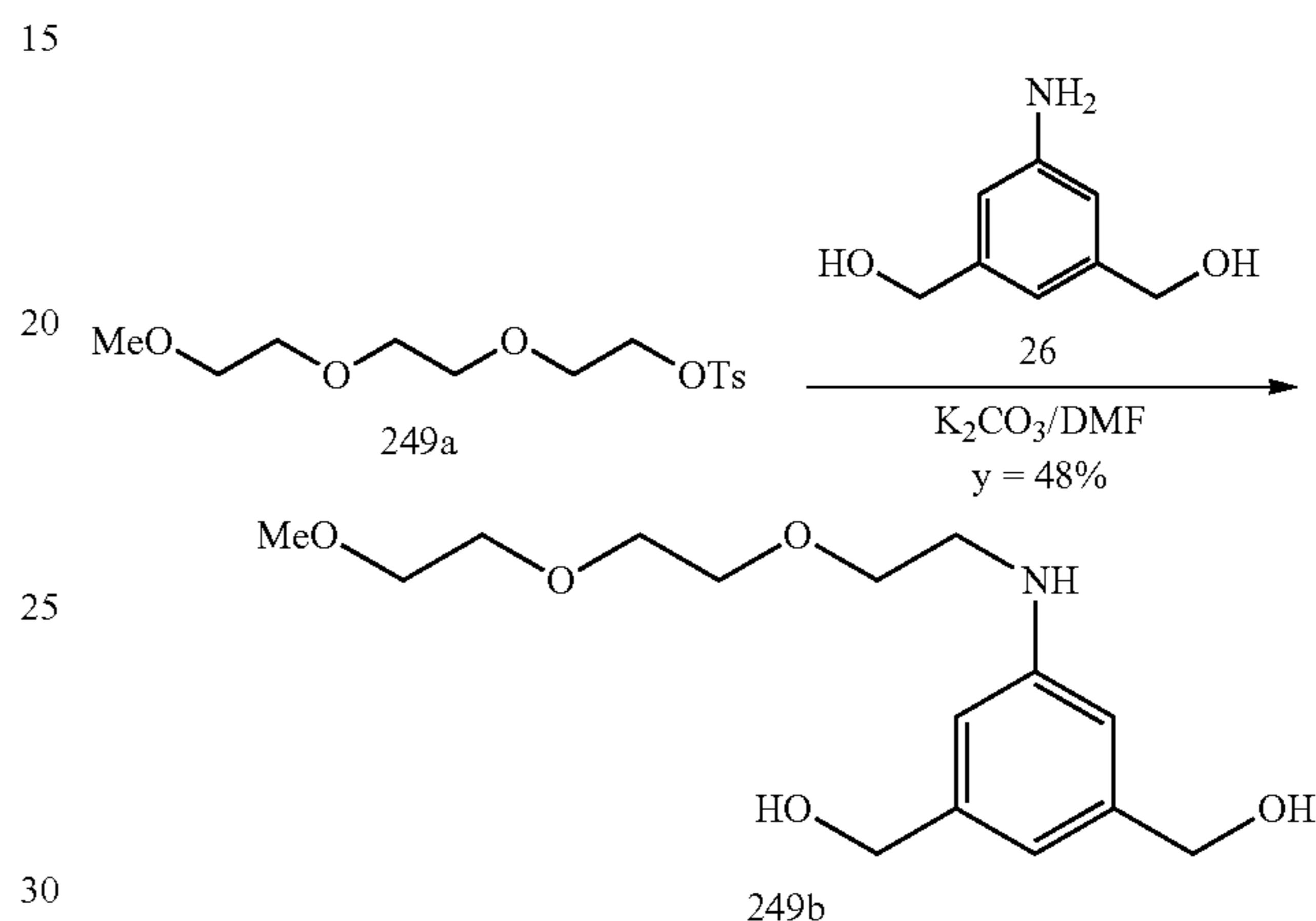
(5-(2-(2-(2-methoxyethoxy)ethoxy)ethylamino)-1,3-phenylene)dimethanol
