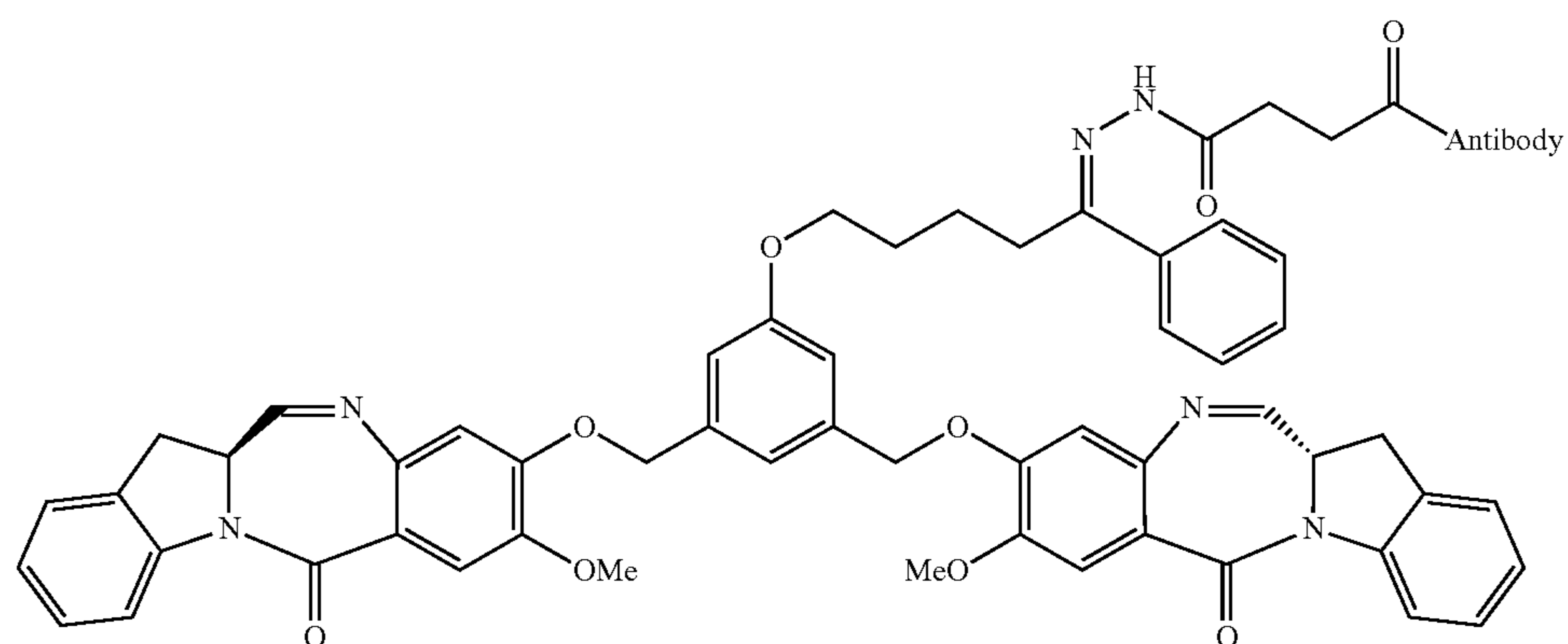
Dimer 4
