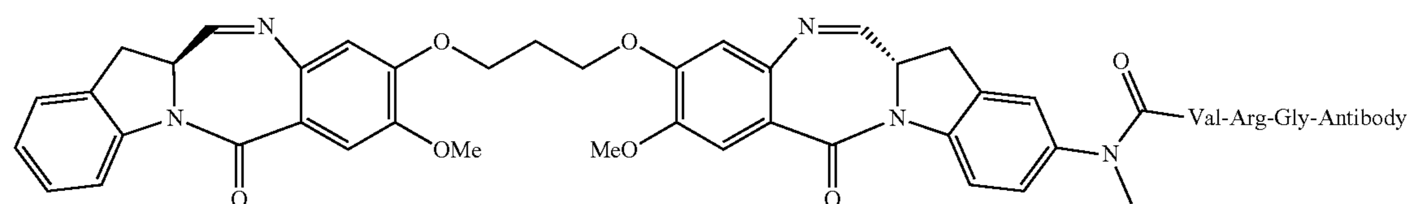
Dimer 6
