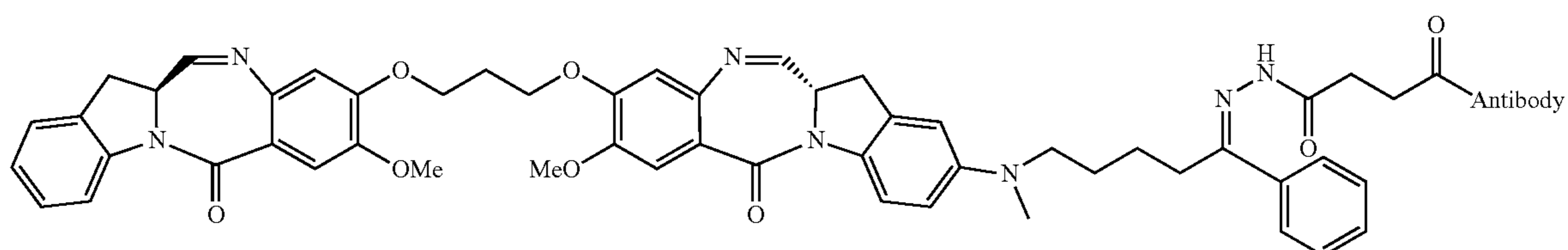
Dimer 8
