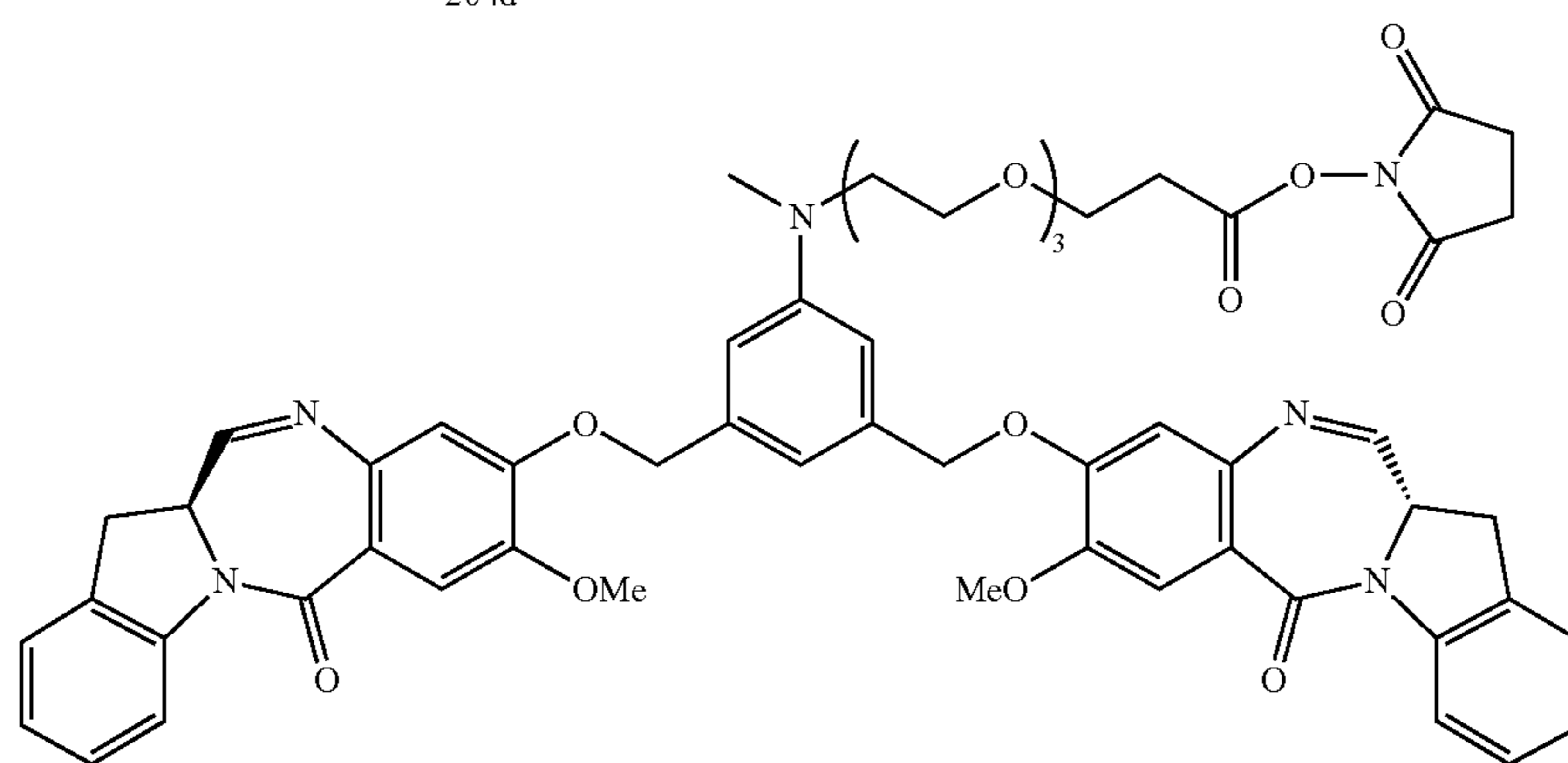
264e
