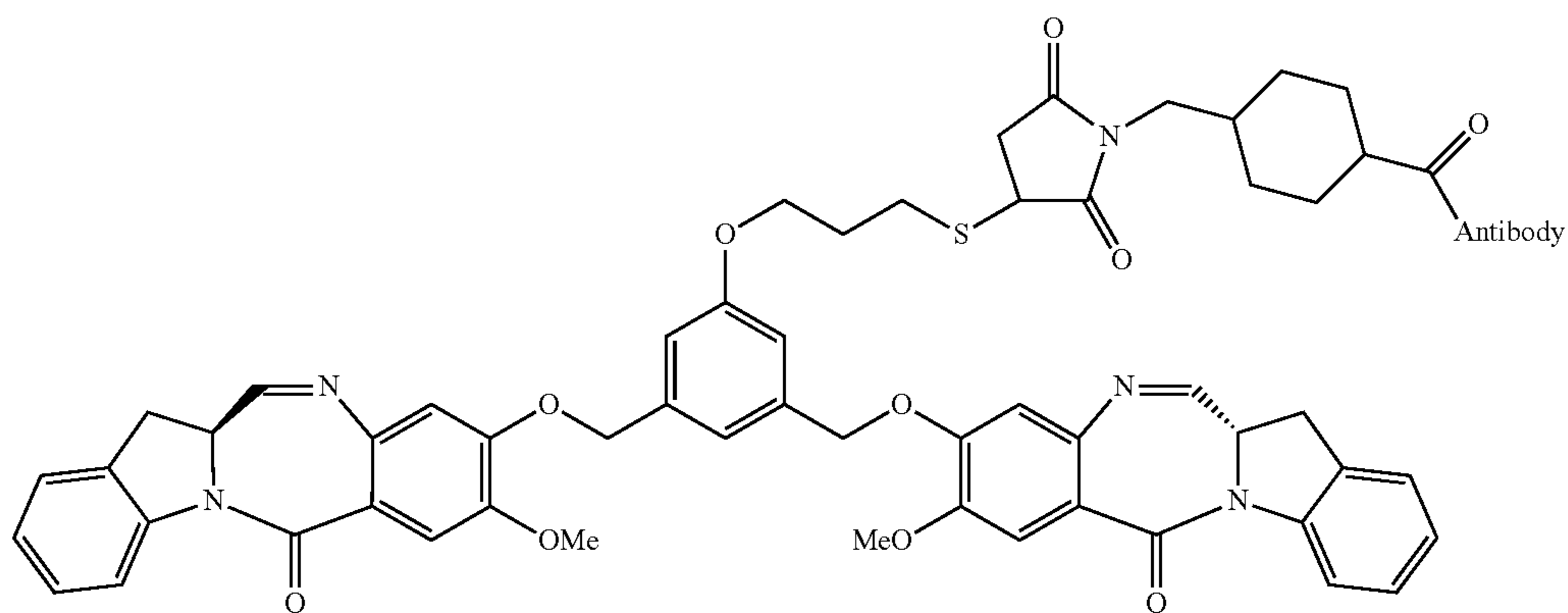
Dimer 3
