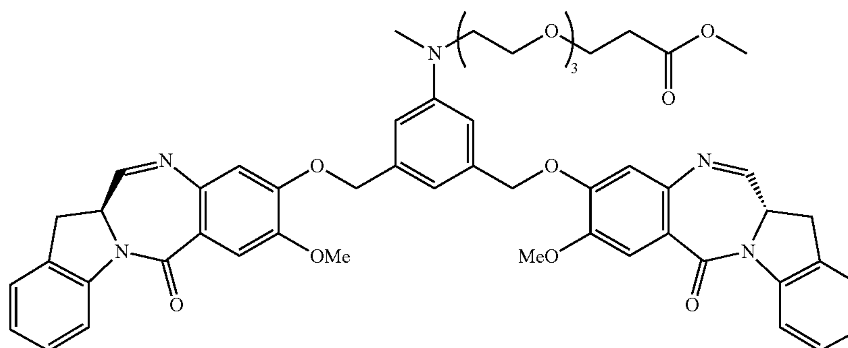
264c
