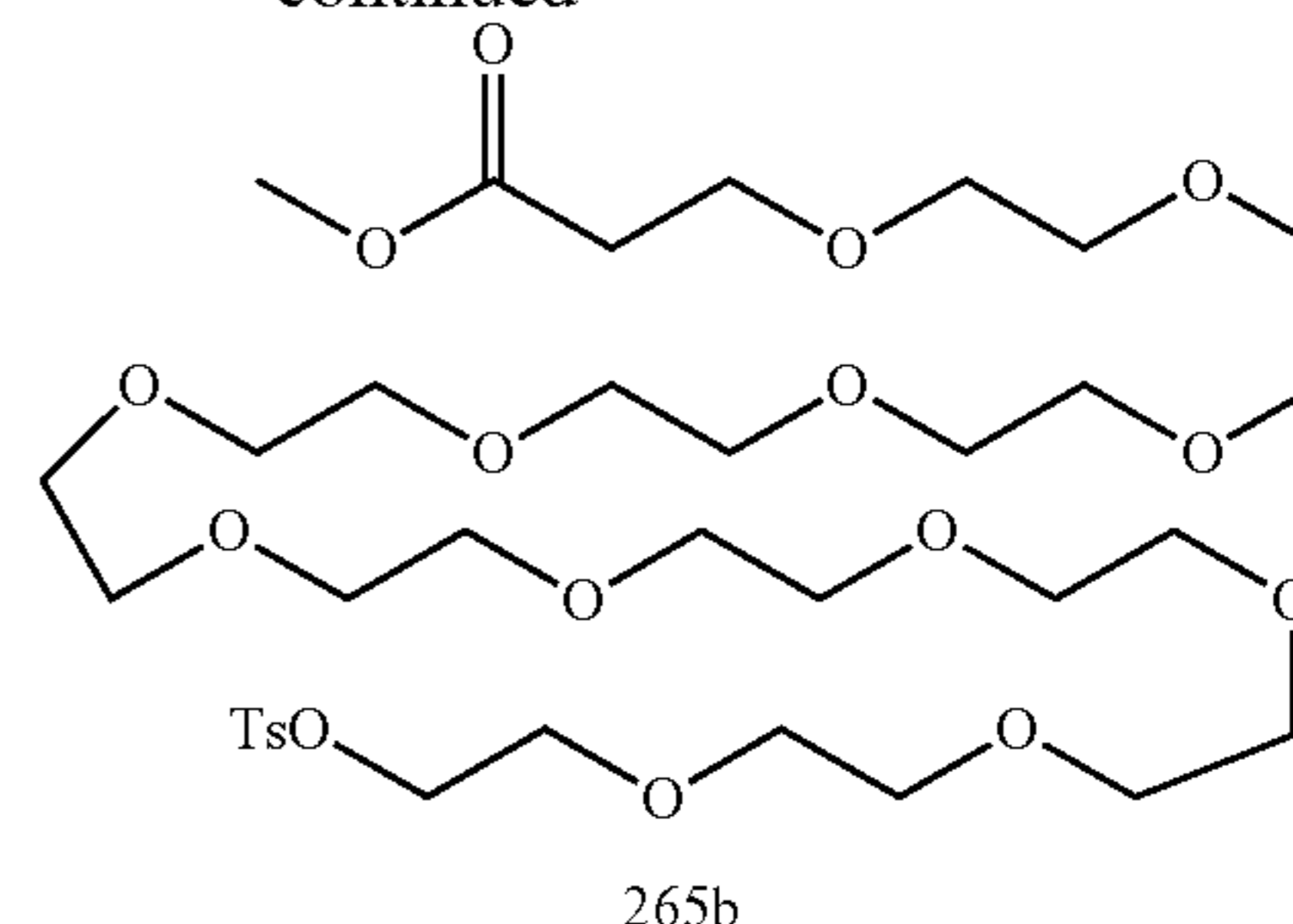
265b
