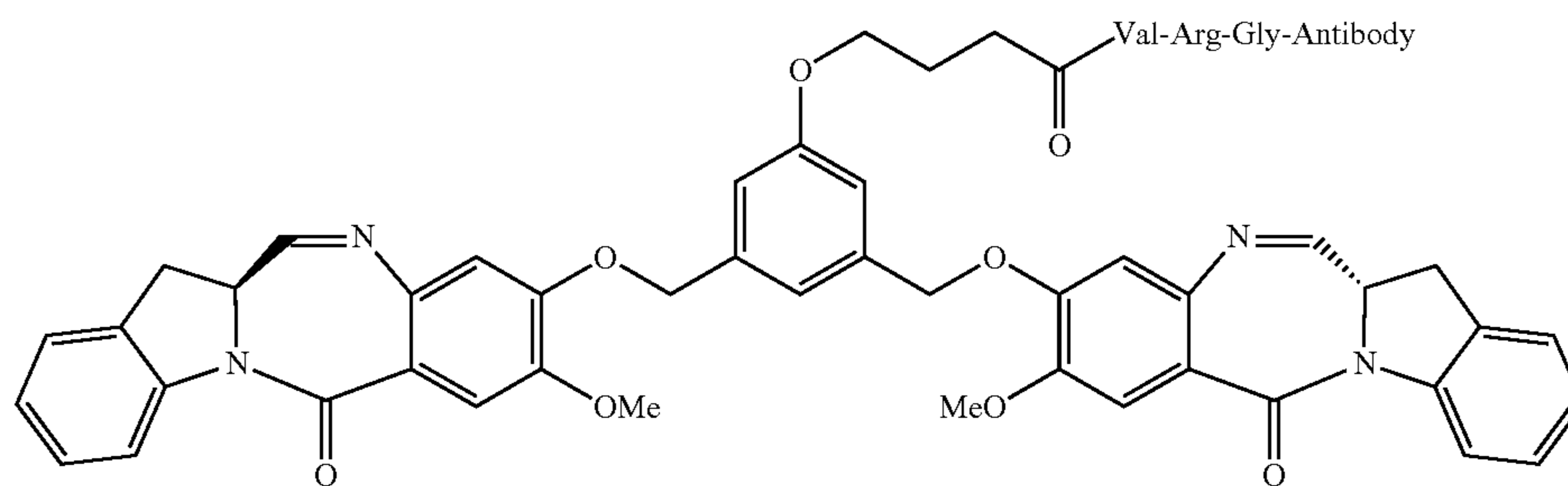
Dimer 2
