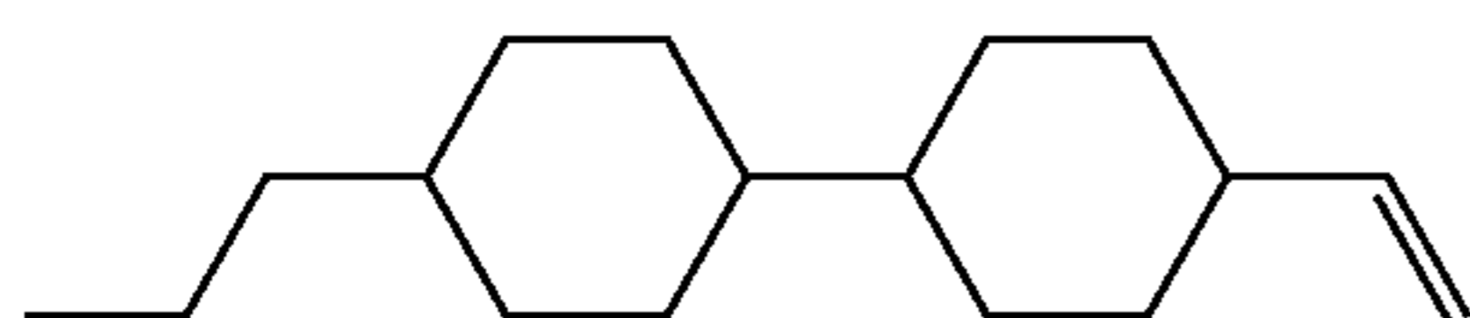
Example 4. V2-HHB-1
