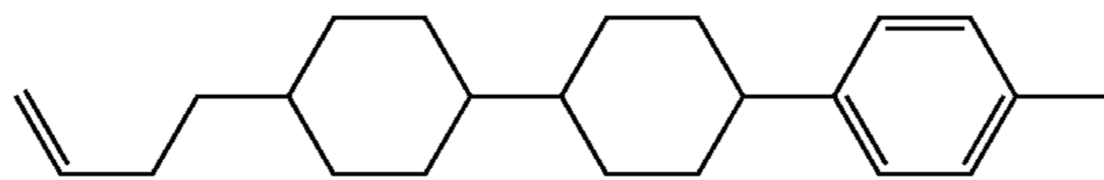
Example 4. V2-HHB-1
