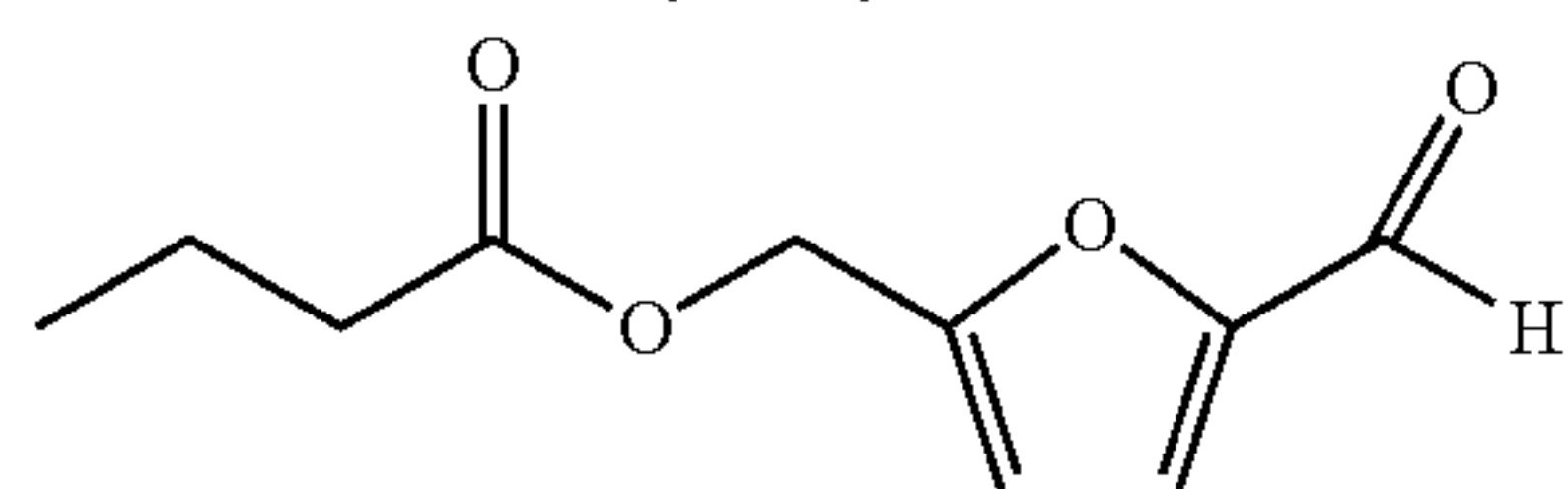
5-butyroxymethylfurfural
