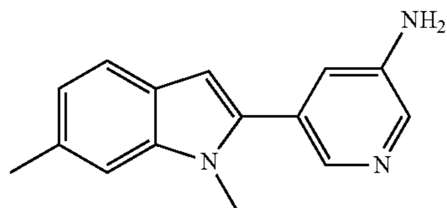
(d) 5-(1,6-Dimethyl-1H-indol-2-yl)-pyridin-3-ylamine
