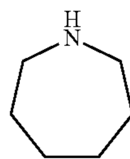
azepane (azepanyl)
