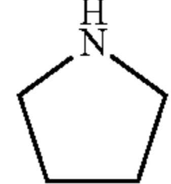
pyrrolidine (pyrrolidinyl)
