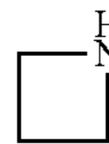
azetidine (azetidiny)
