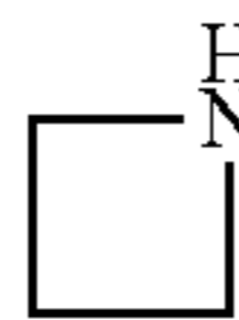
azetidine (azetidyl)
