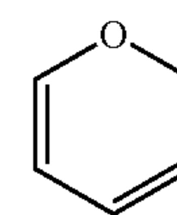
2H-pyran (2H-pyranlyl)
