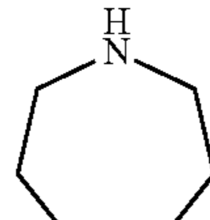
azepane (azepanyl)
