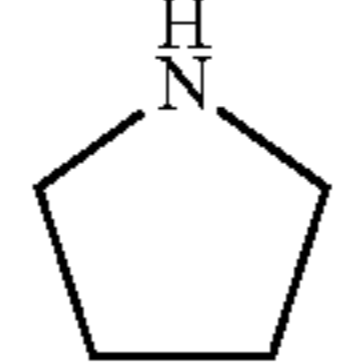
pyrrolidine (pyrrolidinyl)
