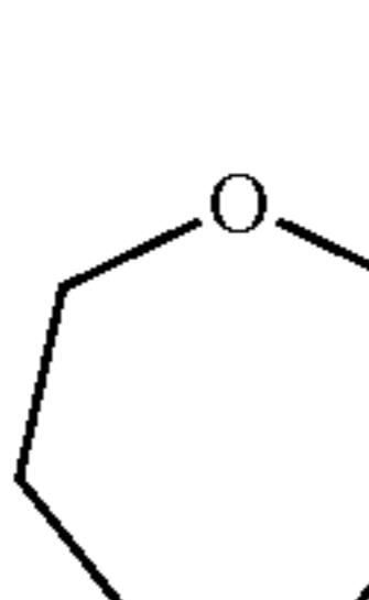
oxepane (oxepanyl)
