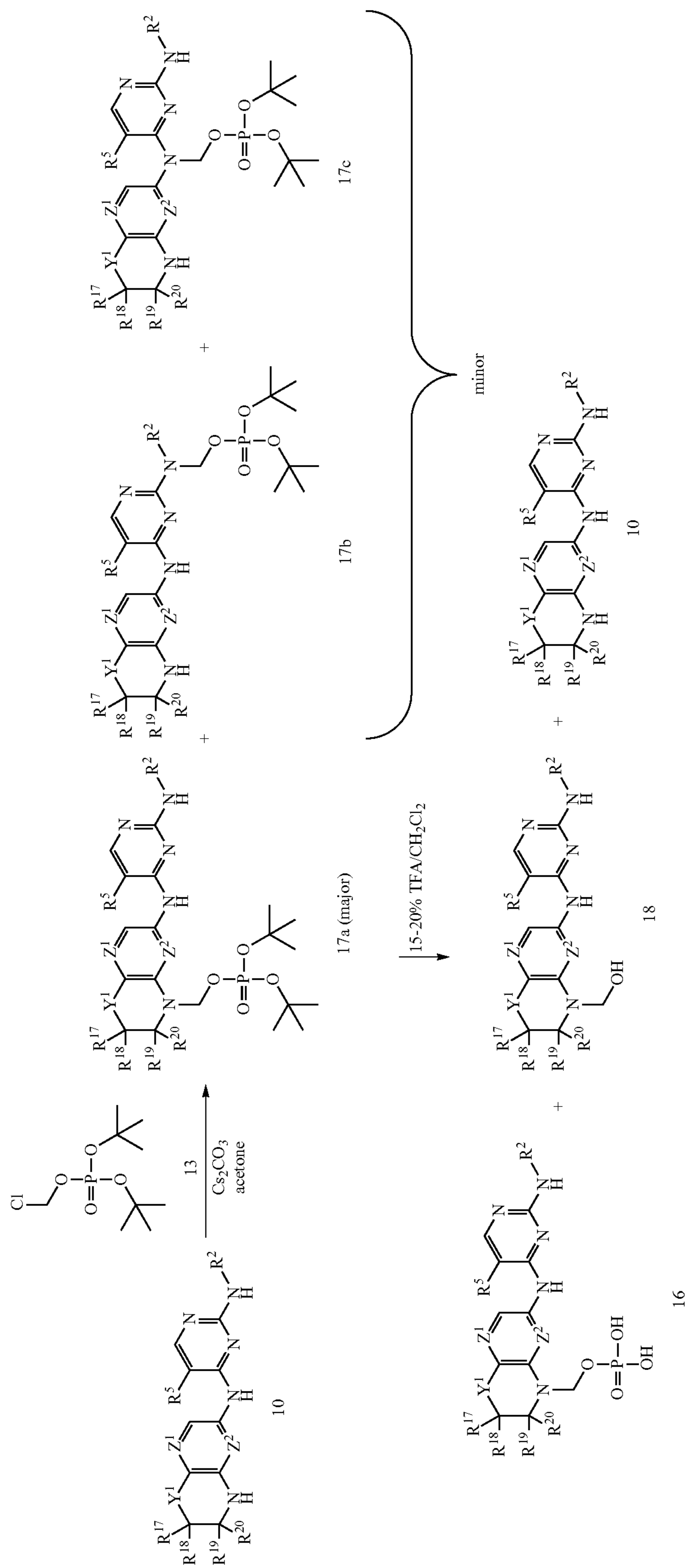
Scheme (IV)
