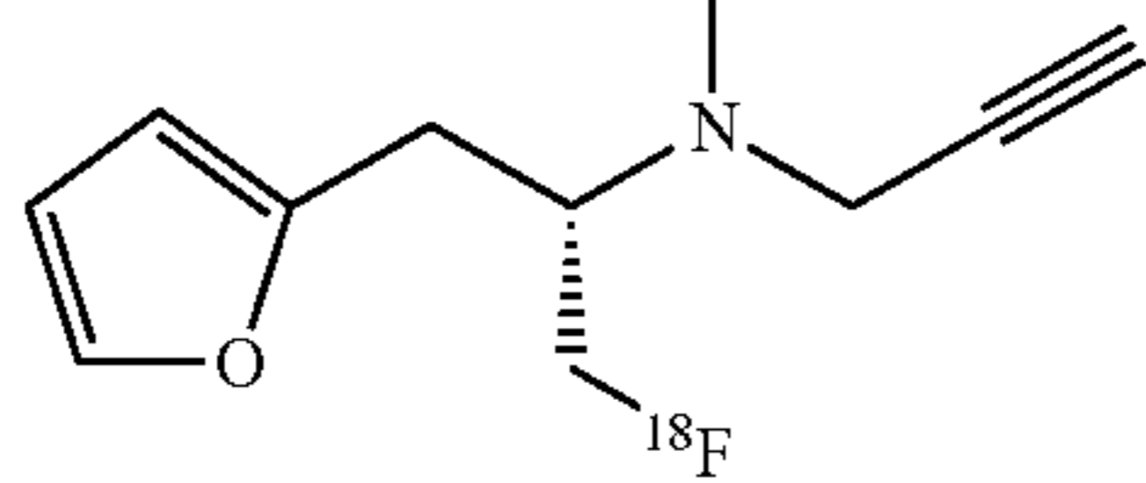
N-[(2S)-1-( 18 F)fluoro-3-(furan-2-yl)propan-2-yl]-N-methylprop-2-yn-1-amine
