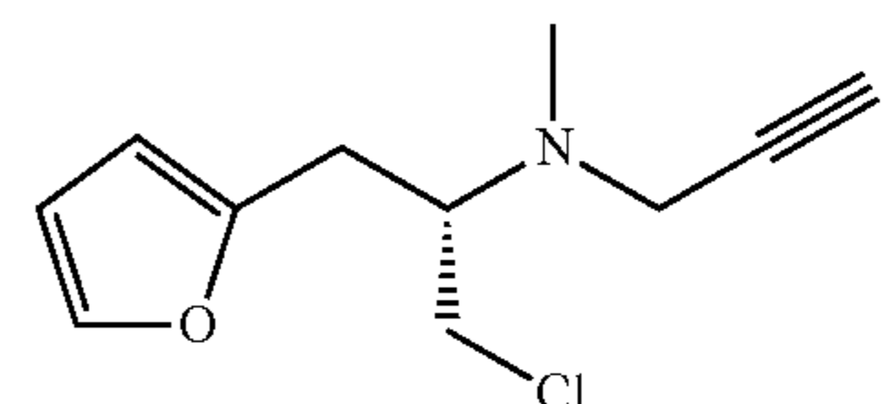
N-[(2S)-1-chloro-3-(furan-2-yl)propan-2-yl]-N-methylprop-2-yn-1-amine
