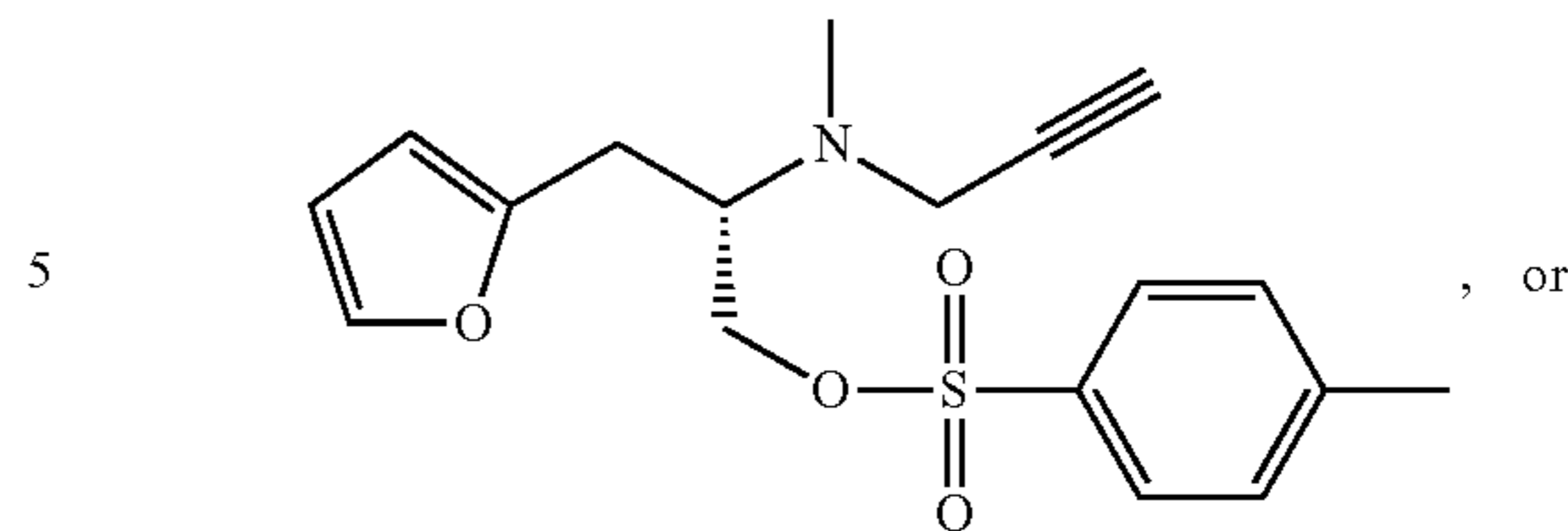
(2S)-3-(furan-2-yl)-2-[methyl(prop-2-yn-1-yl)amino]propyl 4-methylbenzenesulfonate
