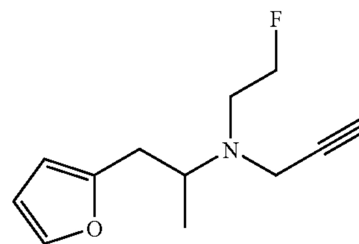
(2-Fluoro-ethyl)-(2-furan-2-yl-1-methyl-ethyl)-prop-2-ynyl-amine
