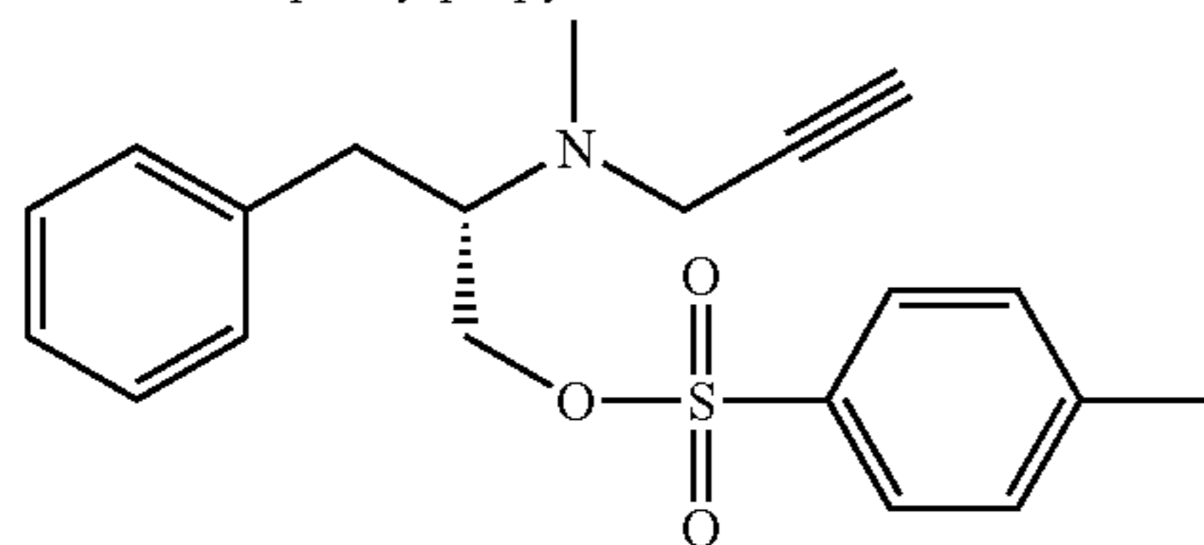
(2S)-2-[methyl(prop-2-yn-1-yl)amino]-3-phenylpropyl 4-methylbenzenesulfonate
