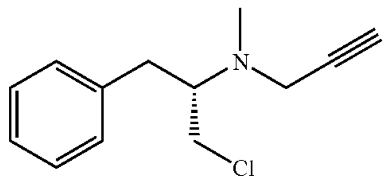
N-[(2S)-1-chloro-3-phenylpropan-2-yl]-N-methylprop-2-yn-1-amine
