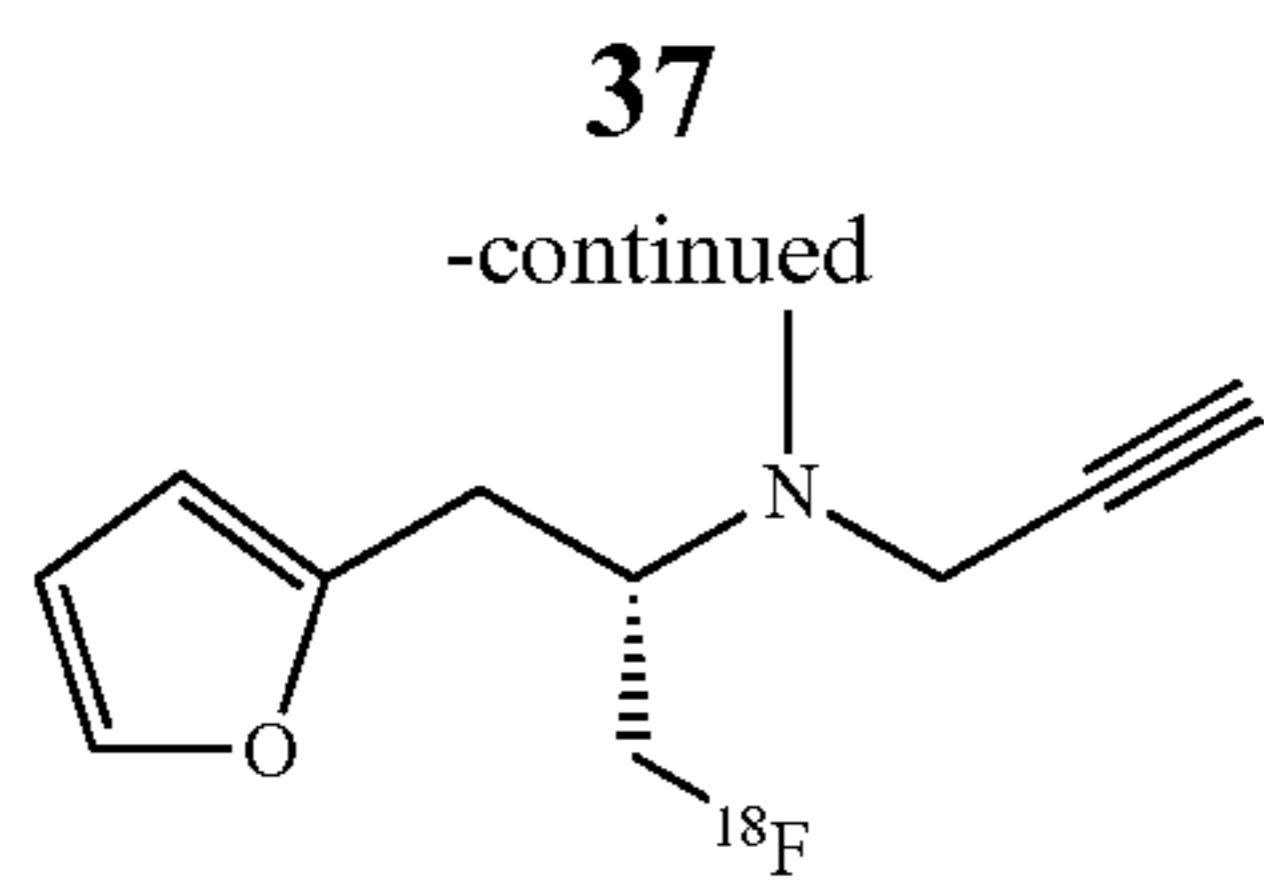
N-[(2S)-1-( 18 F)fluoro-3-(furan-2-yl)propan-2-yl]-N-methylprop-2-yn-1-amine
