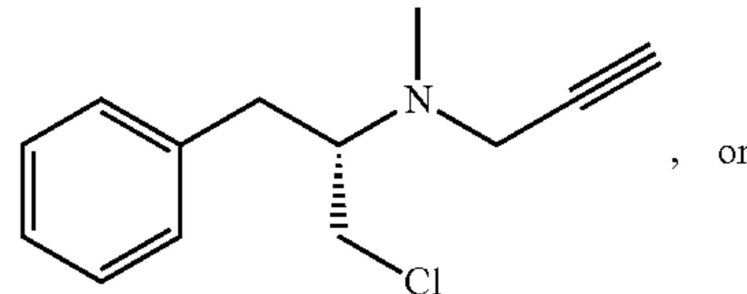
N-[(2S)-1-chloro-3-phenylpropan-2-yl]-N-methylprop-2-yn-1-amine
