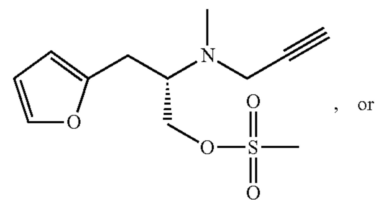
(2S)-3-(furan-2-yl)-2-[methyl(prop-2-yn-1-yl)amino]propyl methanesulfonate
