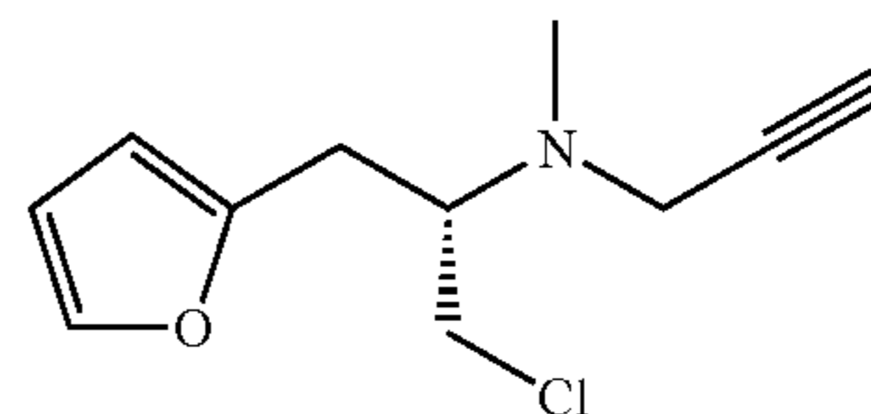
N-[(2S)-1-chloro-3-(furan-2-yl)propan-2-yl]-N-methylprop-2-yn-1-amine
