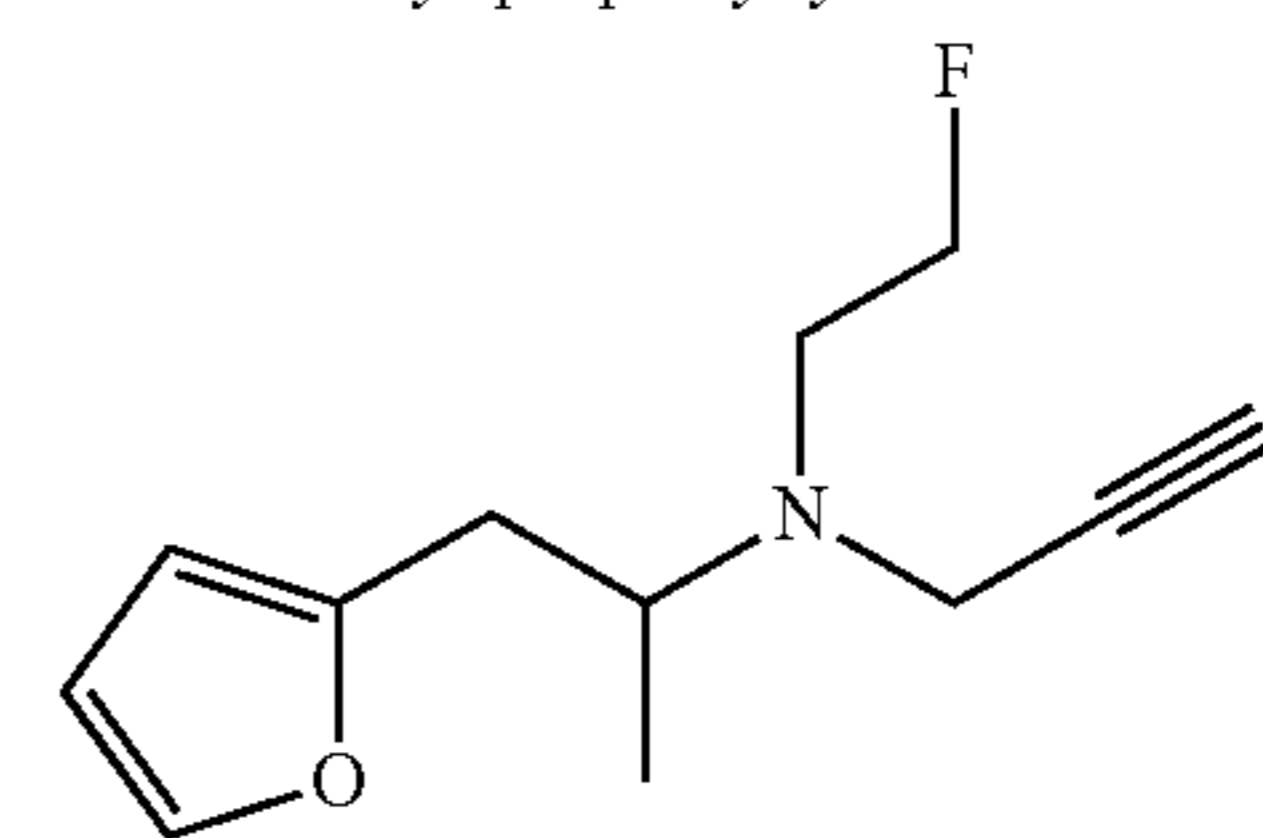
(2-Fluoro-ethyl)-(2-furan-2-yl-1-methyl-ethyl)-prop-2-ynyl-amine
