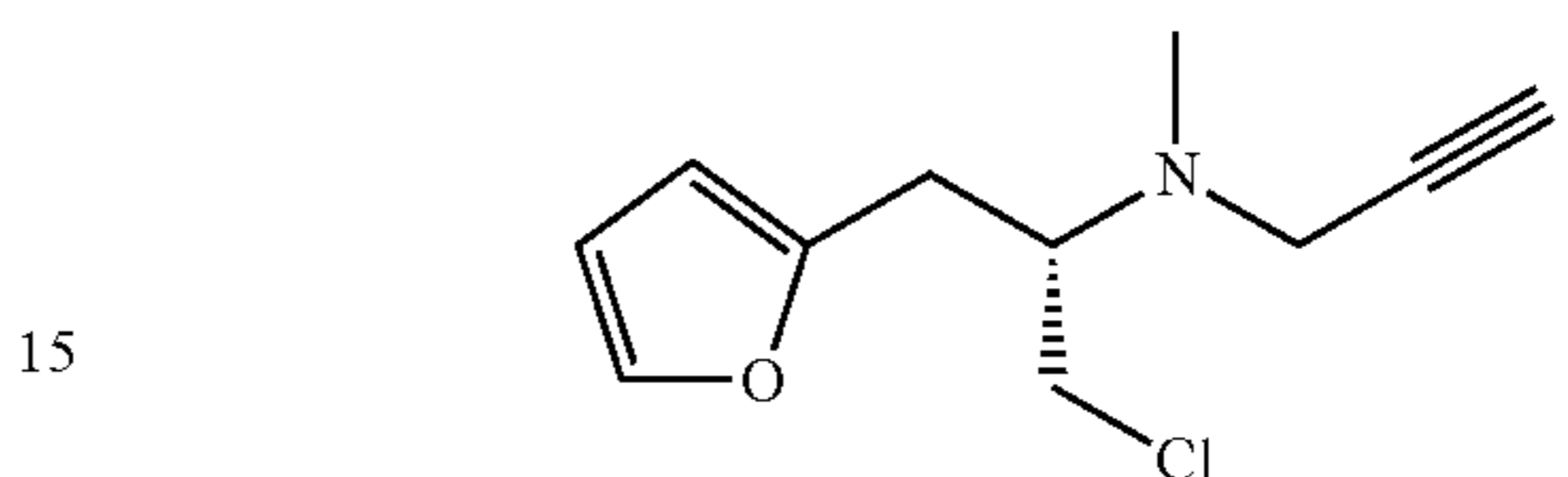
N-[(2S)-1-chloro-3-(furan-2-yl)propan-2-yl]-N-methylprop-2-yn-1-amine
