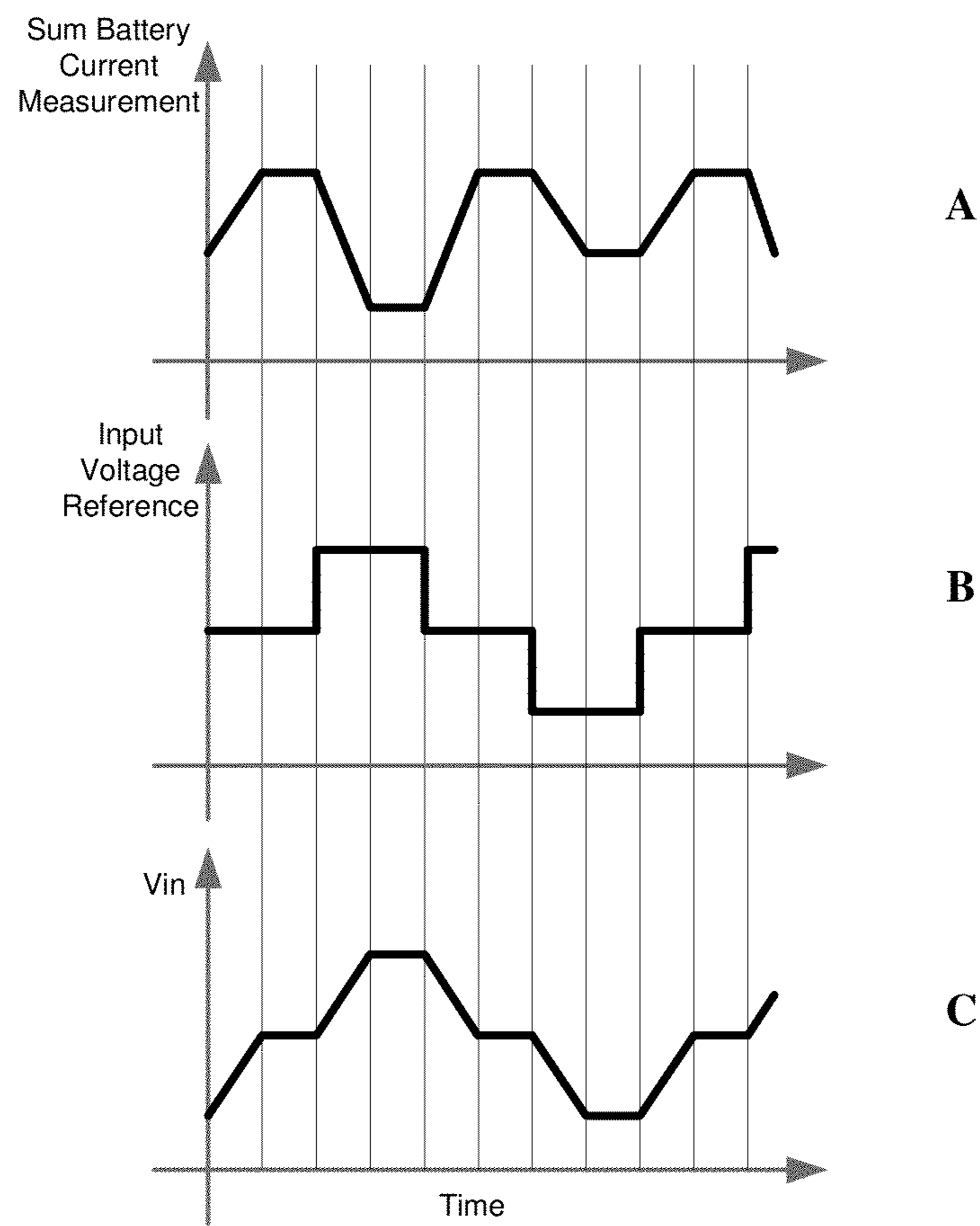
MPPT Mode
