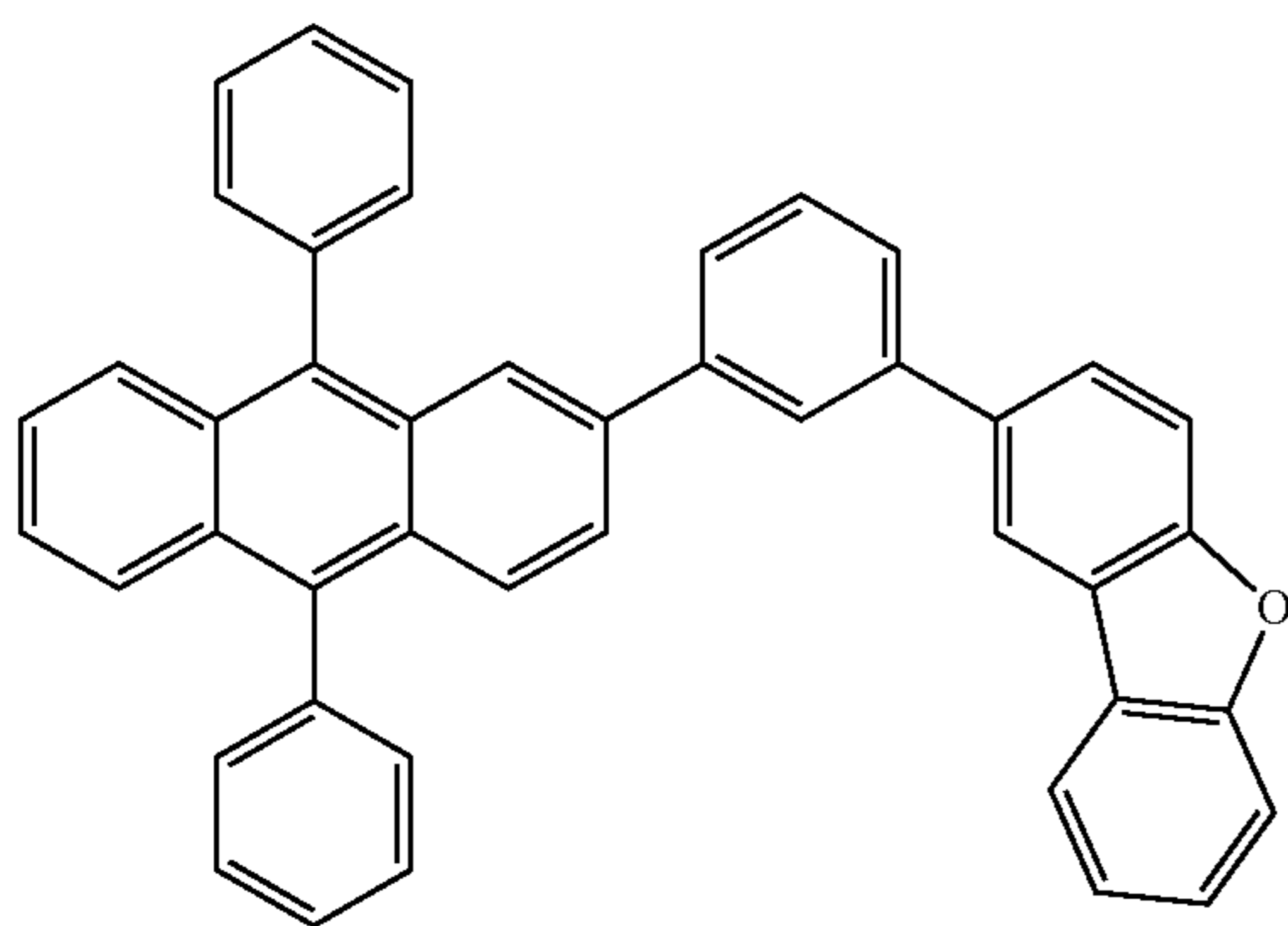
2mDBFPPA
