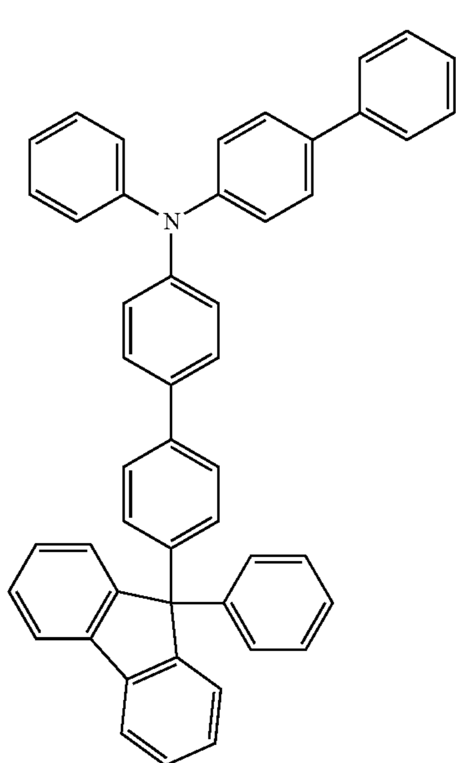
BPAFLBi
