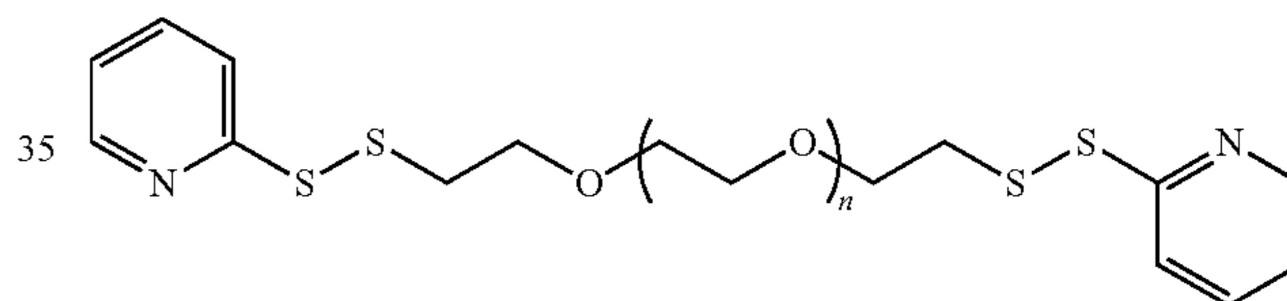
PEG 2000 -Di-((CH 2 ) 2 -Orthopyridyl Disulfide)
