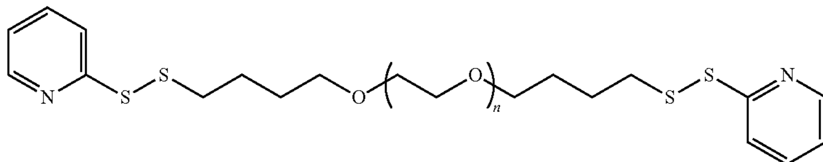
PEG 2000 -Di-((CH 2 ) 4 -Orthopyridyl Disulfide)
