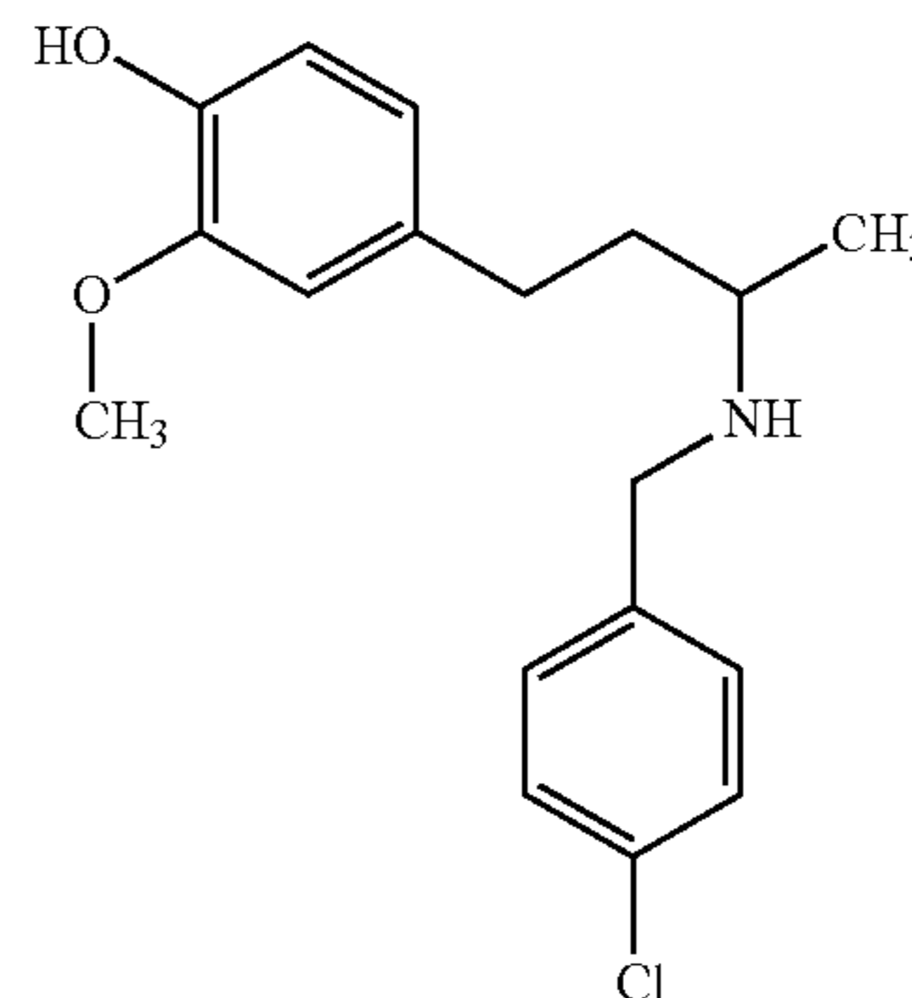
4-(3-(4-chlorobenzylamino)butyl)-2-methoxyphenol
