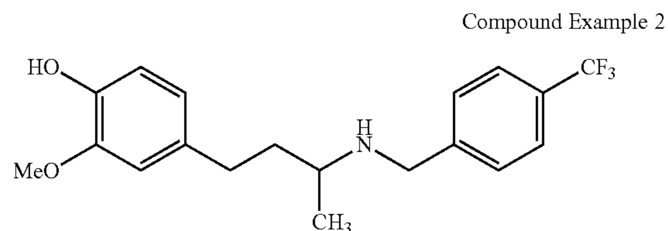
4-(3-(4-(trifluoromethyl)benzylamino)butyl)-2-methoxyphenol
