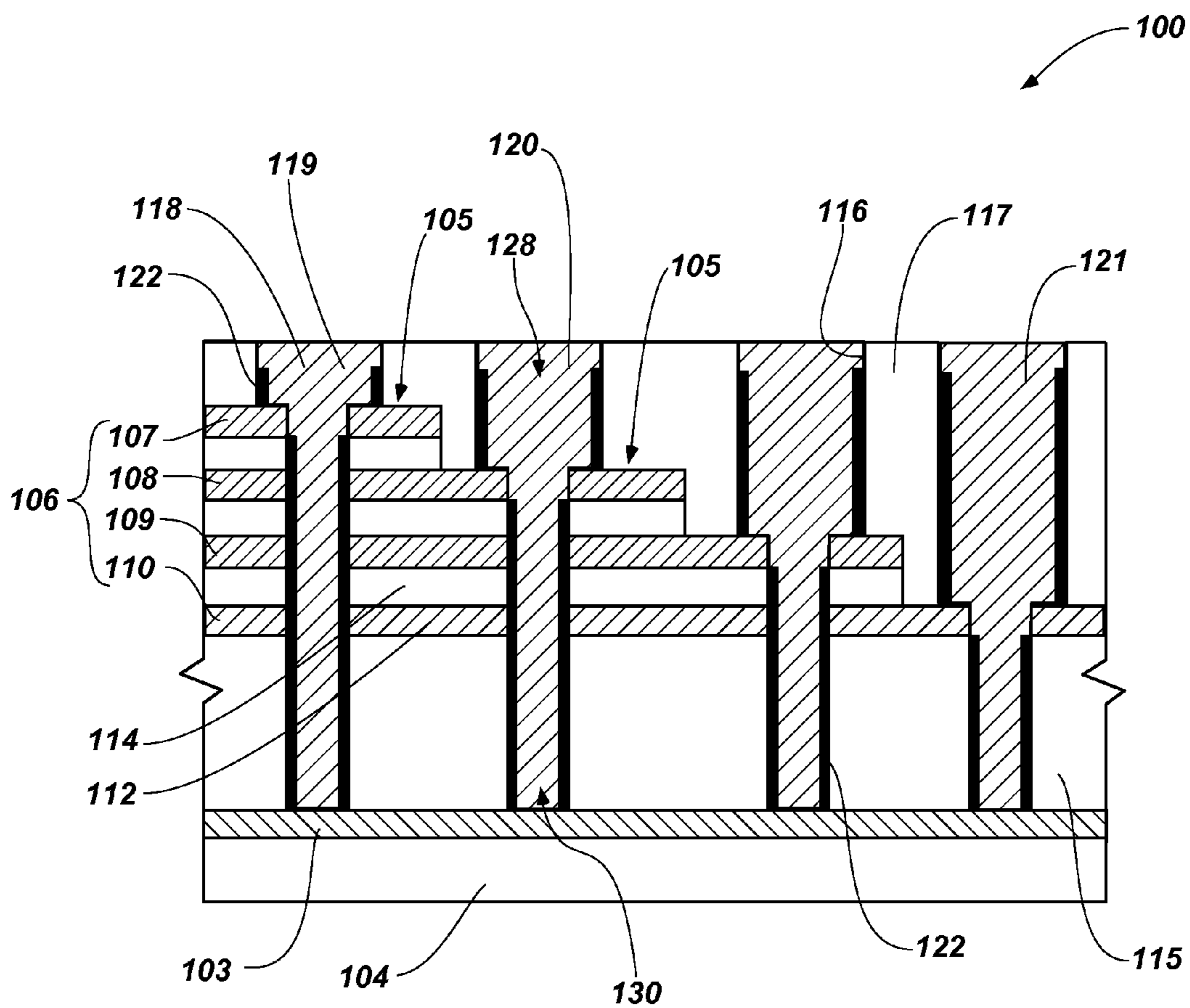
FIG. 2
