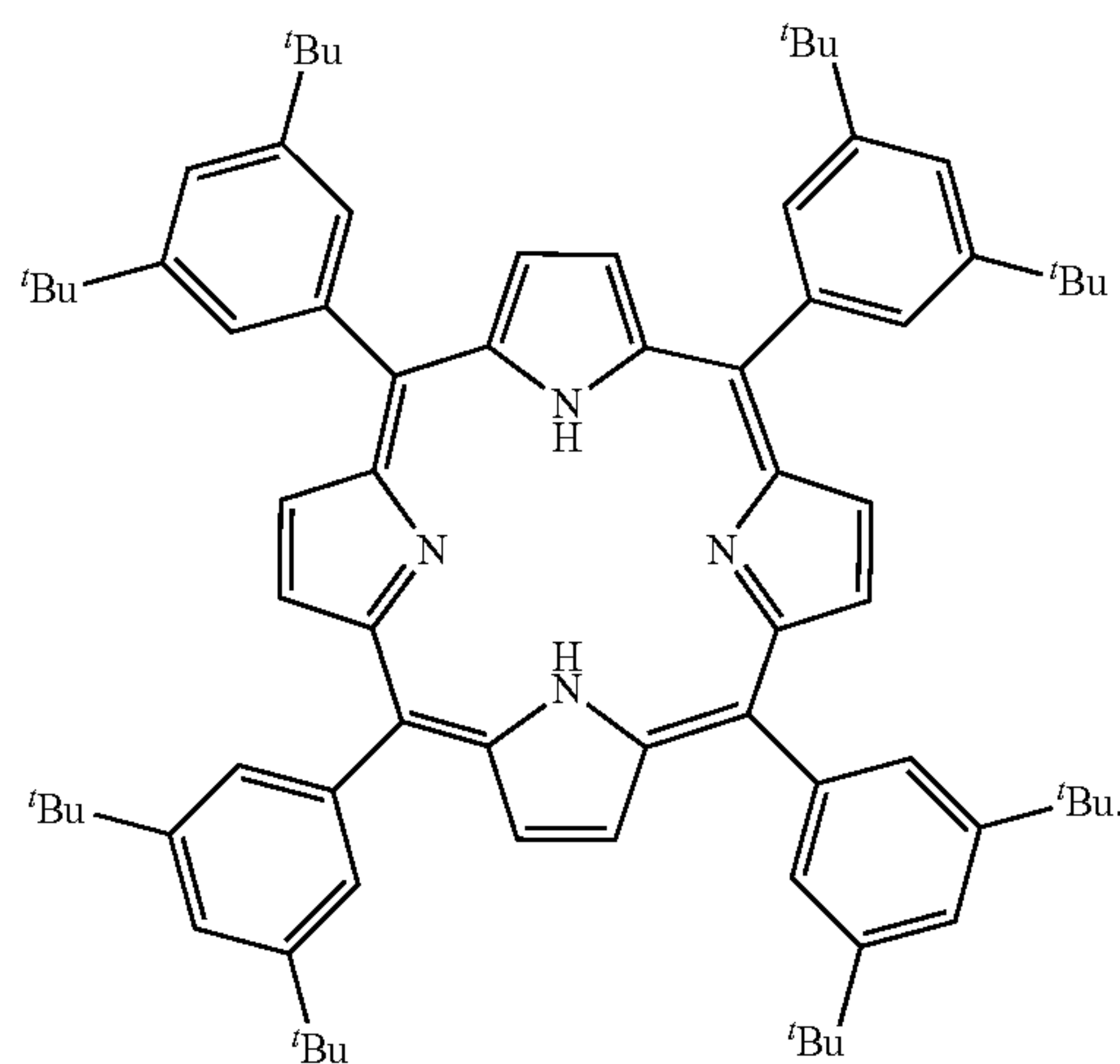
(DTBP)
