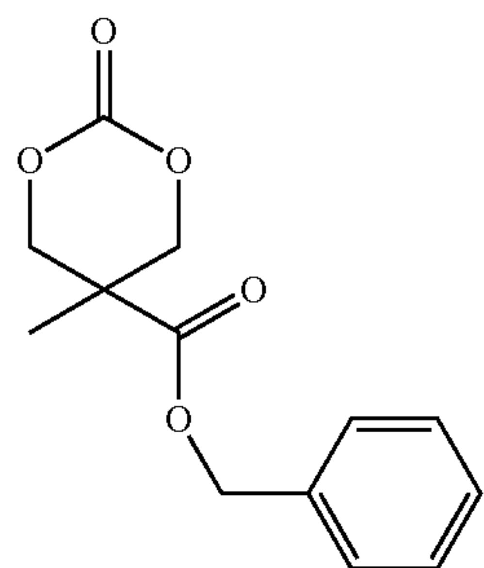
(MTCOBn)
