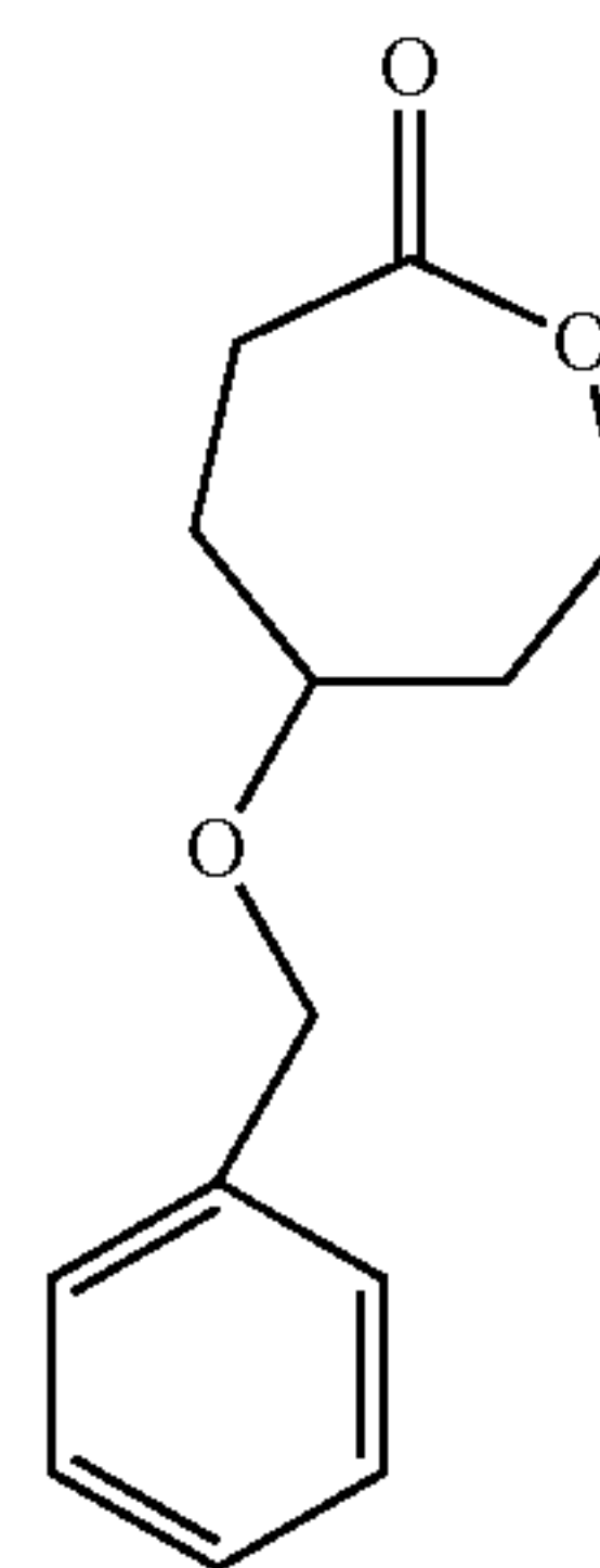
5-(Benzyloxy)oxepan-2-one (BXO)
