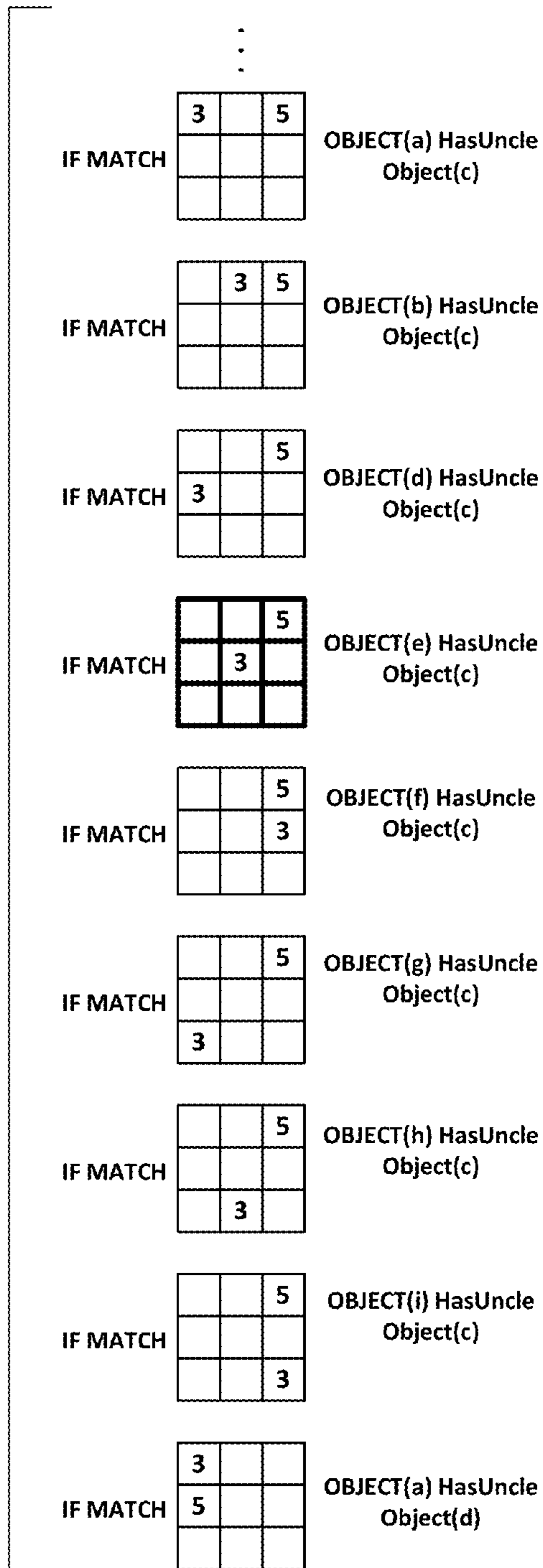
FIG. 26 – PREDICATE TEMPLATES
