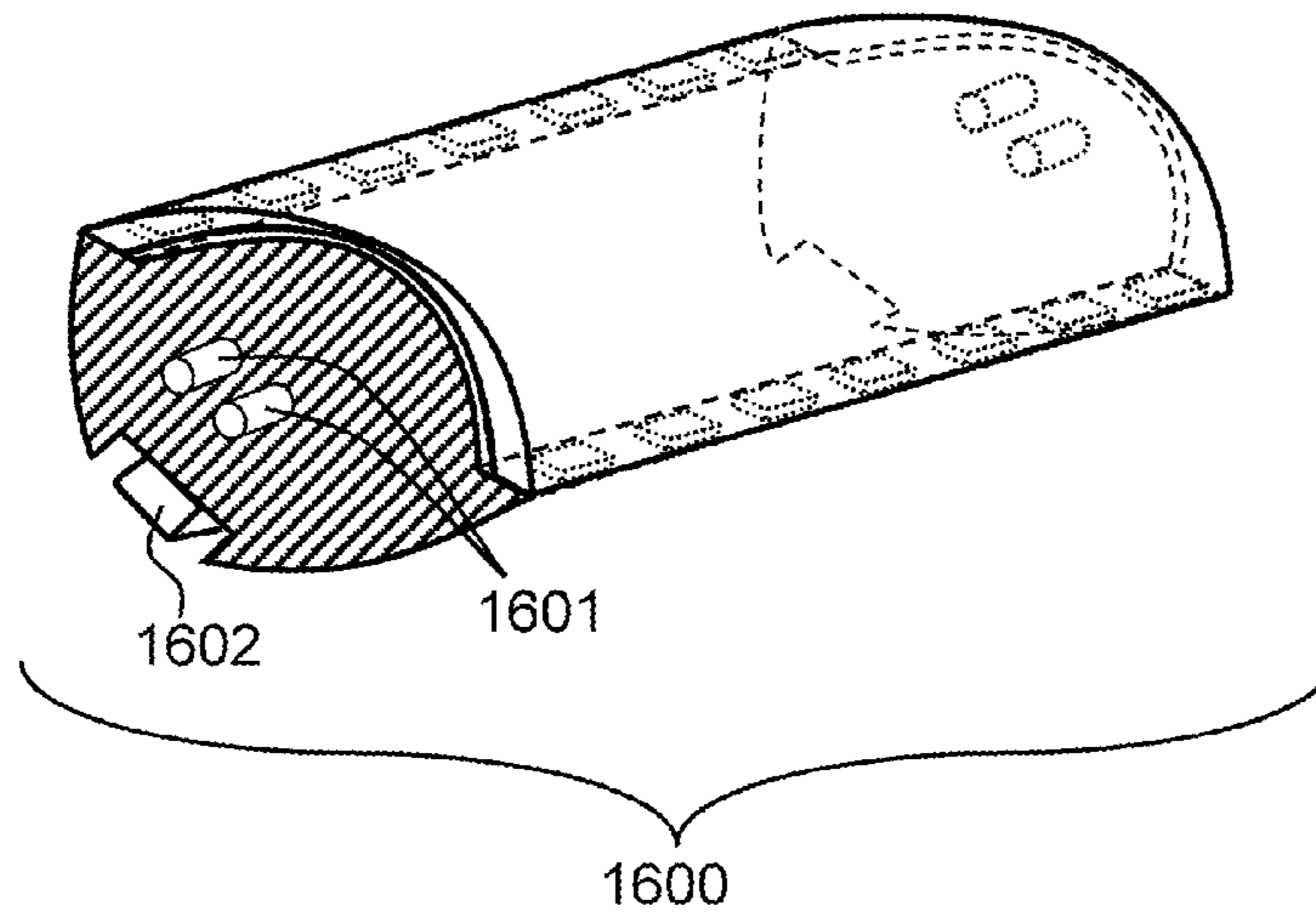
FIG. 16
