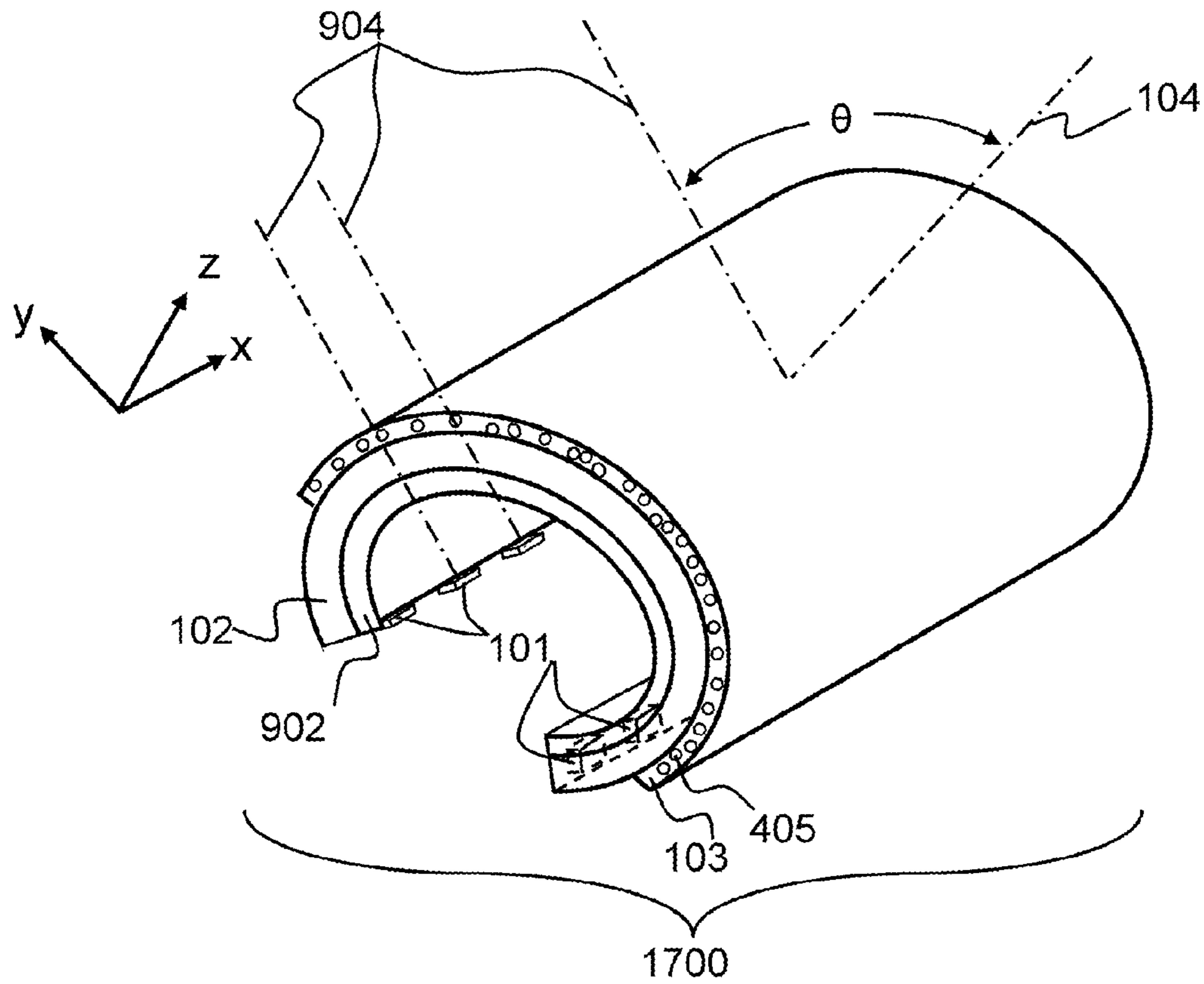
FIG. 17
