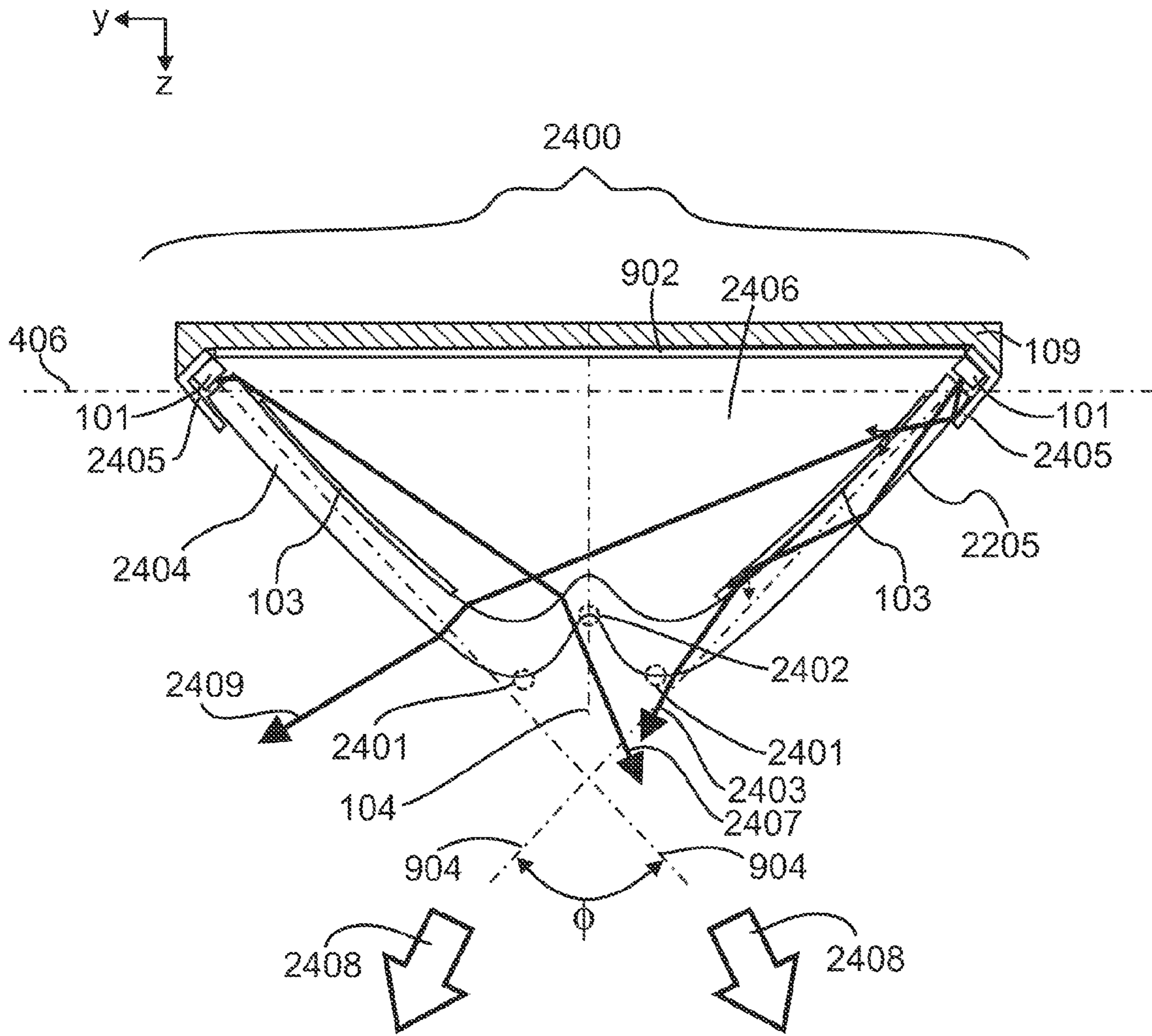
FIG. 24
