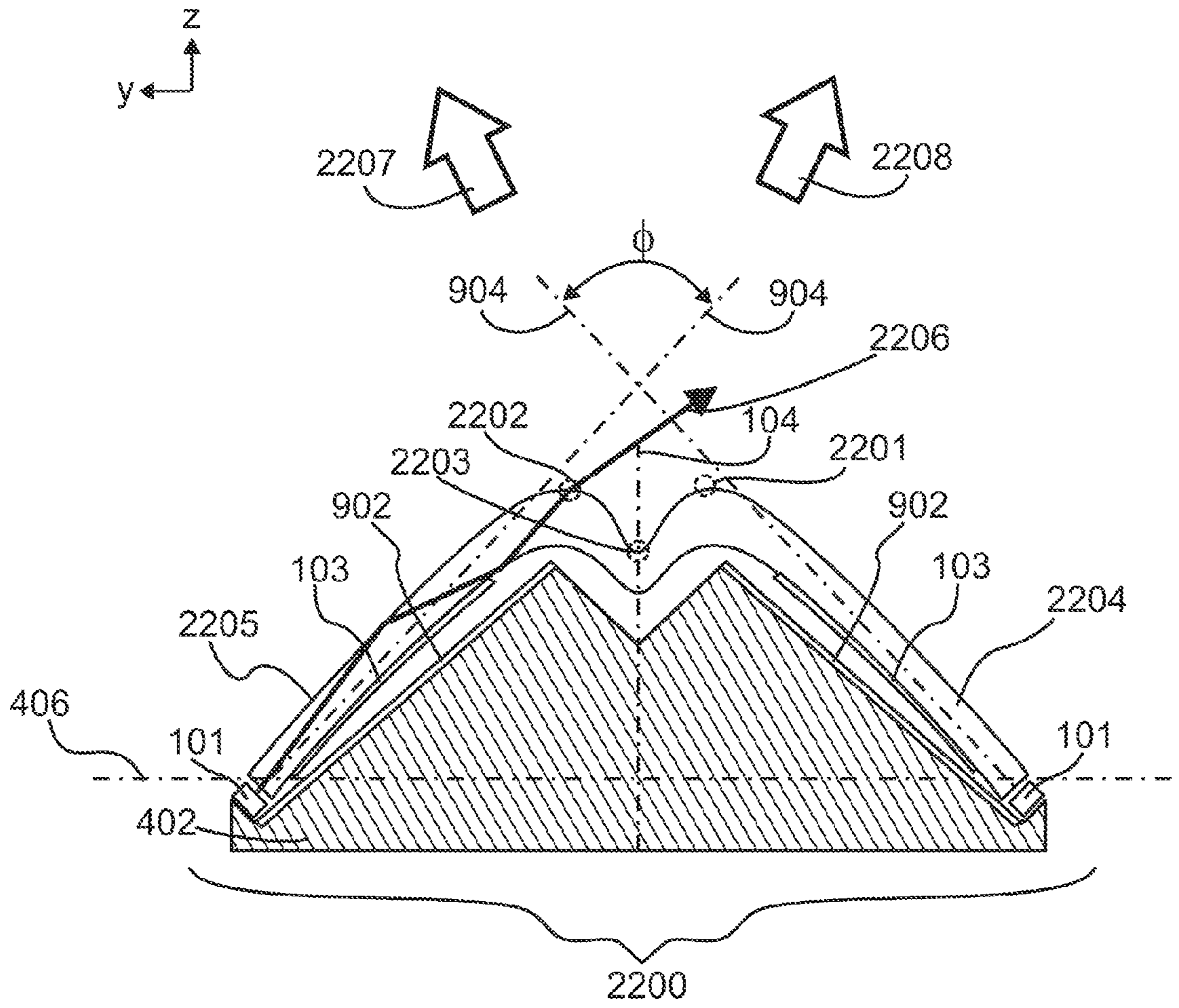
FIG. 22
