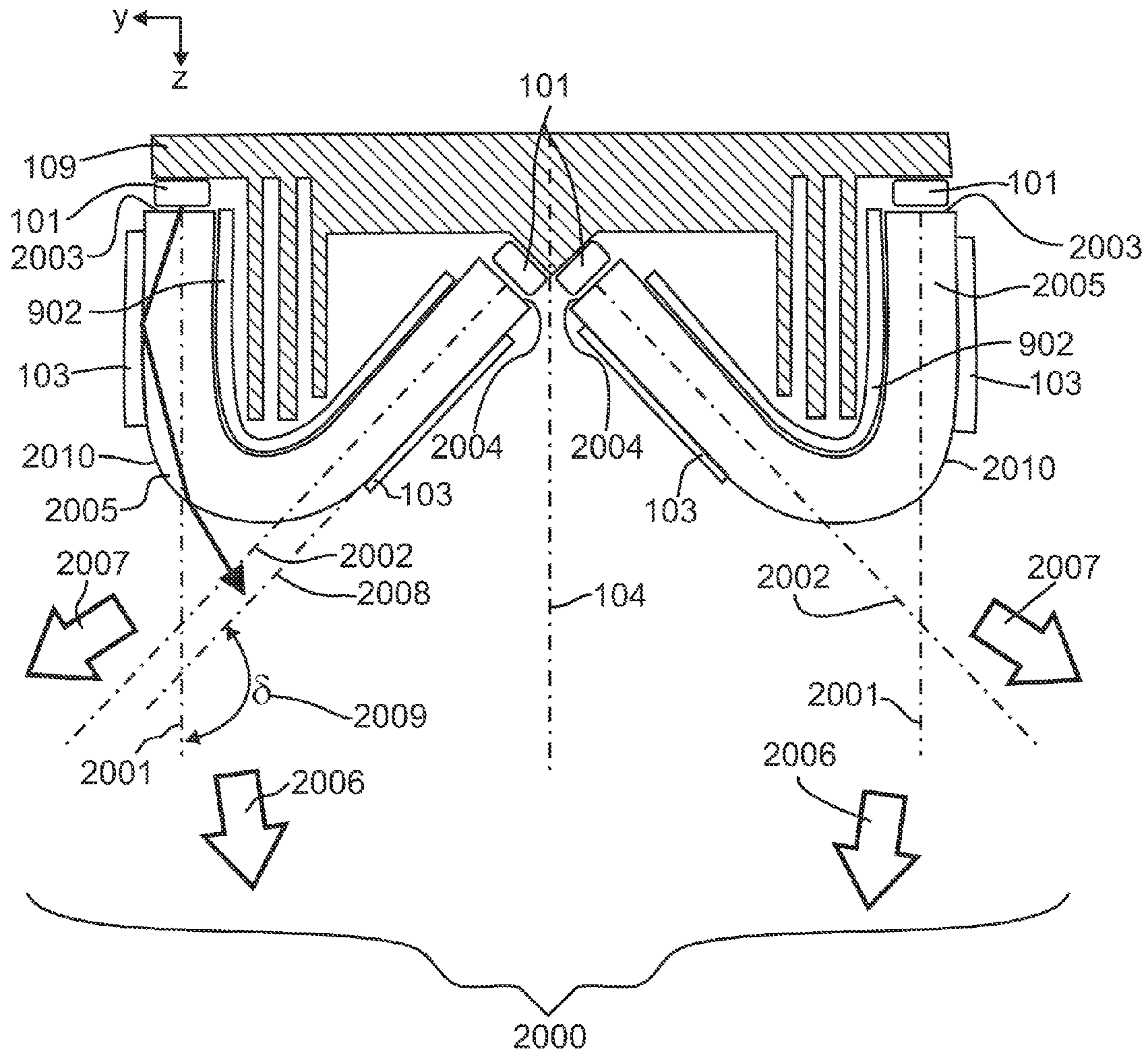
FIG. 20a
