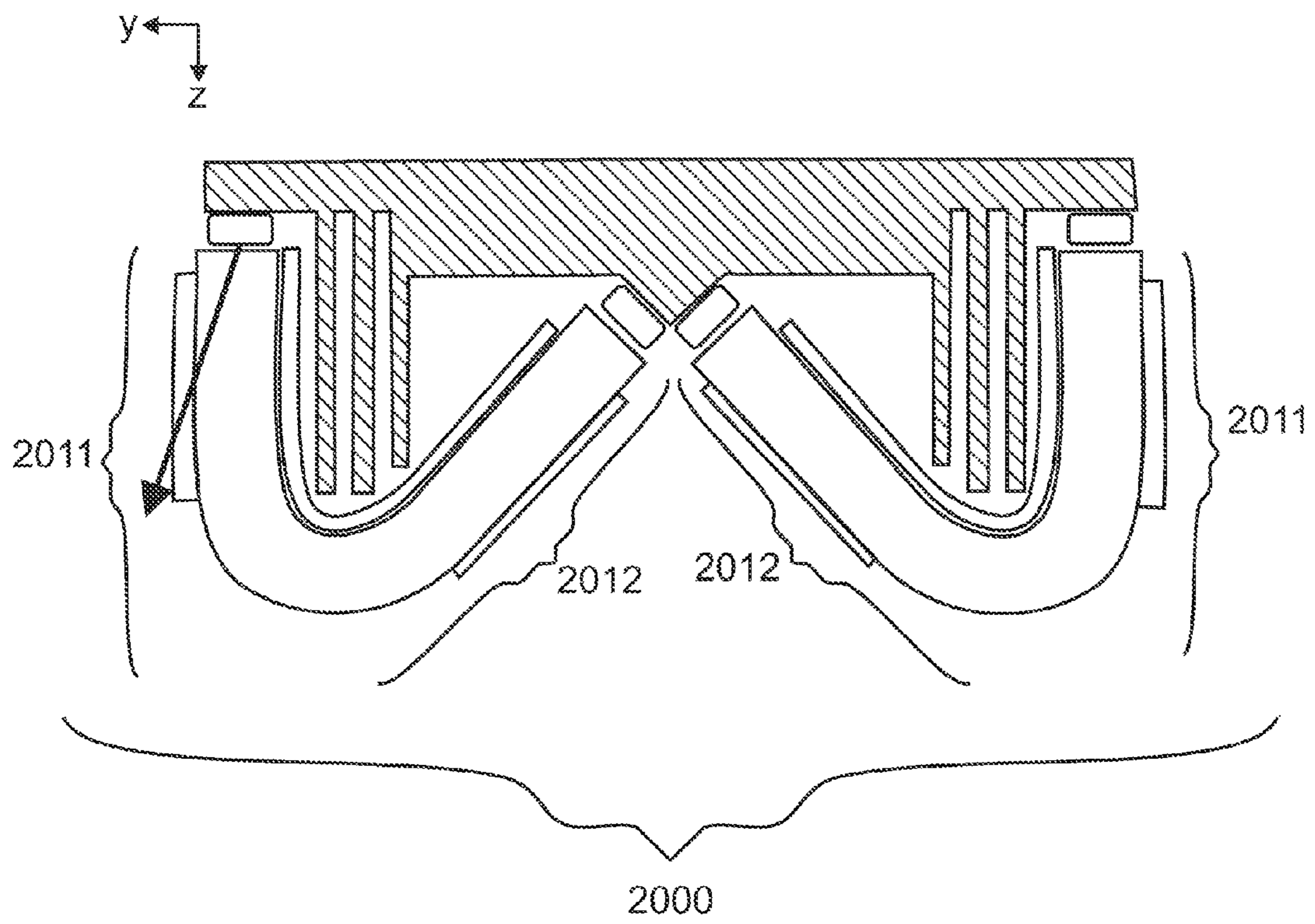
FIG. 20b
