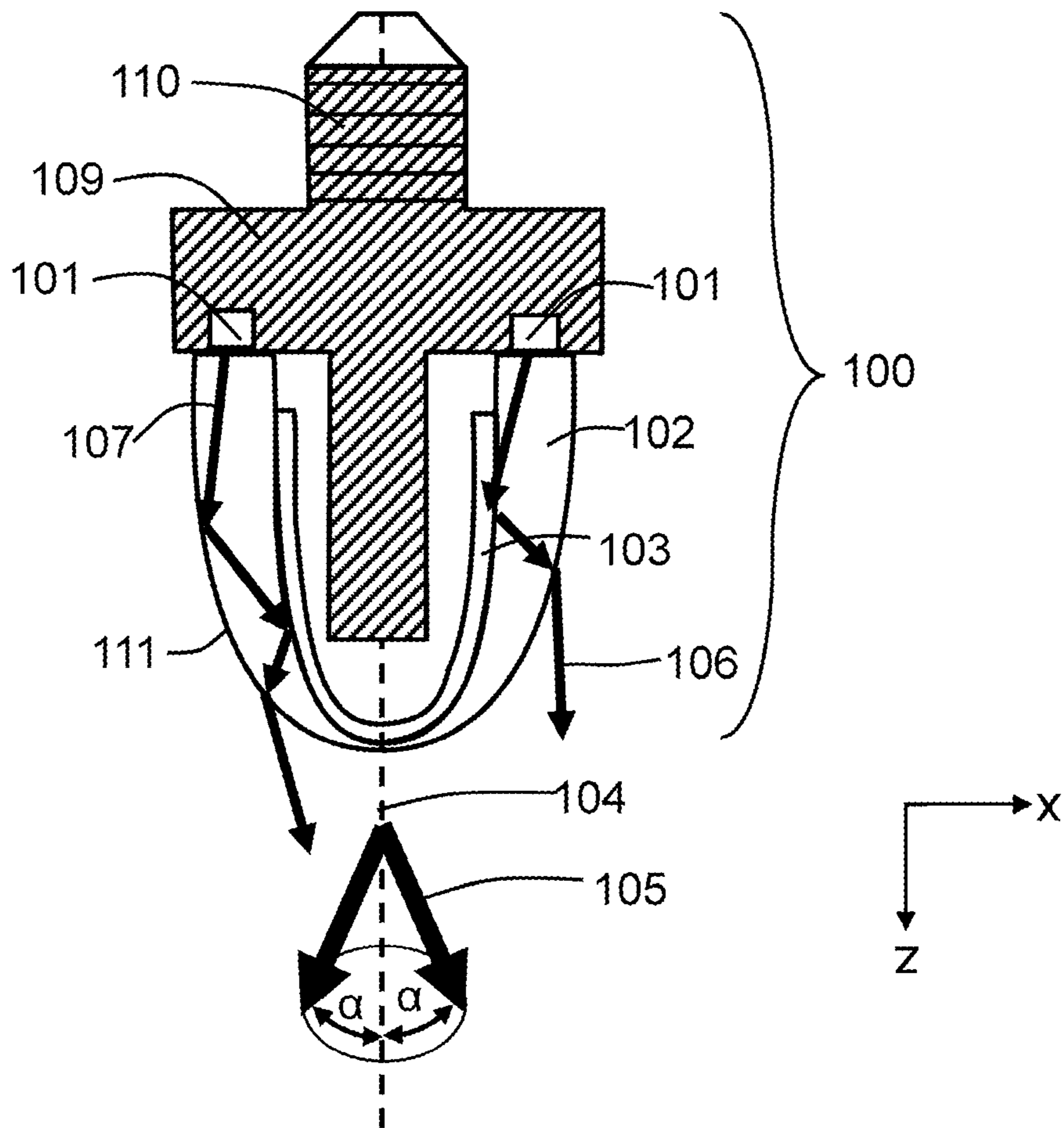
FIG. 1
