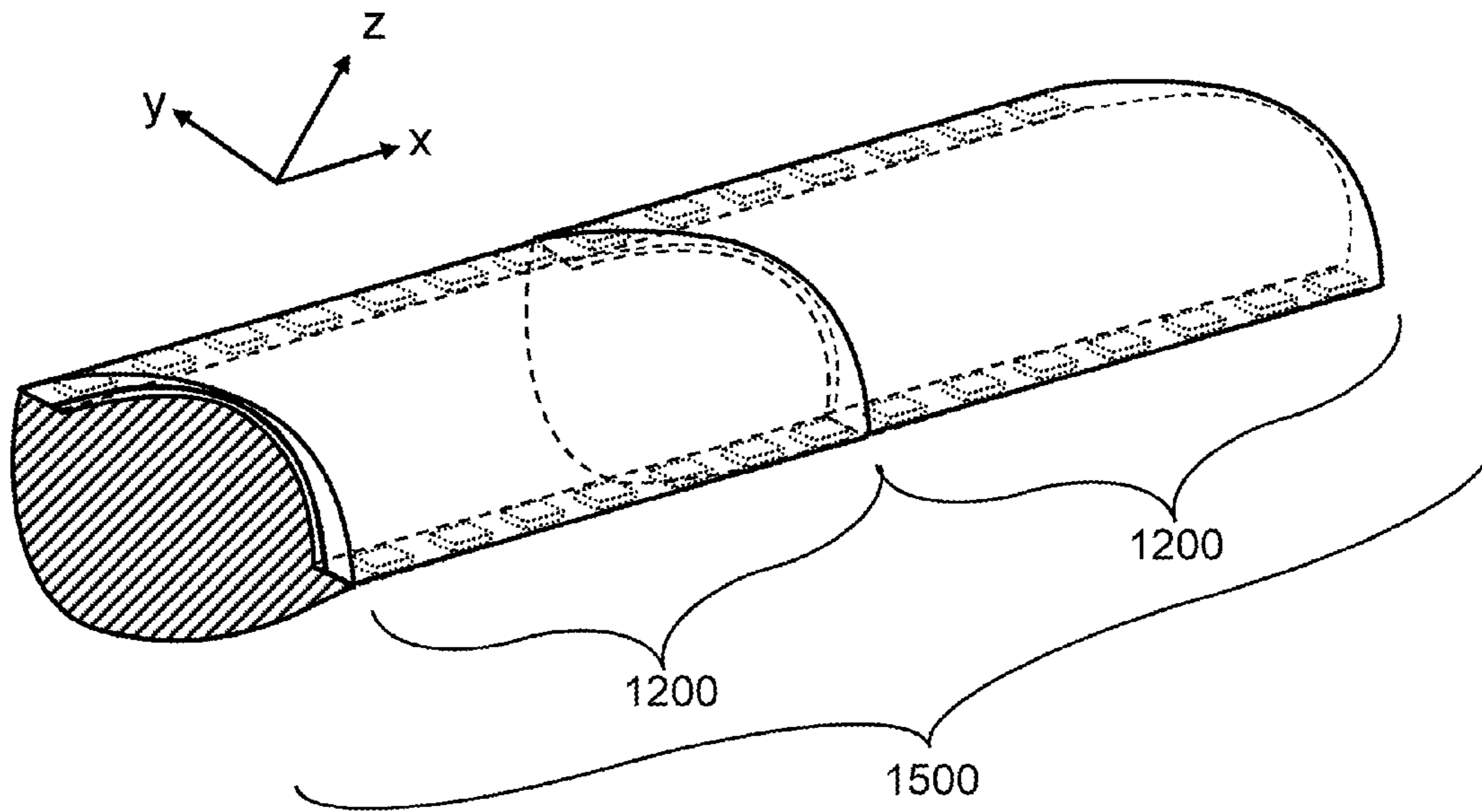
FIG. 15
