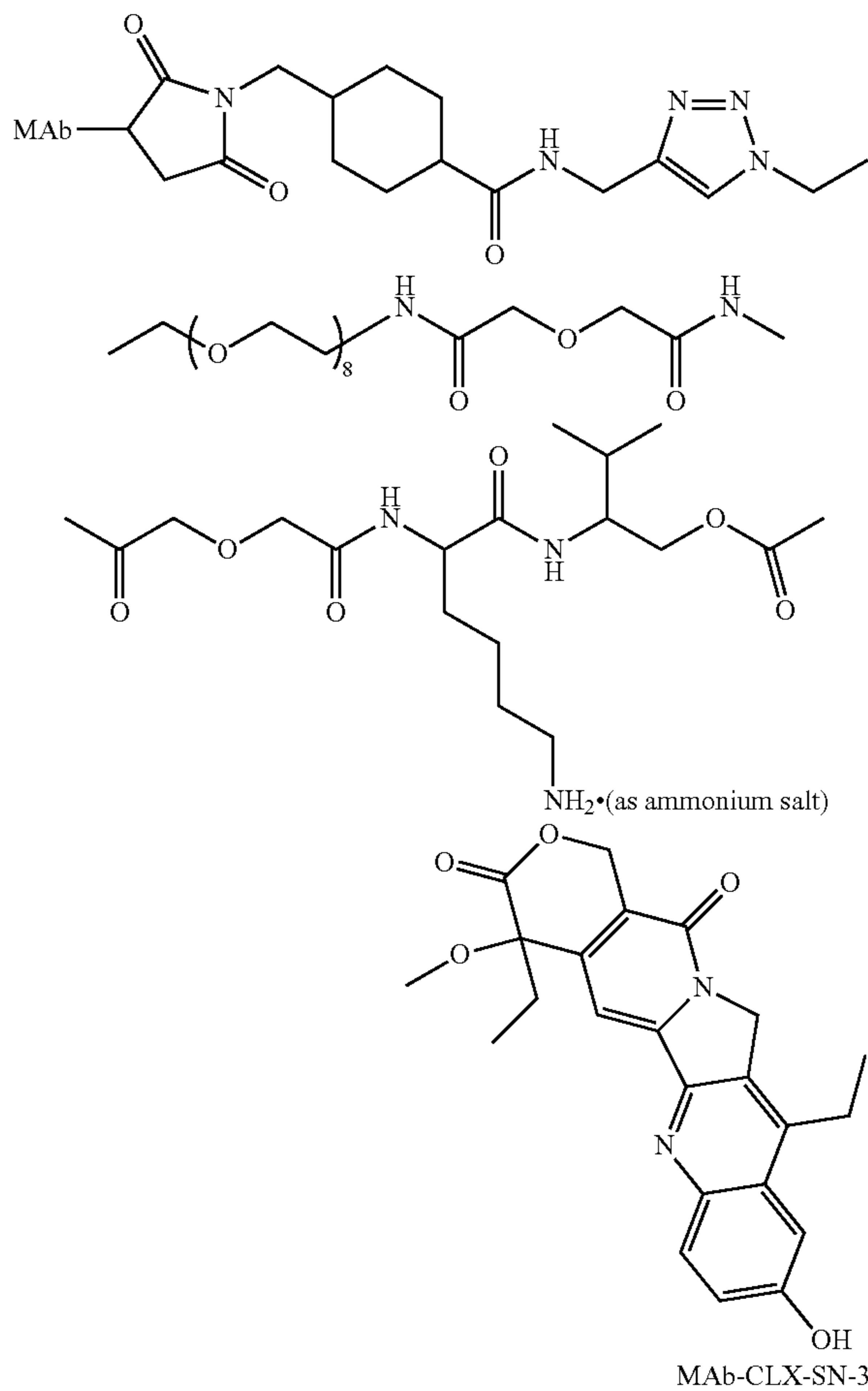
MAb-CL7-SN-38
