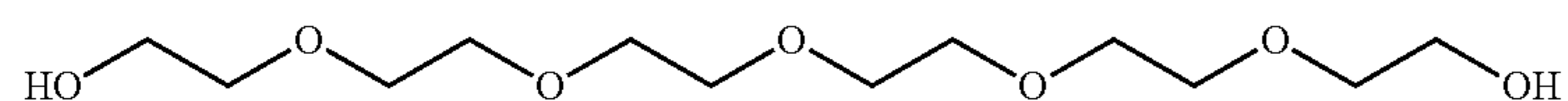
Hexaethylene glycol
