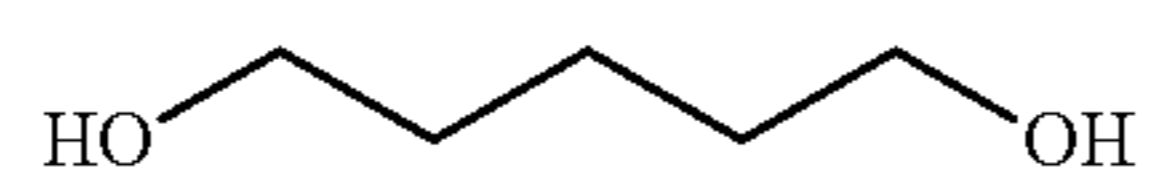
1,5-Pentanediol
