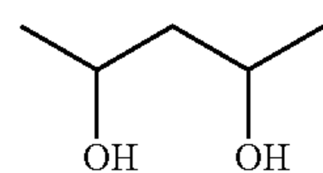
2,4-Pentanediol
