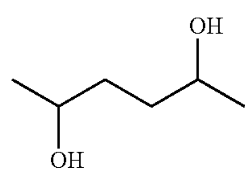
2,5-Hexanediol
