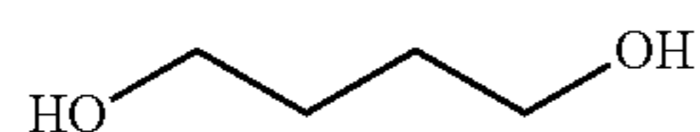
1,4-Butanediol
