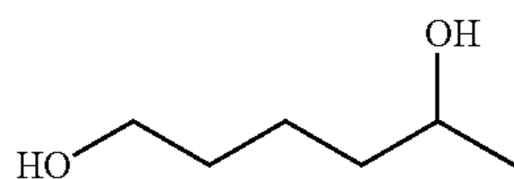
1,5-Hexanediol
