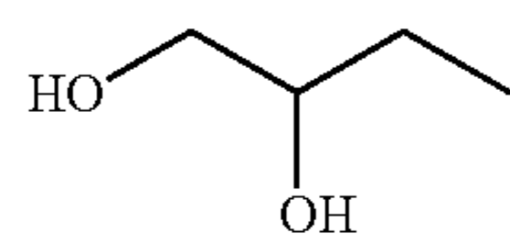
1,4-Butanediol
