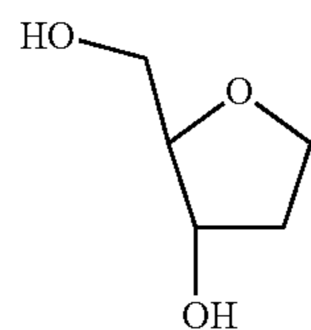
1,2-Dideoxyribose
