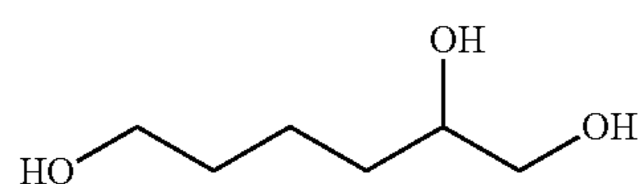
1,2,6-Hexanetriol
