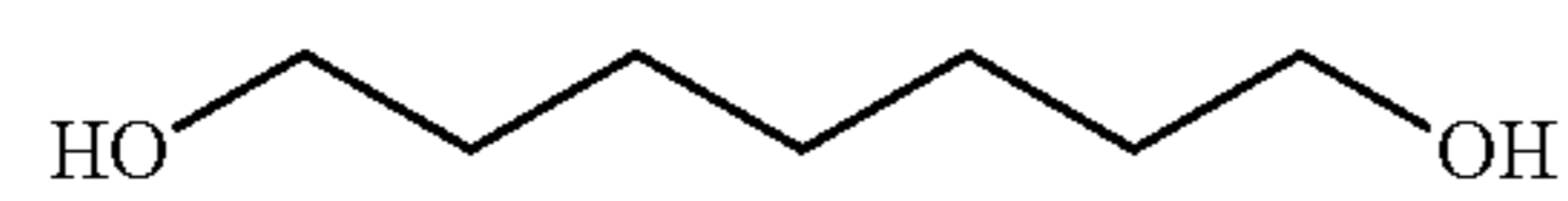
1,7-Heptanediol
