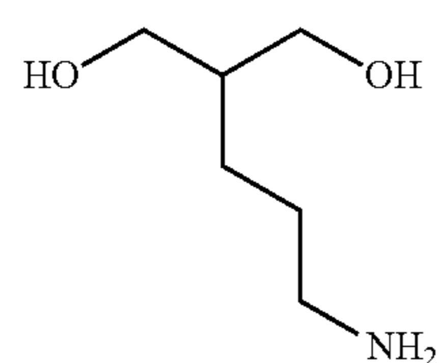
2-(1-Aminopropyl)- 1,3-propanediol
