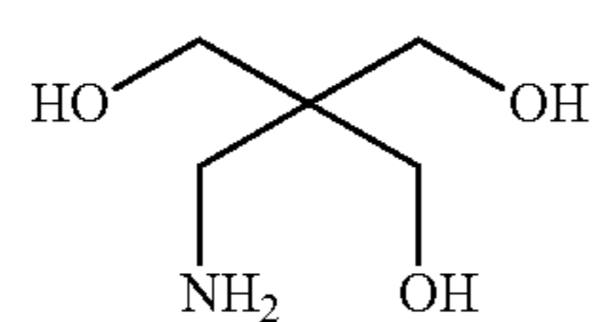
2-Amino-2-(hydroxymethyl)- 1,3-propanediol
