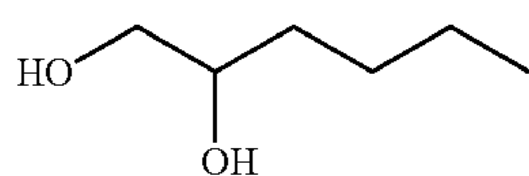
1,2-Hexanediol
